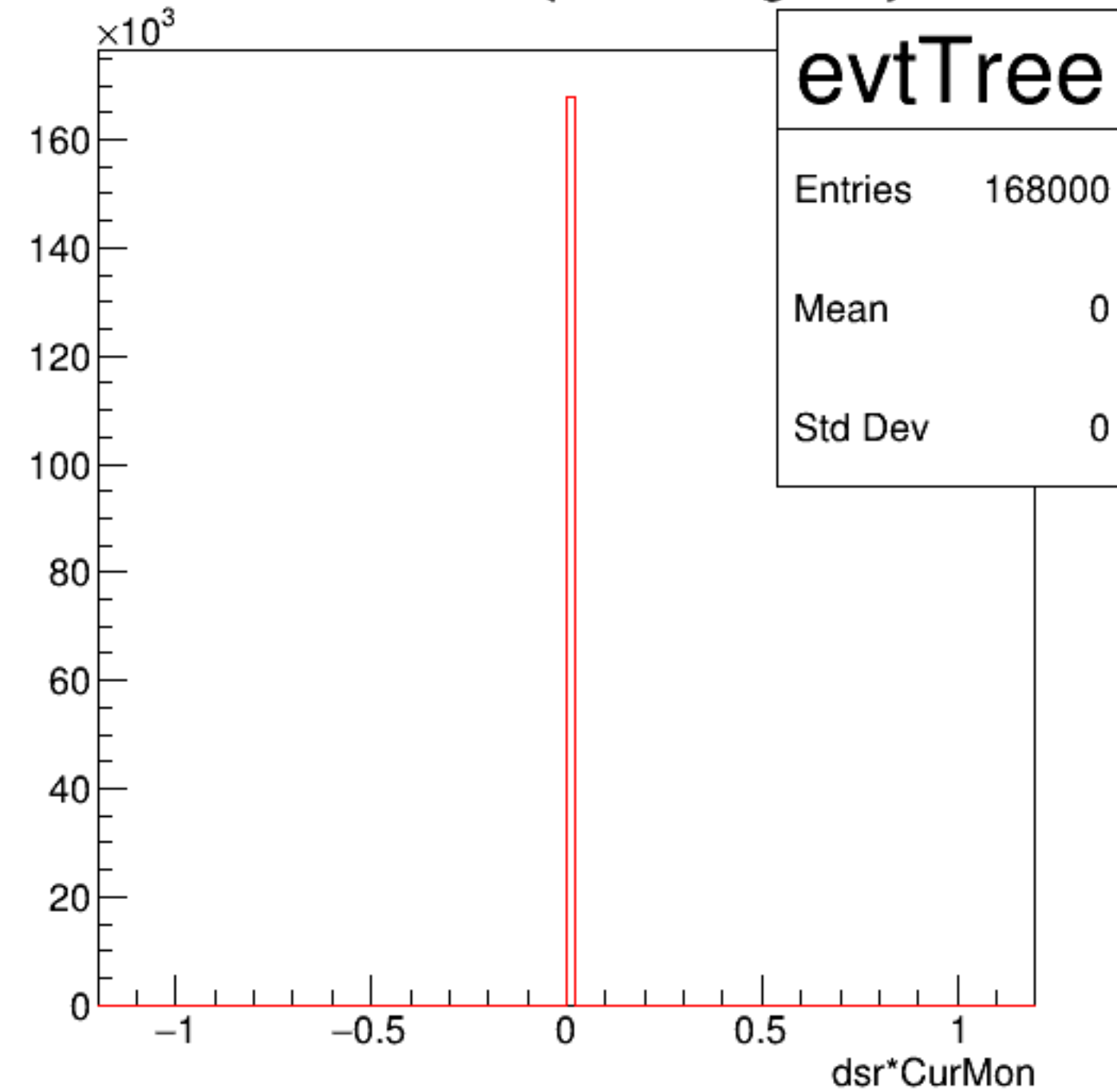
dsr*CurMon {ErrorFlag==0}
