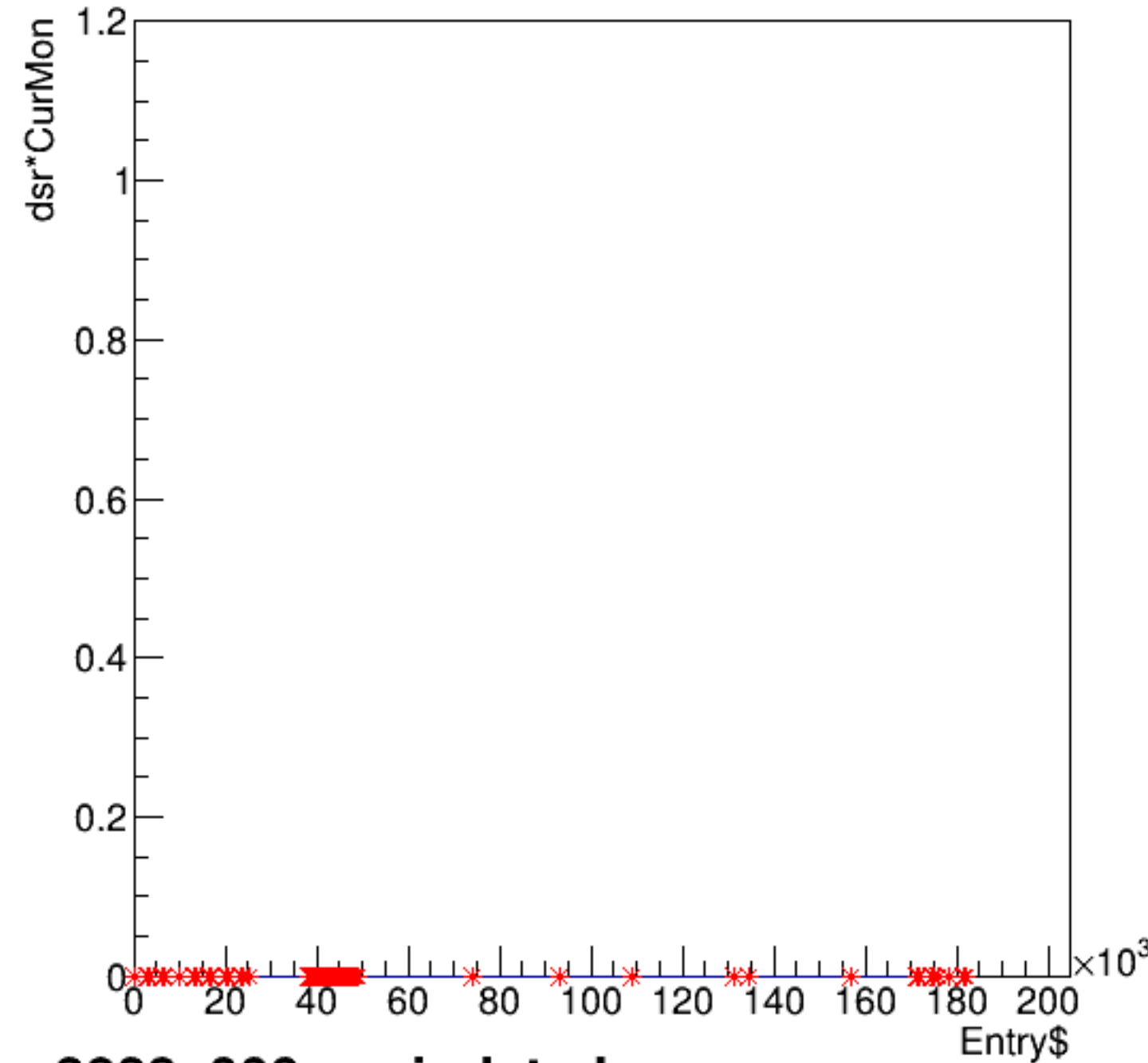
dsr*CurMon:Entry$
