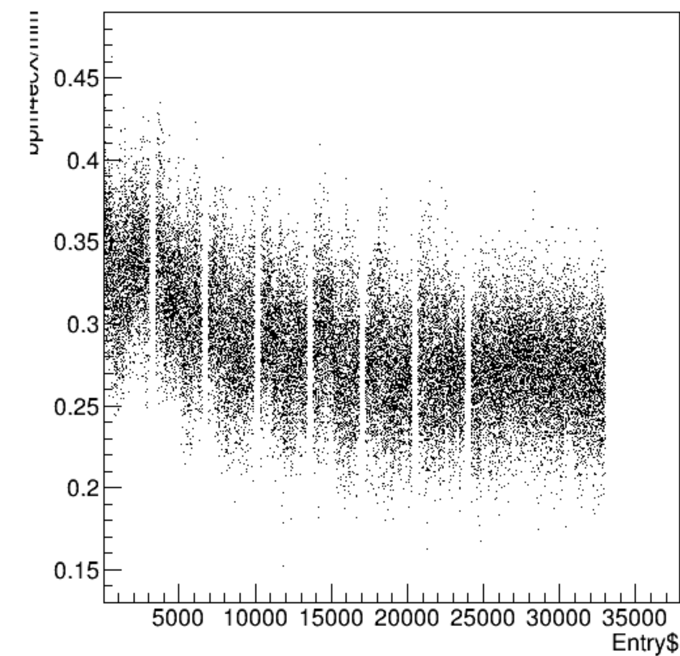
bpm4ecX/mm:Entry$ {ErrorFlag==0}
