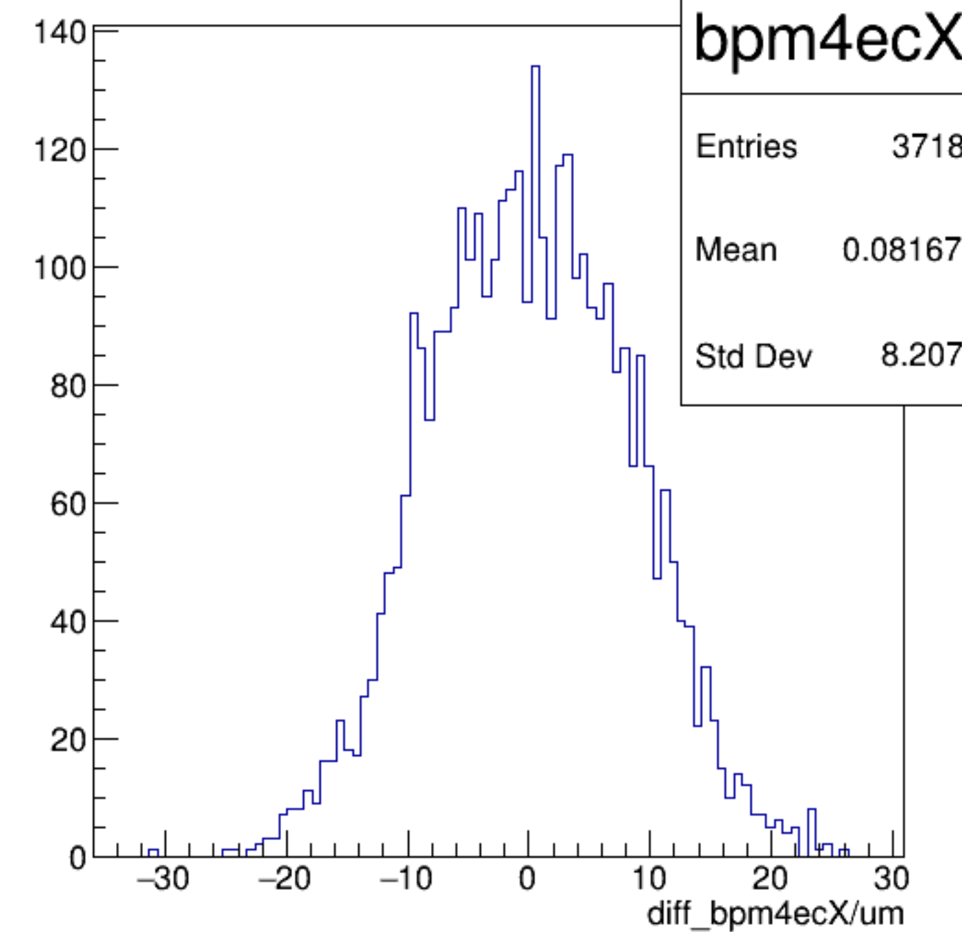
diff_bpm4ecX/um {ErrorFlag==0}
