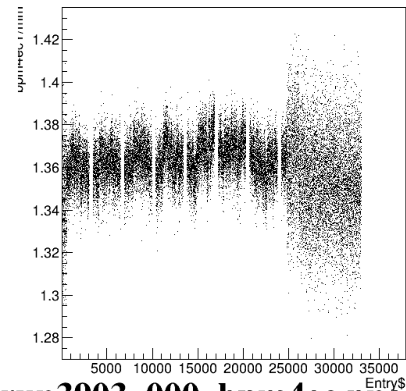
bpm4ecY/mm:Entry$ {ErrorFlag==0}
