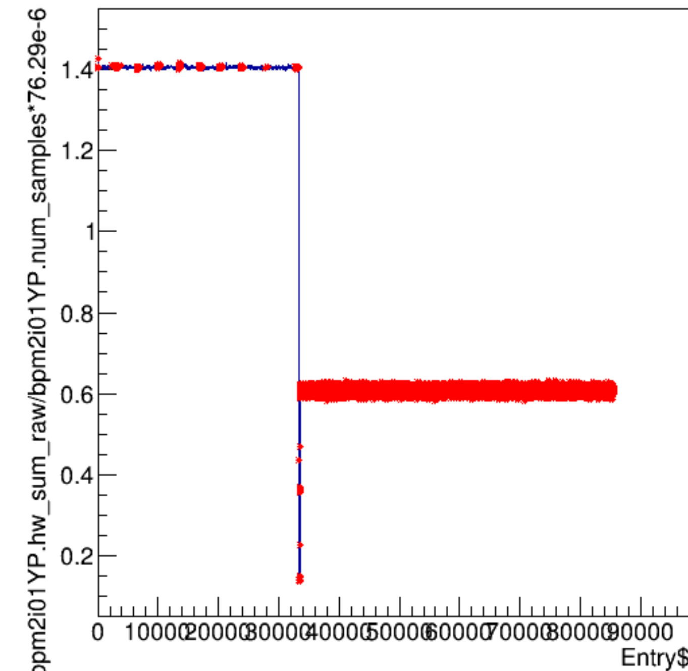
bpm2i01YP.hw_sum_raw/bpm2i01YP.num_samples*76.29e-6:Entry$
