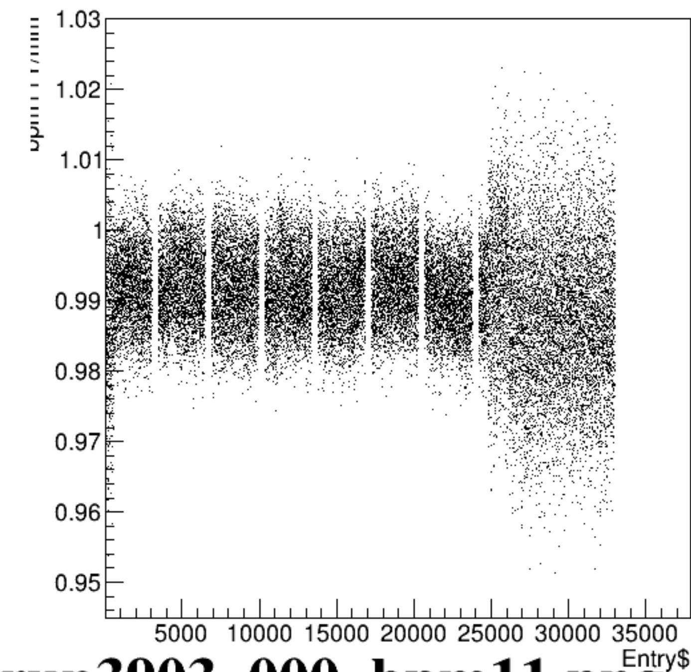
bpm11Y/mm:Entry$ {ErrorFlag==0}
