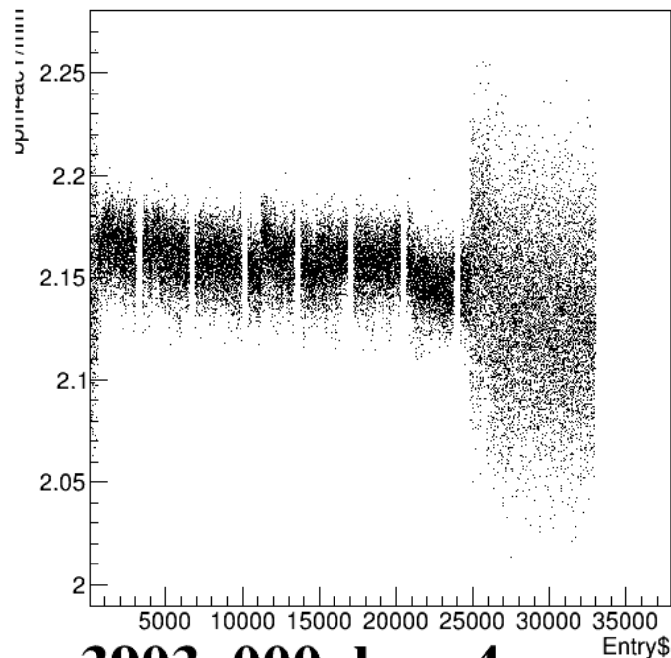
bpm4acY/mm:Entry$ {ErrorFlag==0}
