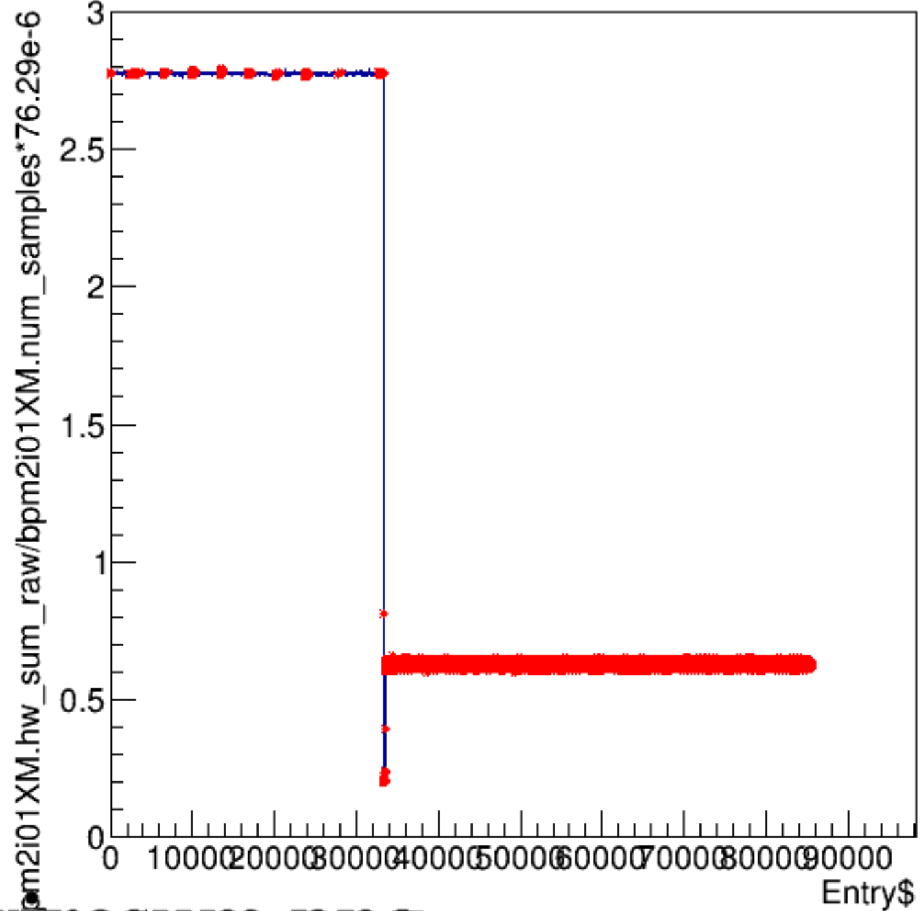
bpm2i01XM.hw_sum_raw/bpm2i01XM.num_samples*76.29e-6:Entry$
