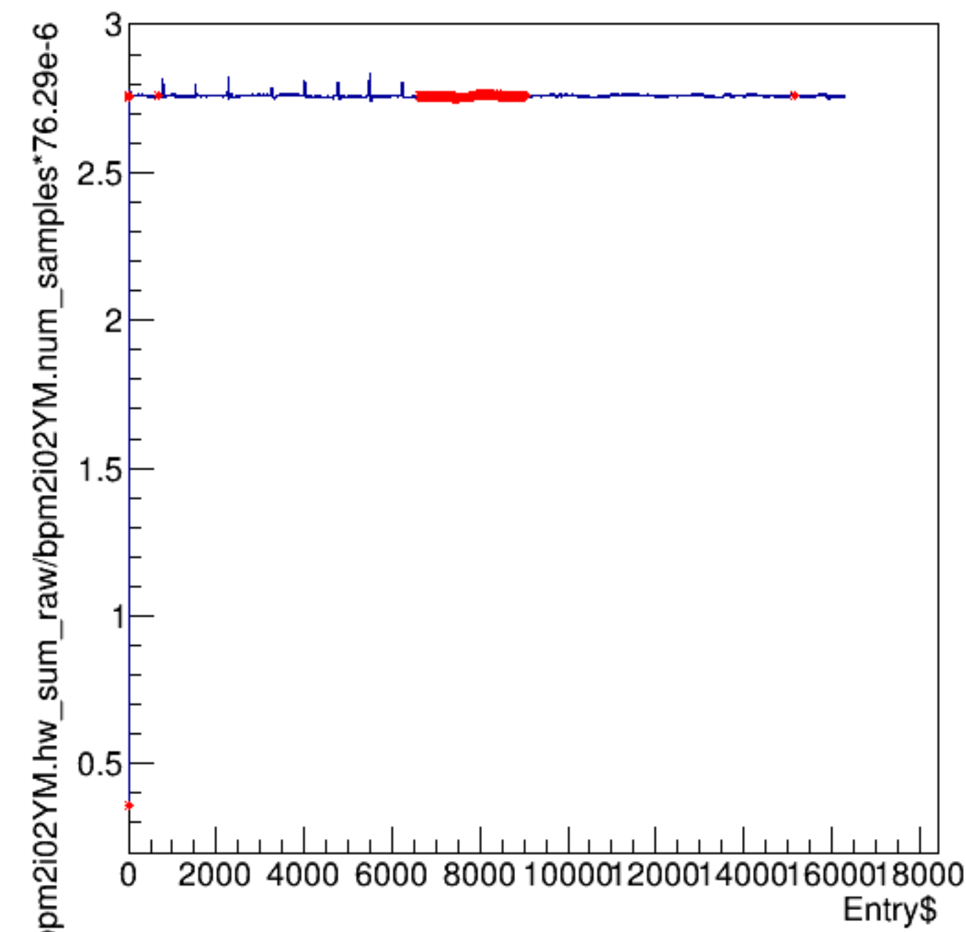
bpm2i02YM.hw_sum_raw/bpm2i02YM.num_samples*76.29e-6:Entry$
