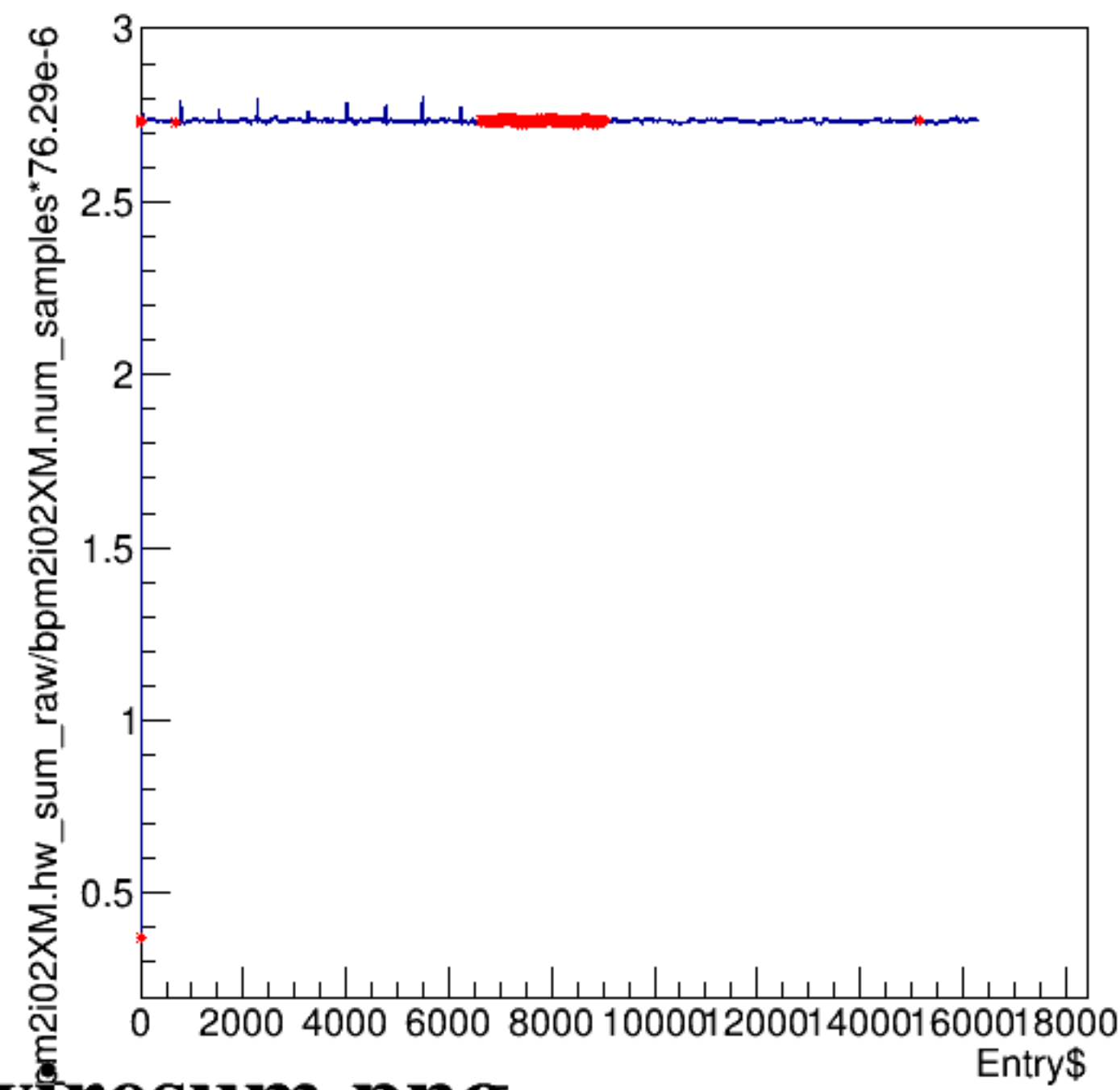
bpm2i02XM.hw_sum_raw/bpm2i02XM.num_samples*76.29e-6:Entry$
