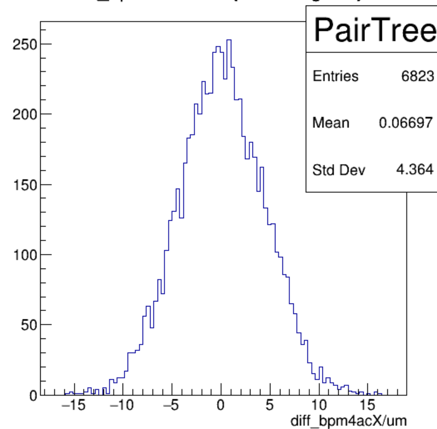
diff_bpm4acX/um {ErrorFlag==0}
