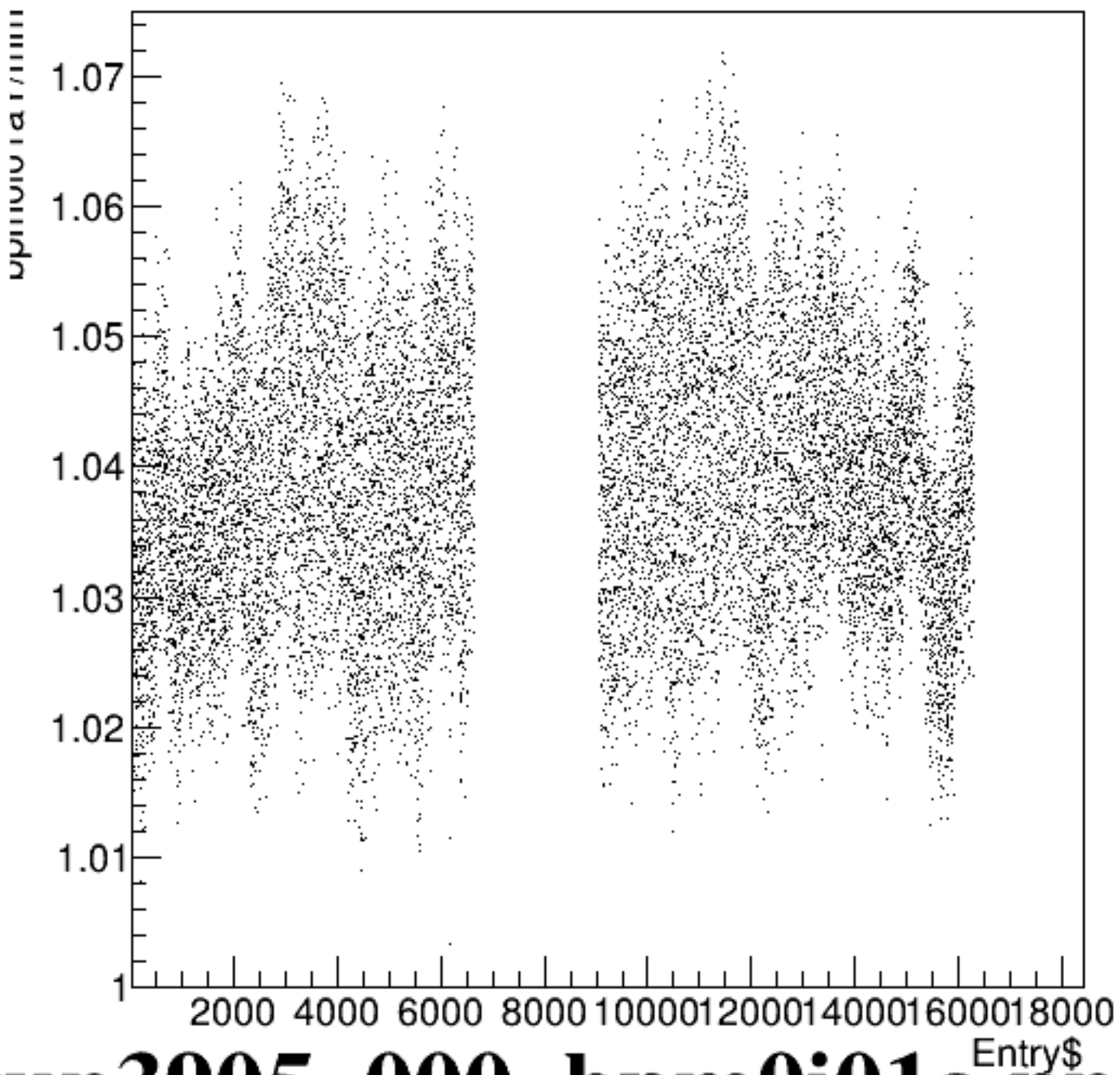
bpm0i01aY/mm:Entry$ {ErrorFlag==0}
