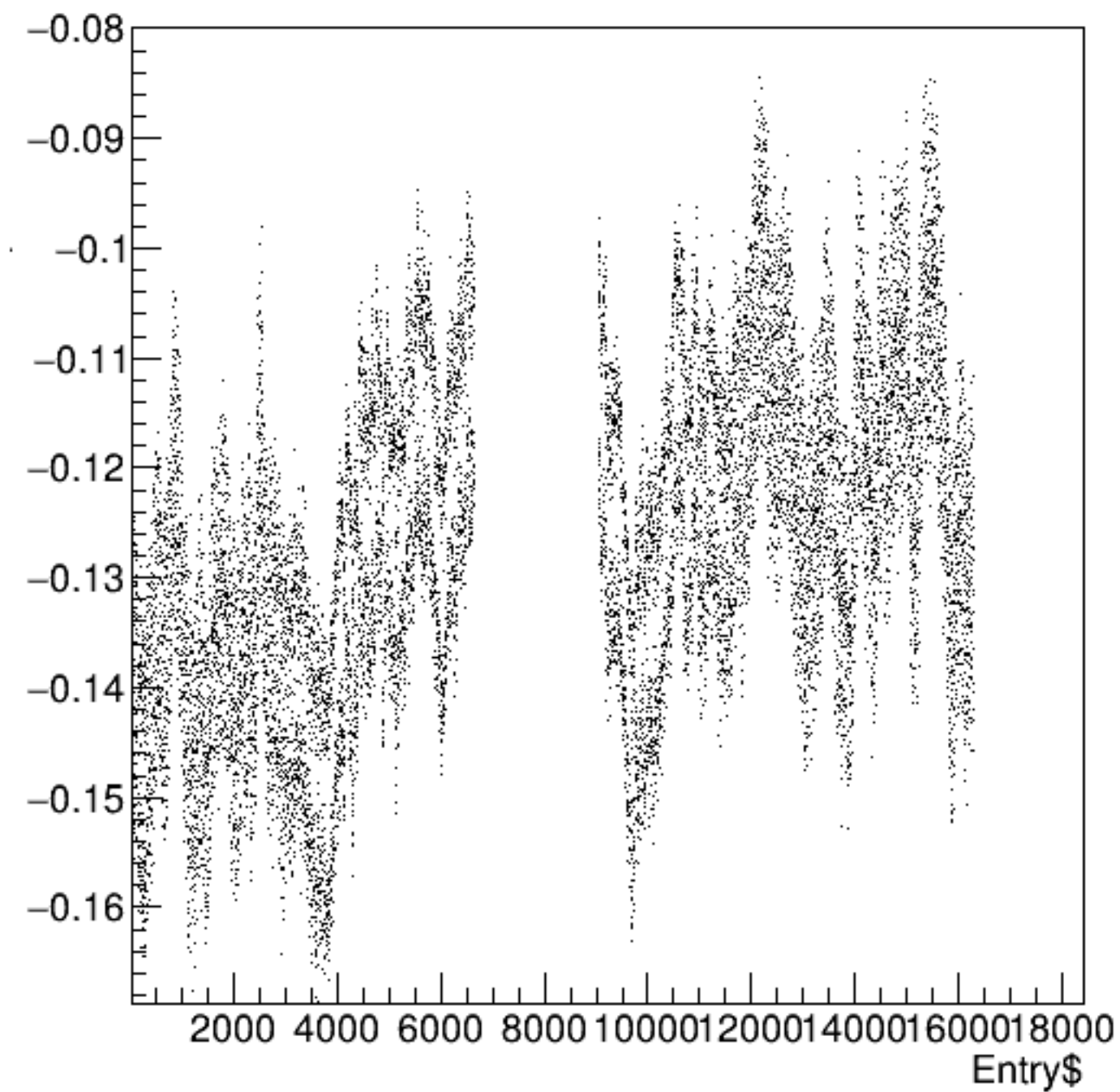
bpm1i02X/mm:Entry$ {ErrorFlag==0}
