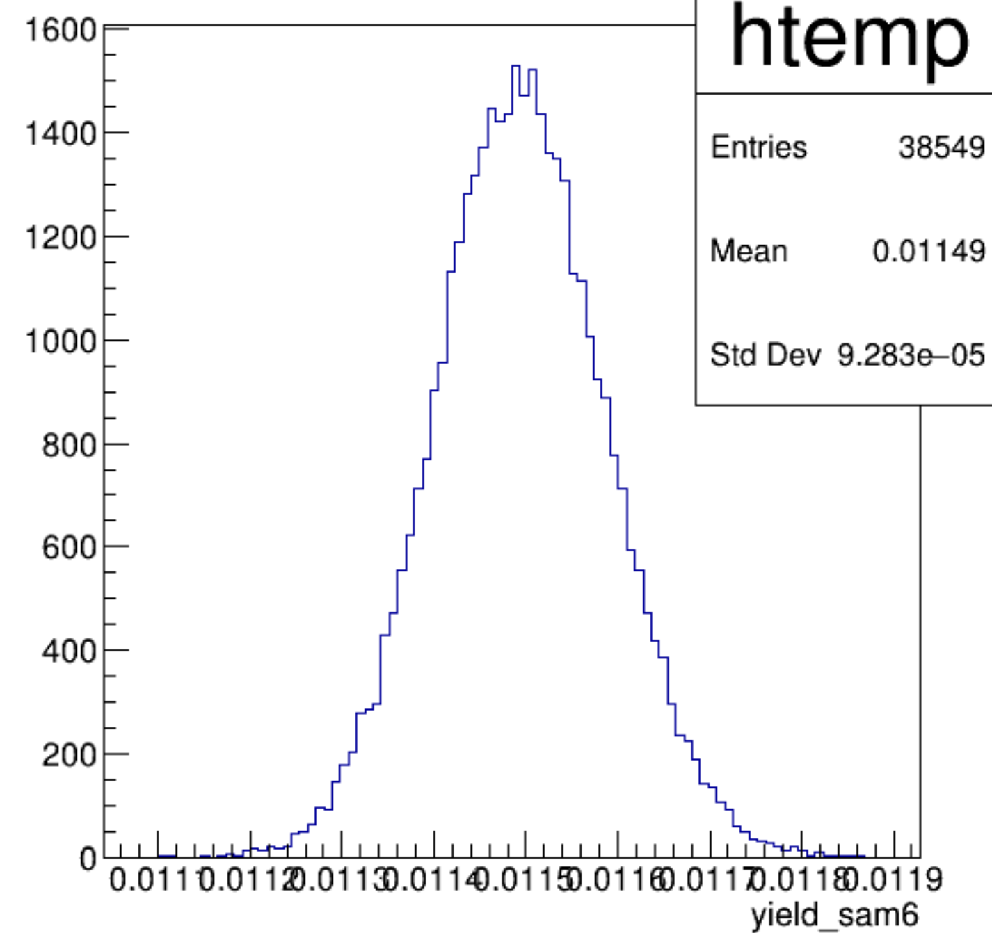
yield_sam6 {ErrorFlag==0}
