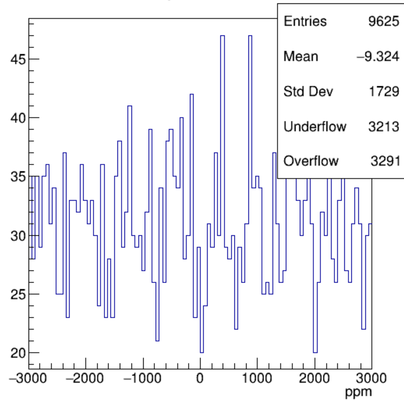
asym_sam2
