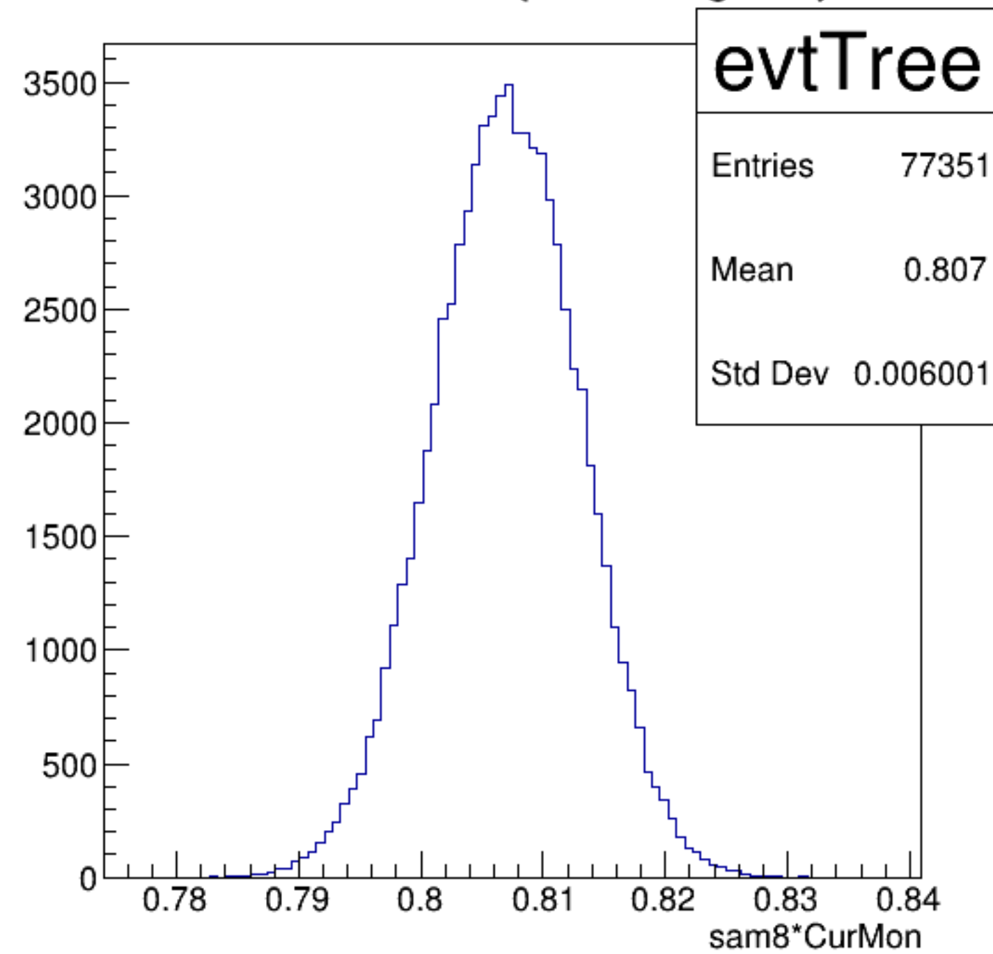
sam8*CurMon {ErrorFlag==0}
