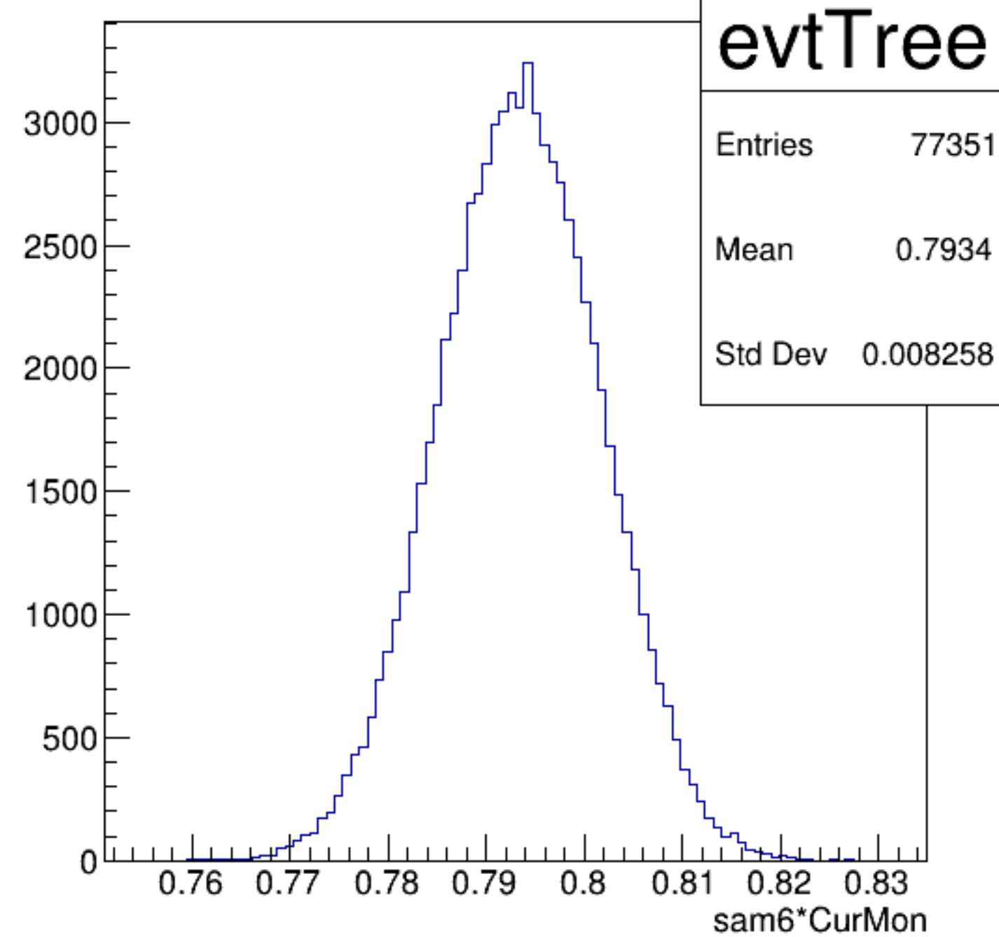
sam6*CurMon {ErrorFlag==0}
