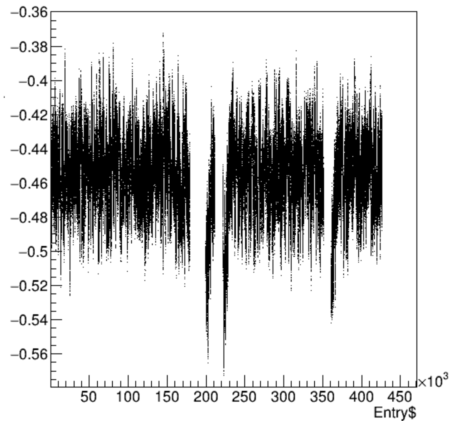
bpm2i02X/mm:Entry$ {ErrorFlag==0}
