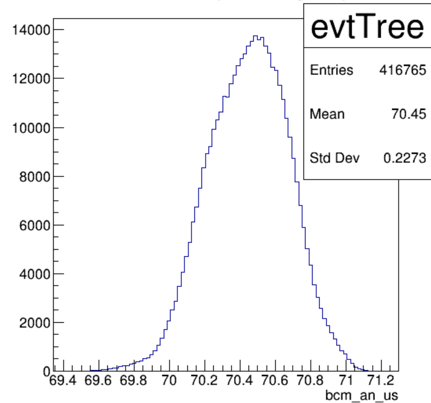
bcm_an_us {ErrorFlag==0}
