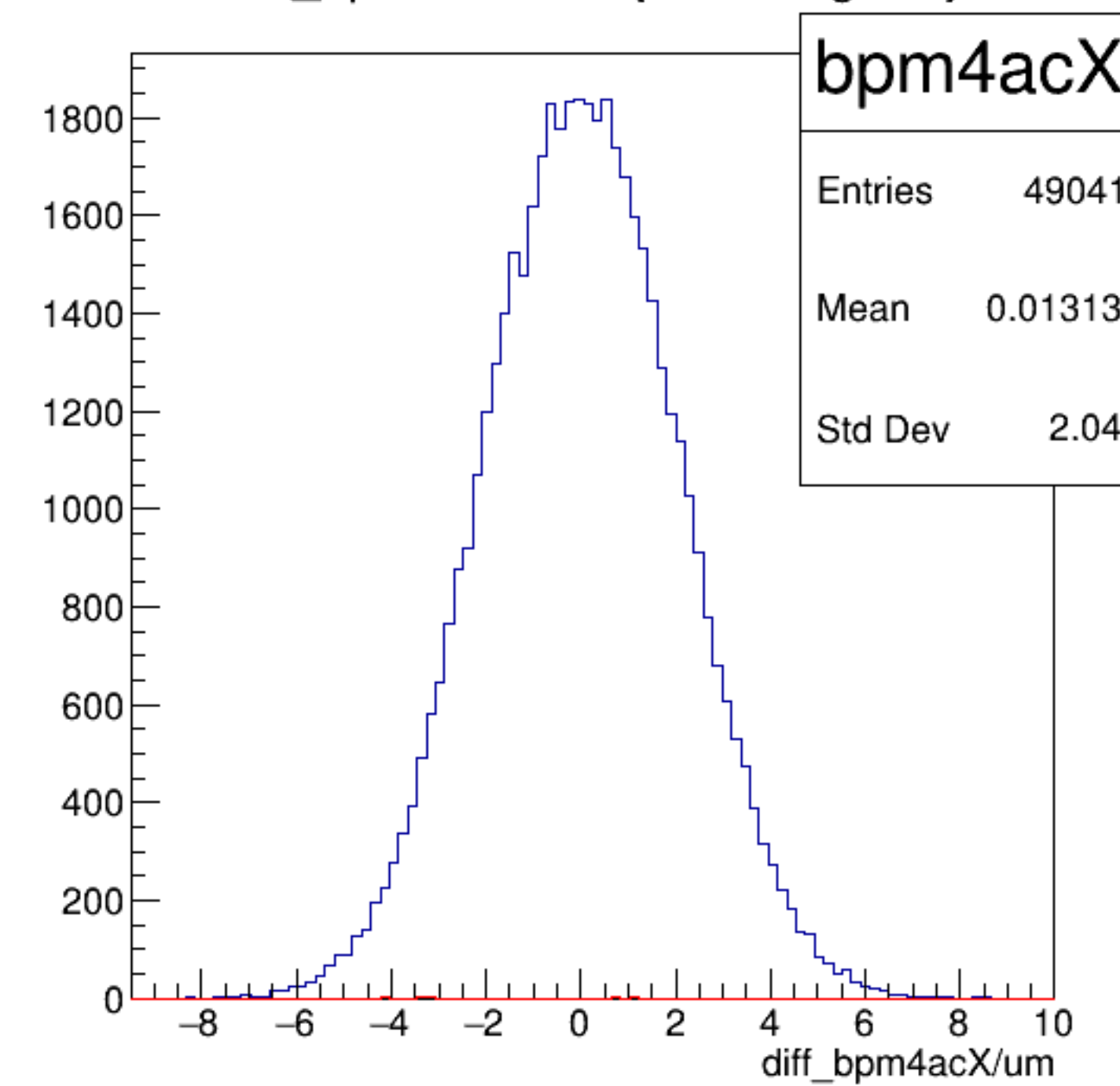
diff_bpm4acX/um {ErrorFlag==0}
