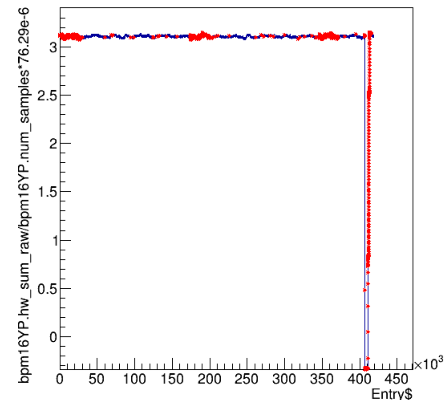
bpm16YP.hw_sum_raw/bpm16YP.num_samples*76.29e-6:Entry$
