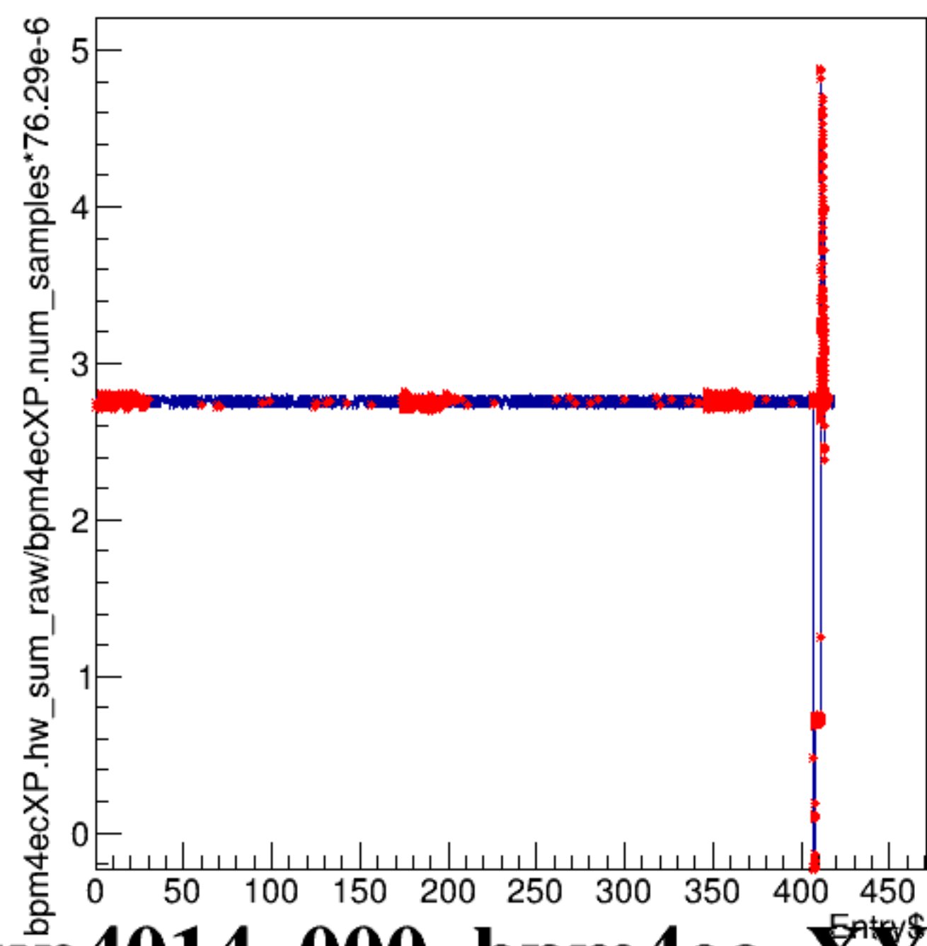
bpm4ecXP.hw_sum_raw/bpm4ecXP.num_samples*76.29e-6:Entry$
