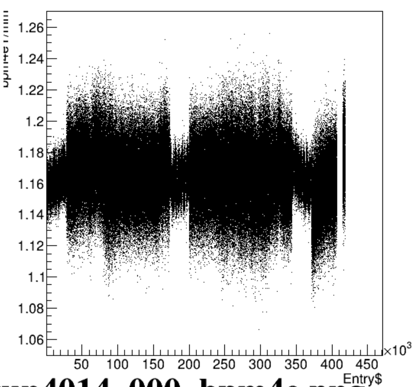
bpm4eY/mm:Entry$ {ErrorFlag==0}
