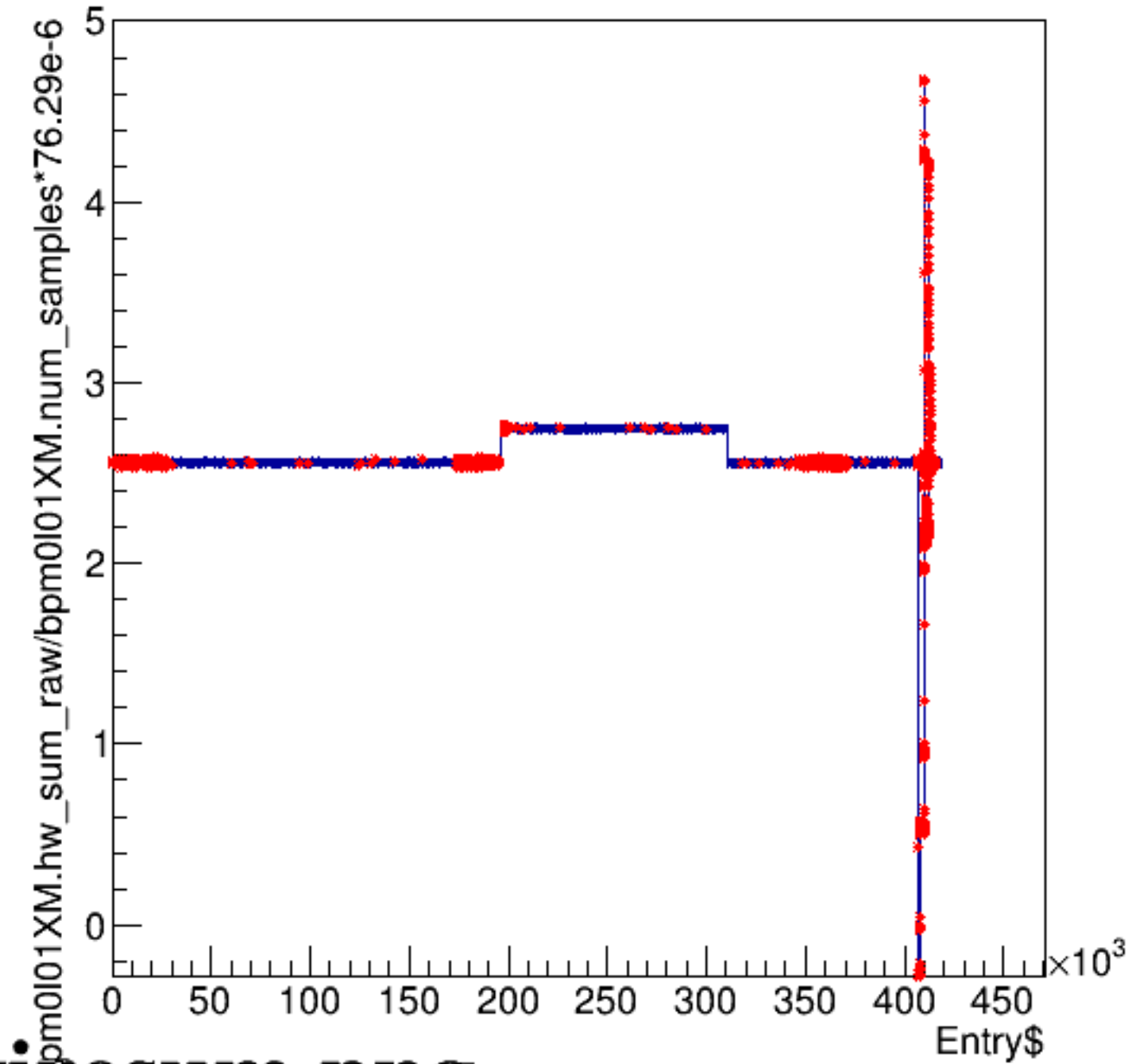
bpm0l01XM.hw_sum_raw/bpm0l01XM.num_samples*76.29e-6:Entry$
