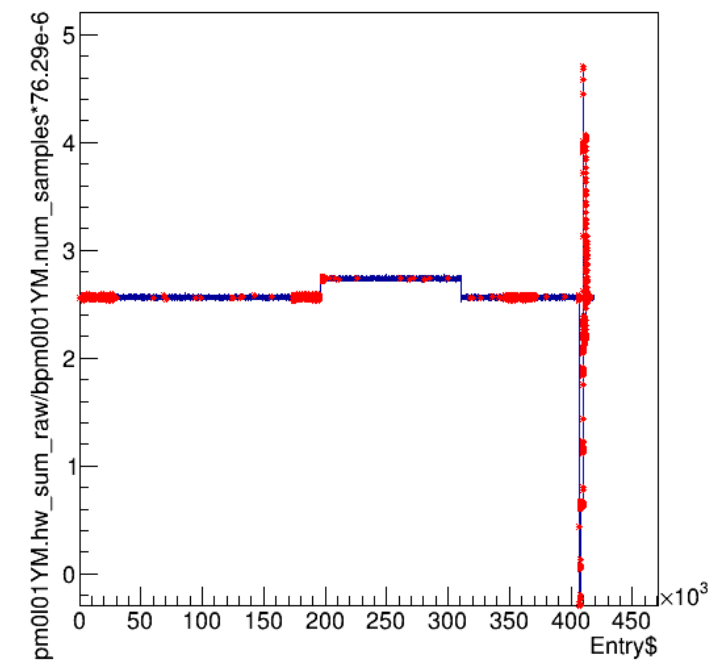
bpm0l01YM.hw_sum_raw/bpm0l01YM.num_samples*76.29e-6:Entry$
