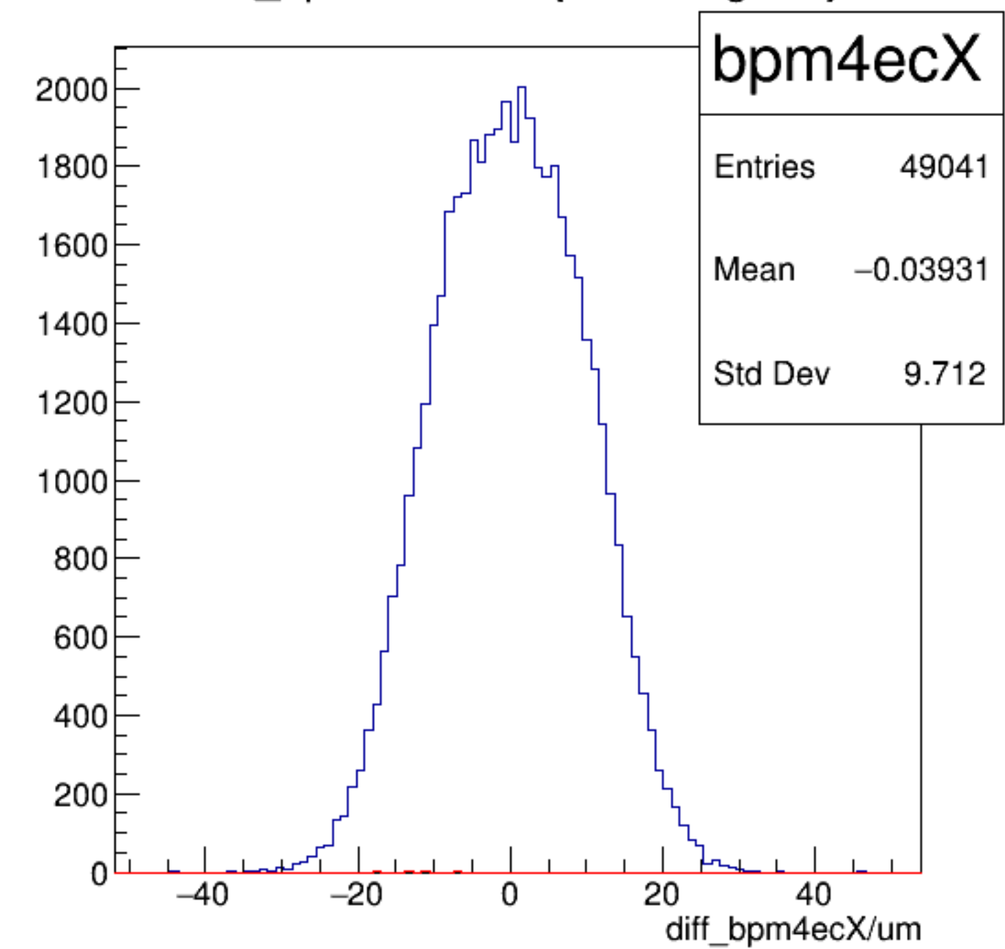
diff_bpm4ecX/um {ErrorFlag==0}
