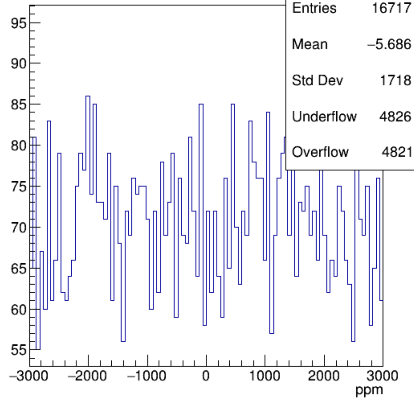
asym_sam4
