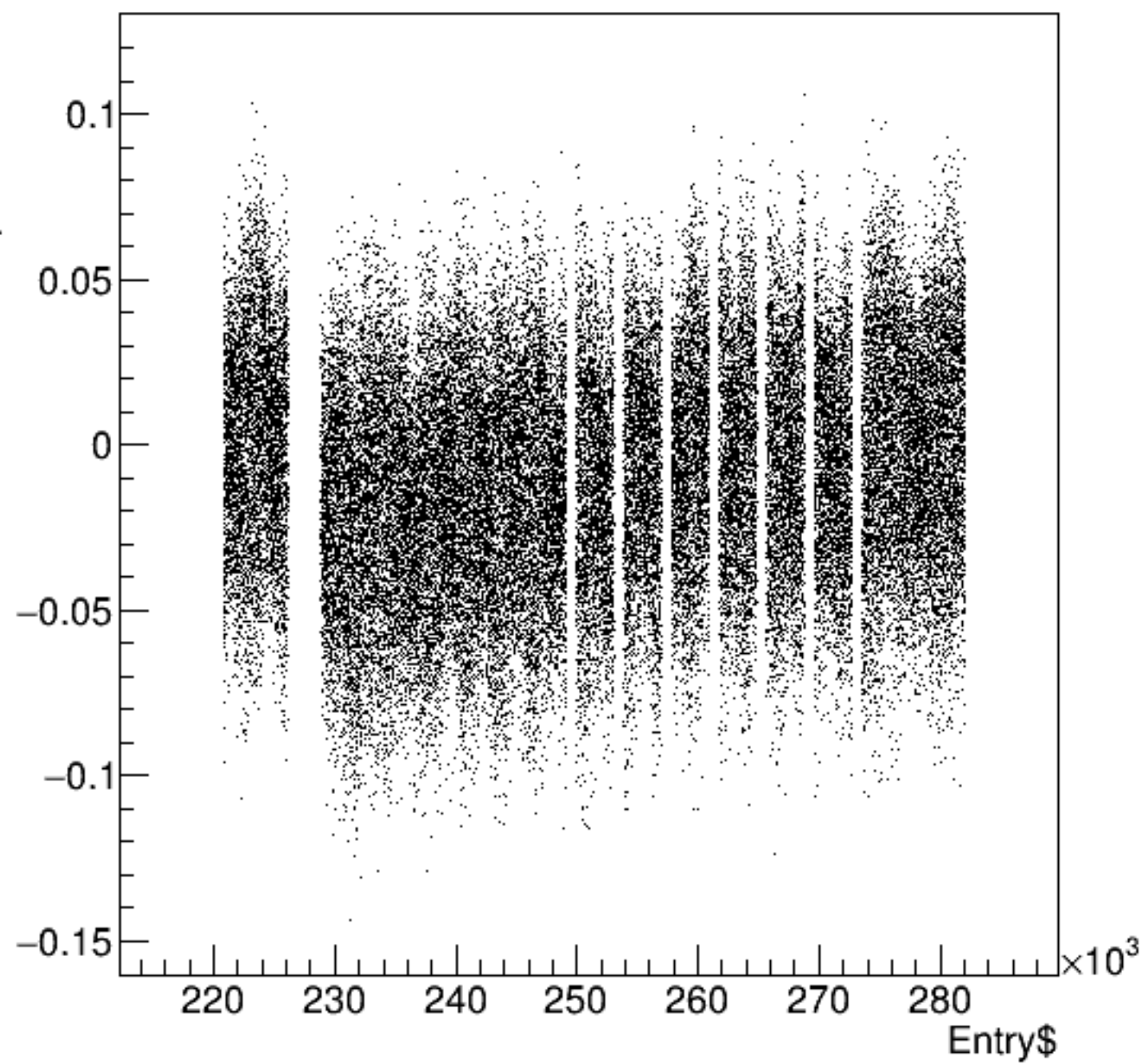
bpm0l01X/mm:Entry$ {ErrorFlag==0}
