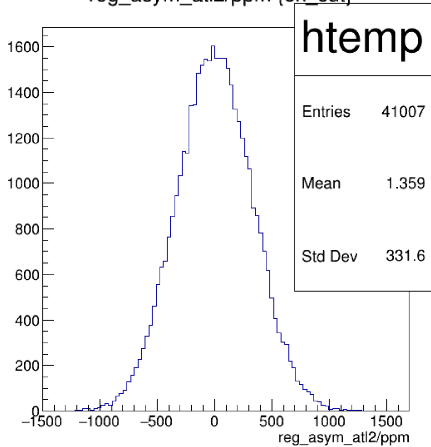
reg_asym_atl2/ppm {ok_cut}
