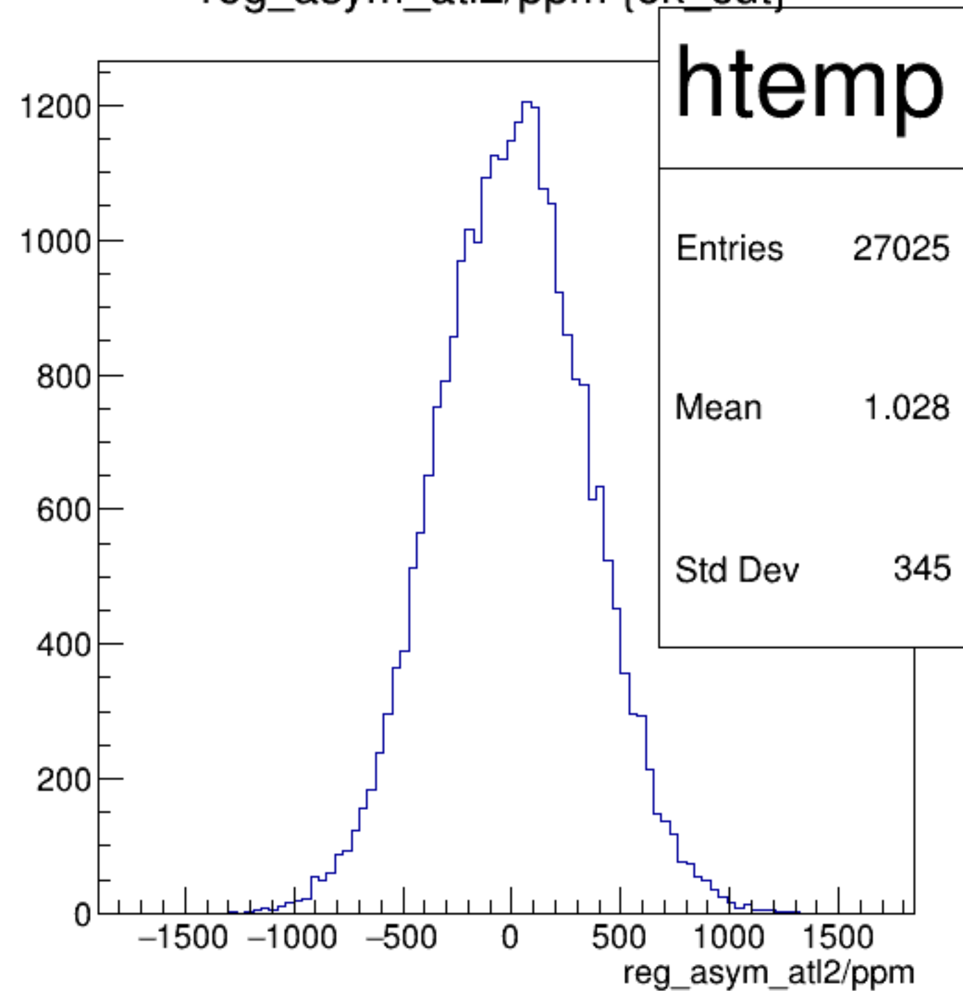
reg_asym_atl2/ppm {ok_cut}
