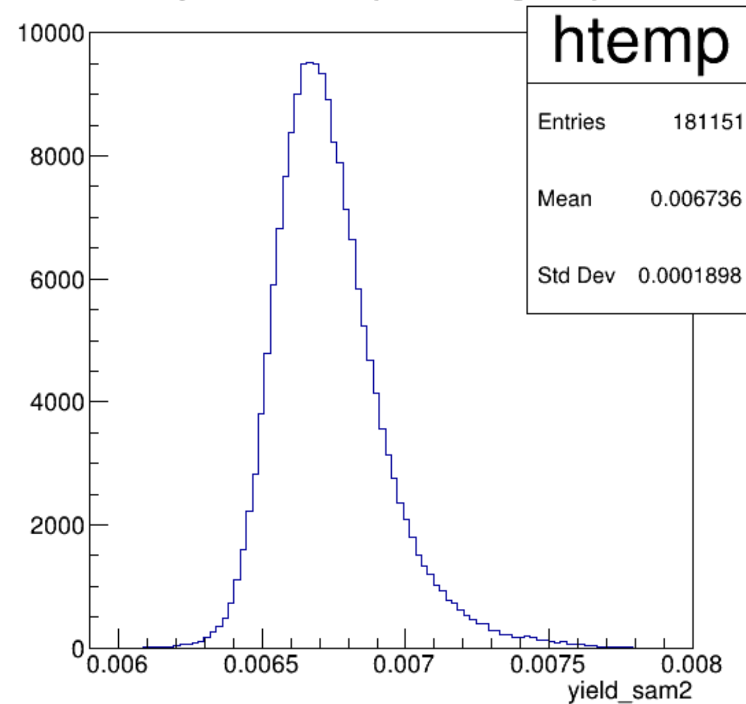
yield_sam2 {ErrorFlag==0}
