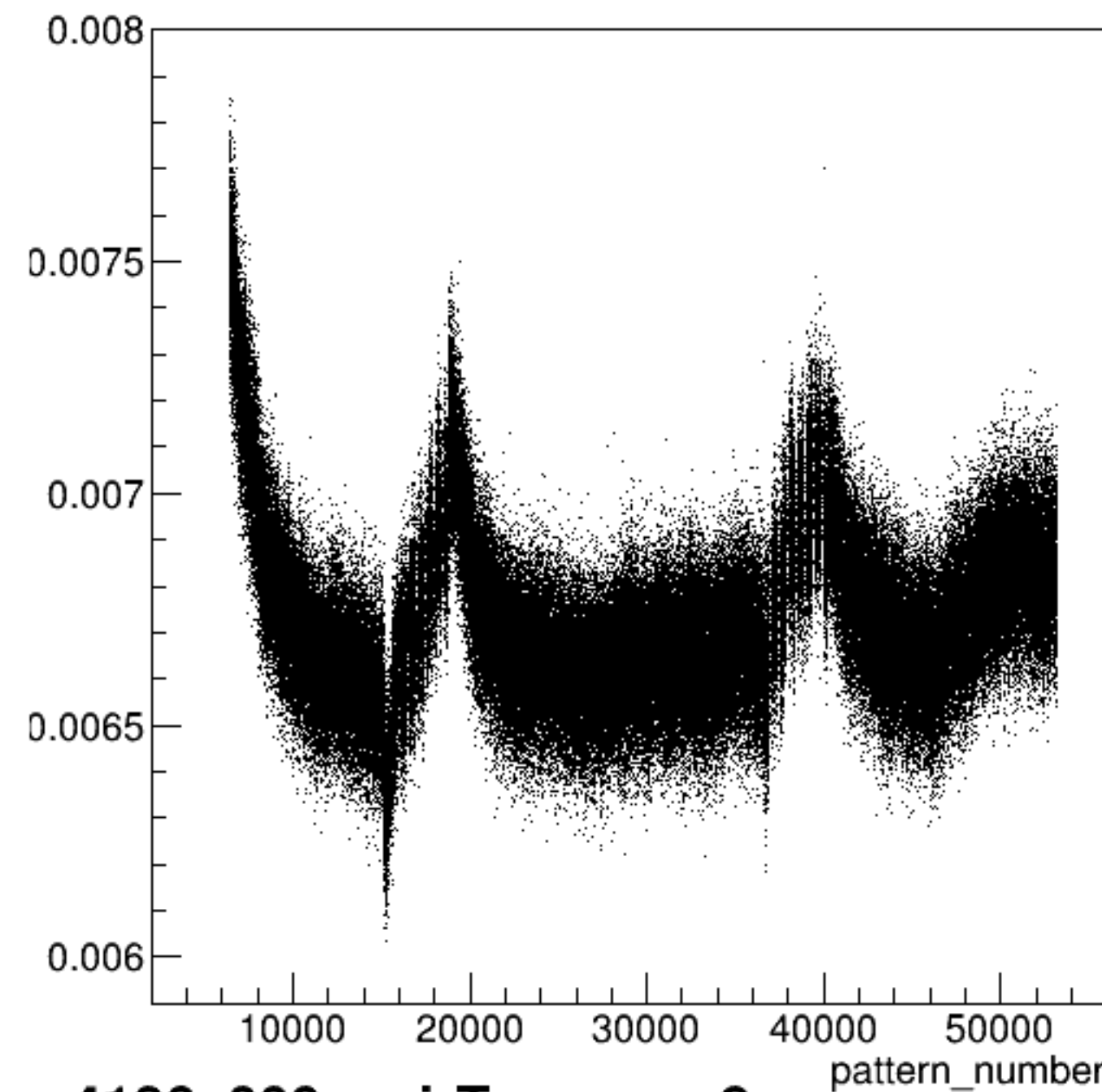
yield_sam2:pattern_number {ErrorFlag==0}
