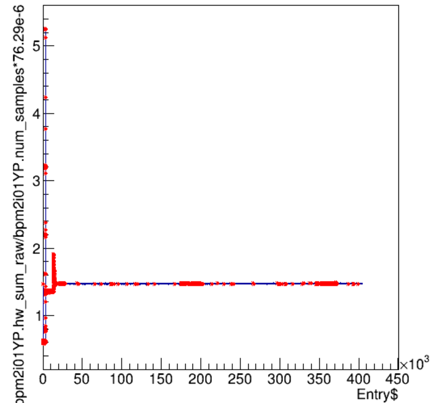
bpm2i01YP.hw_sum_raw/bpm2i01YP.num_samples*76.29e-6:Entry$
