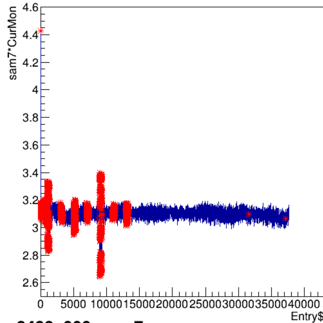
sam7*CurMon:Entry$
