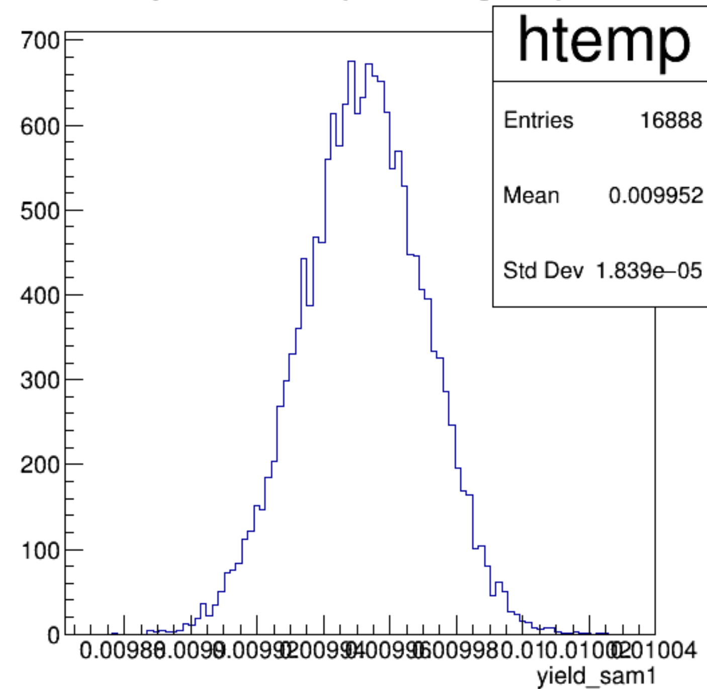
yield_sam1 {ErrorFlag==0}
