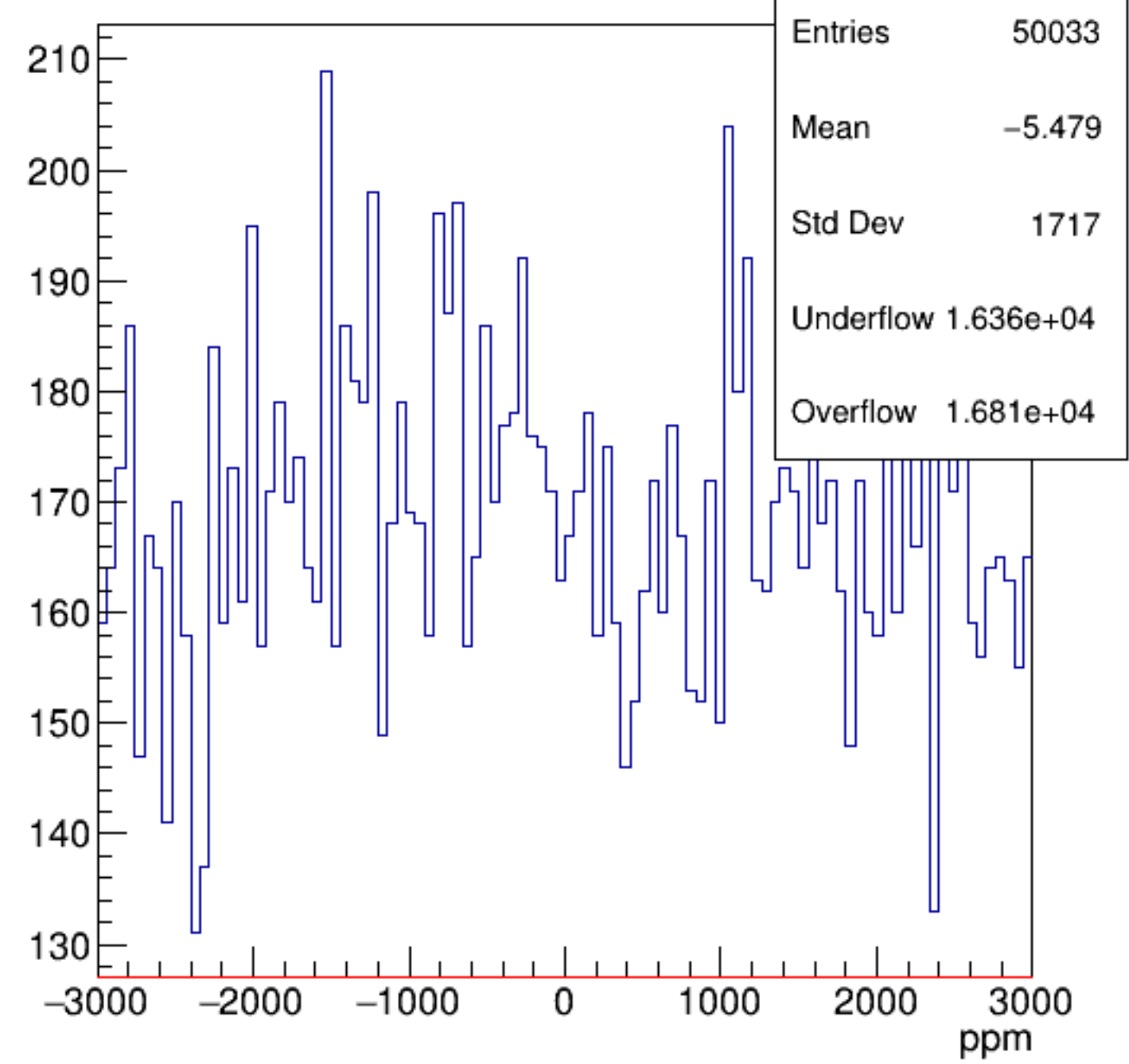
asym_sam2
