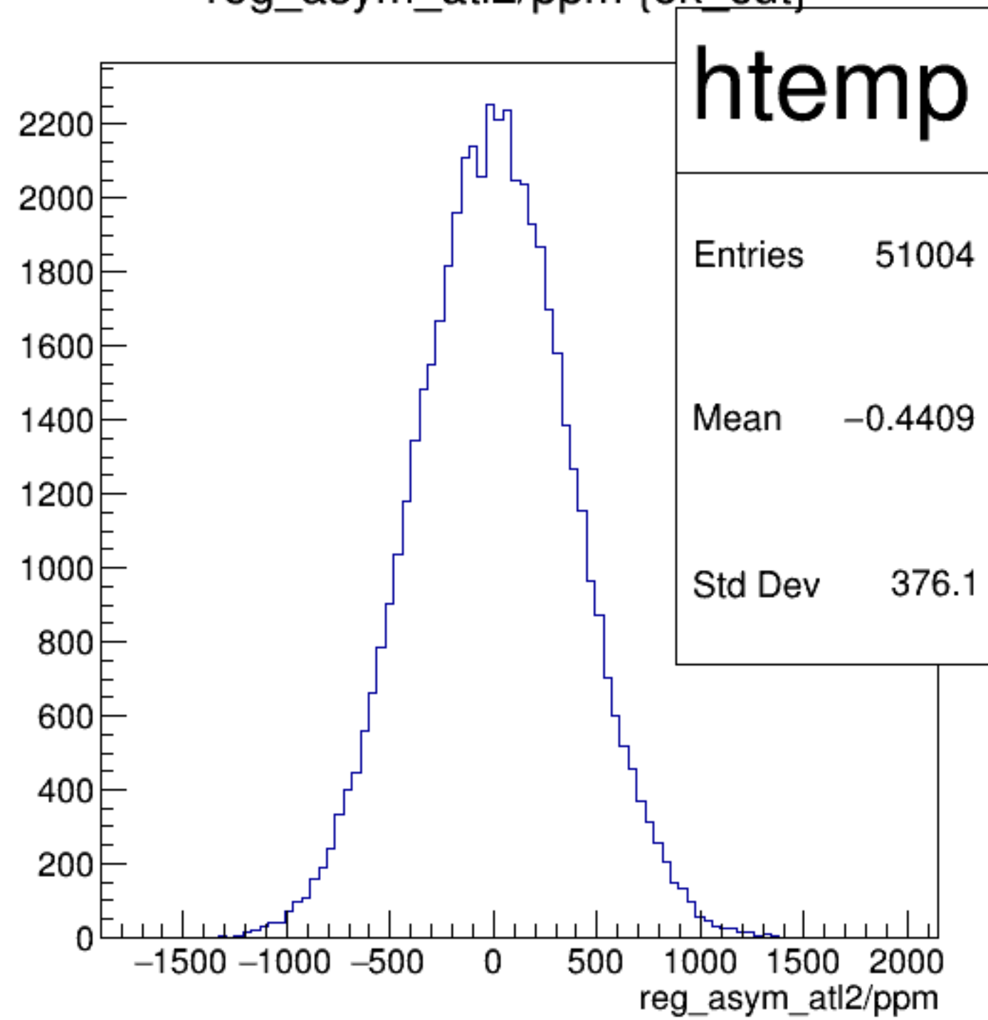
reg_asym_atl2/ppm {ok_cut}
