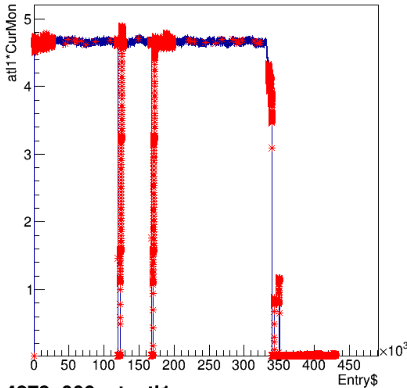
atl1*CurMon:Entry$
