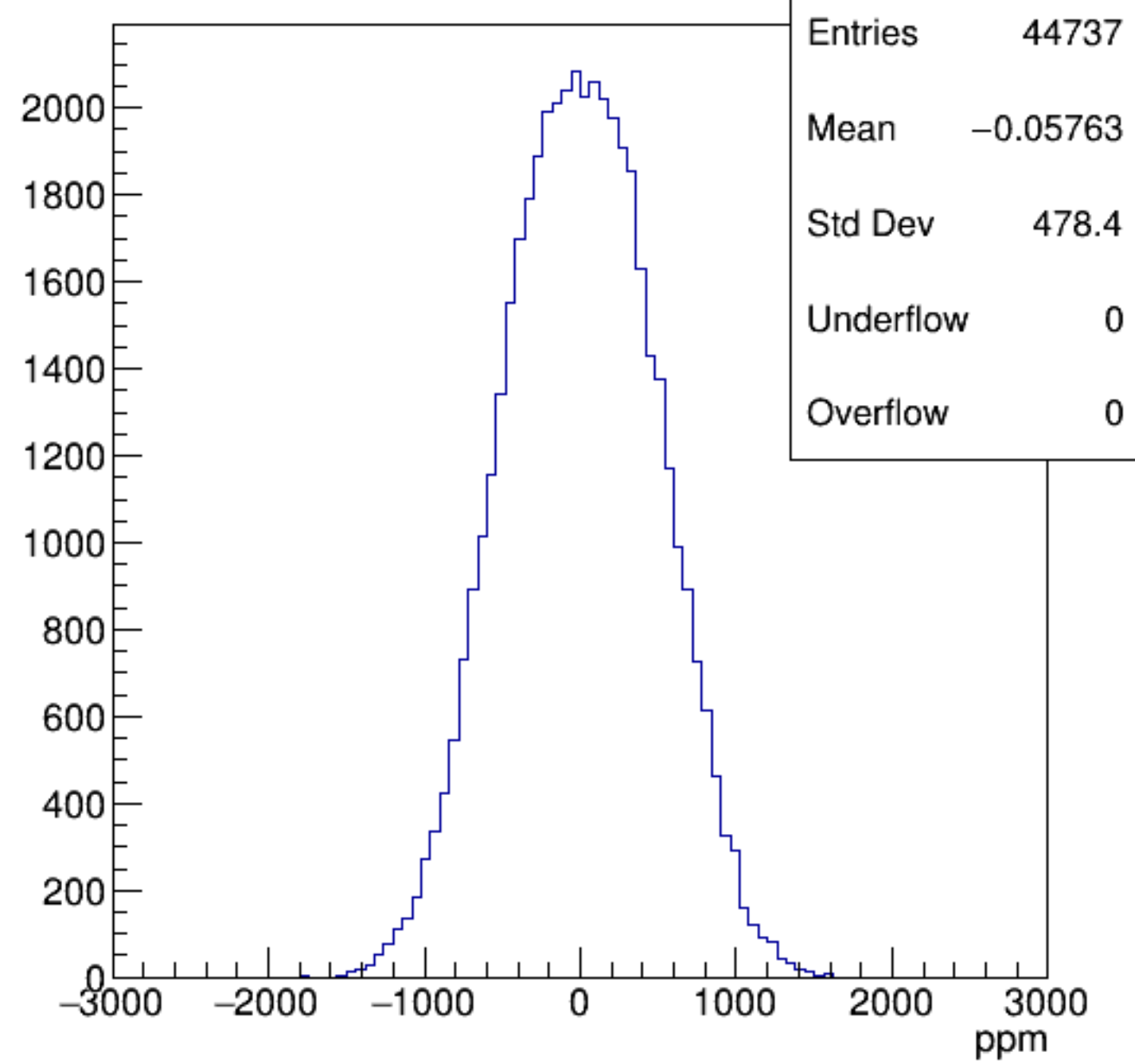
asym_usl
