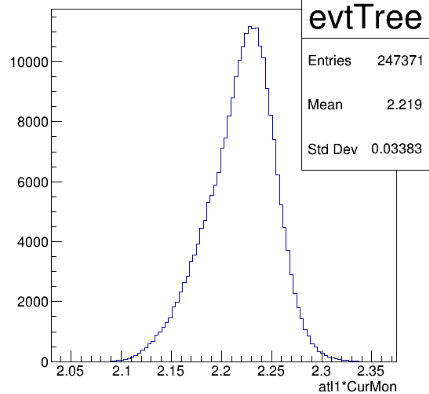
atl1*CurMon {ErrorFlag==0}
