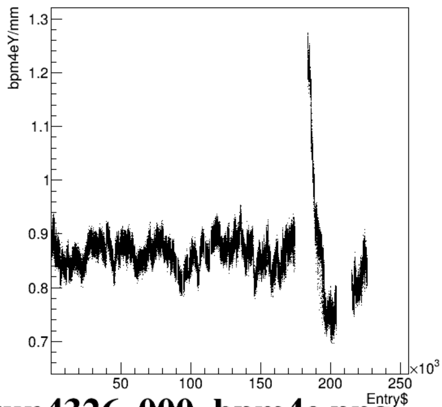
bpm4eY/mm:Entry$ {ErrorFlag==0}
