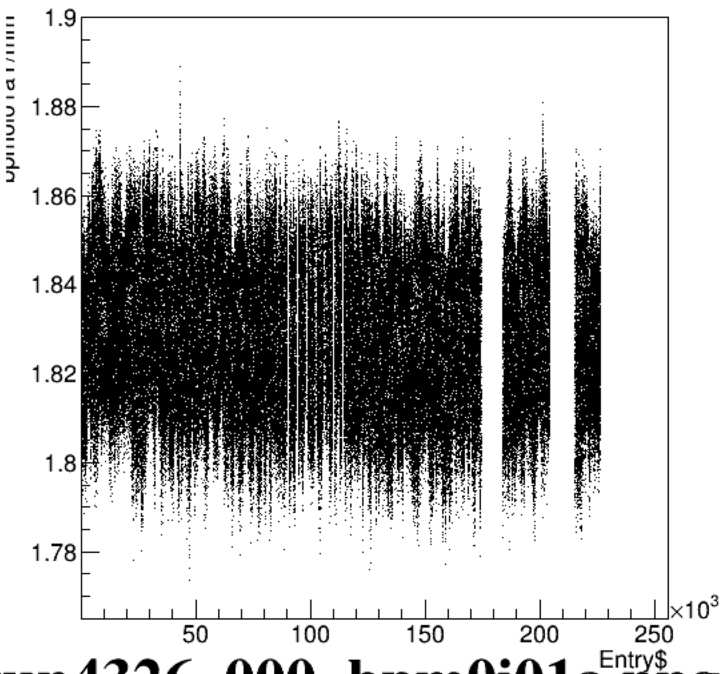
bpm0i01aY/mm:Entry$ {ErrorFlag==0}
