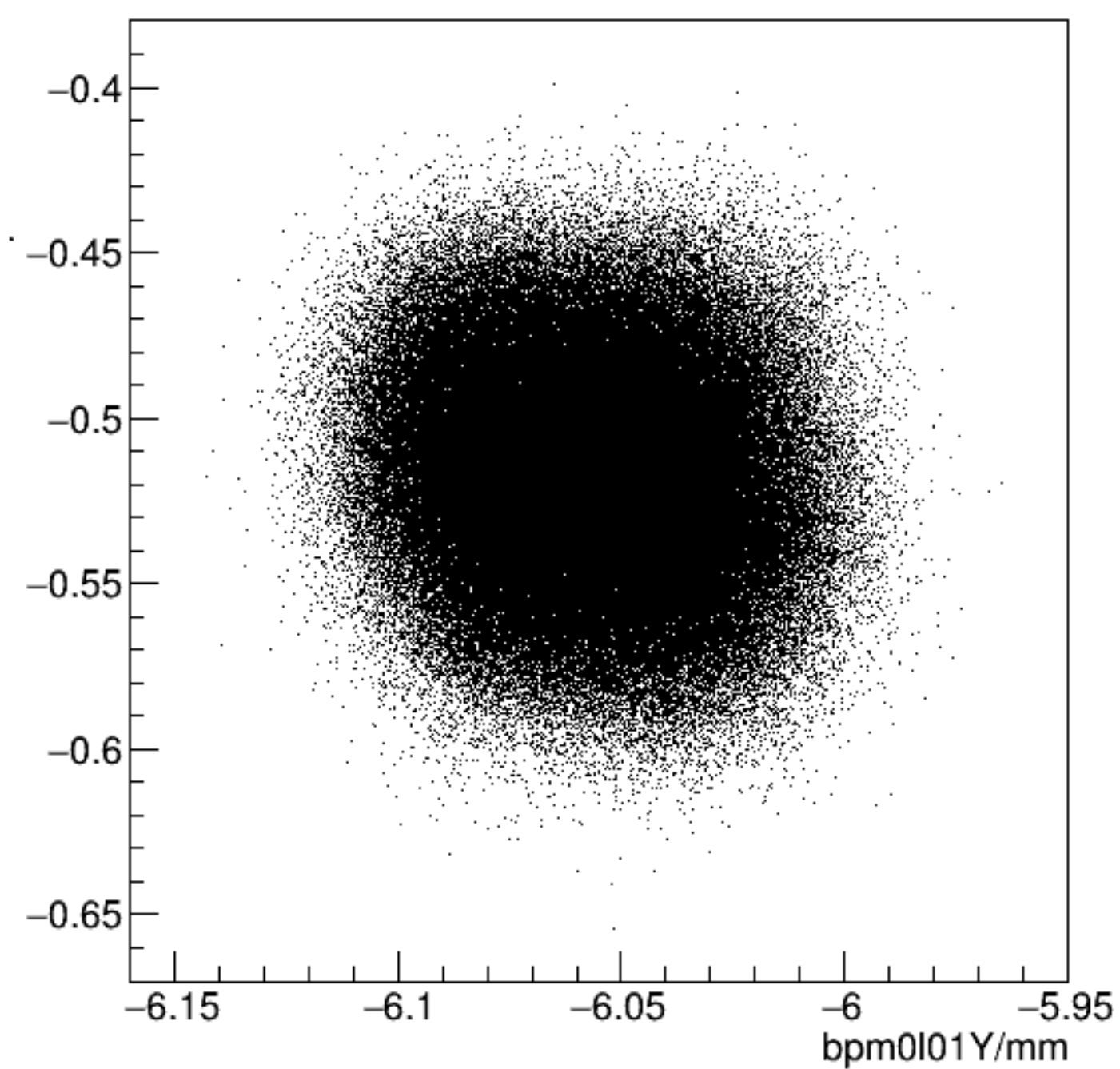
bpm0l01X/mm:bpm0l01Y/mm {ErrorFlag==0}
