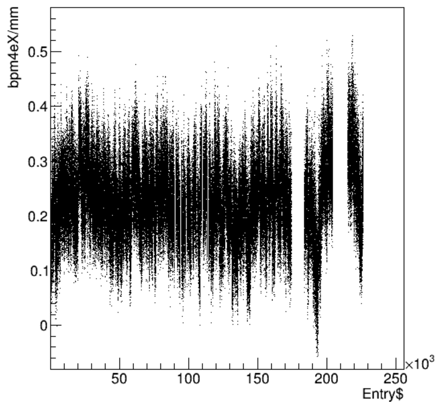
bpm4eX/mm:Entry$ {ErrorFlag==0}
