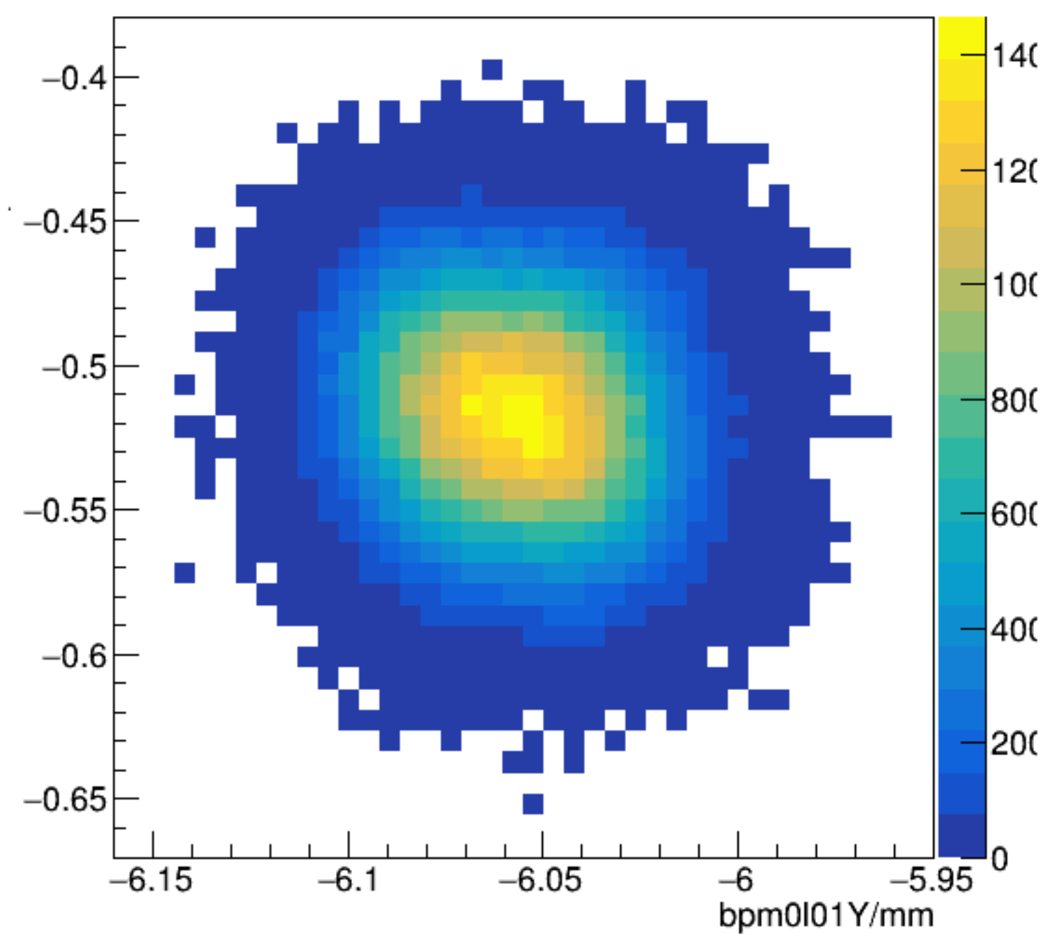
bpm0l01X/mm:bpm0l01Y/mm {ErrorFlag==0}
