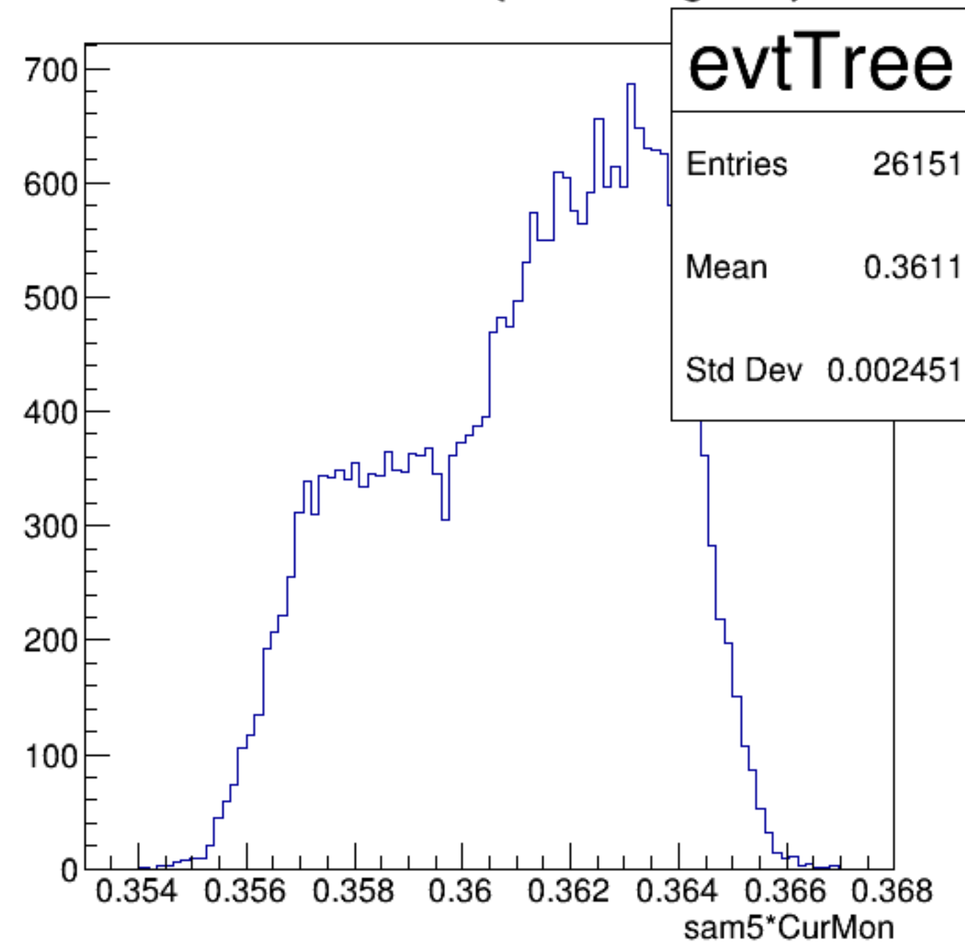
sam5*CurMon {ErrorFlag==0}
