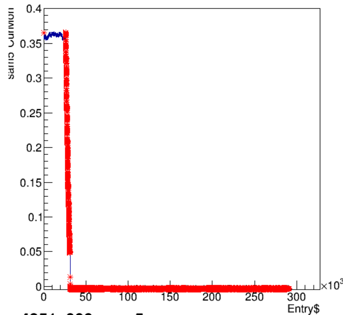
sam5*CurMon:Entry$
