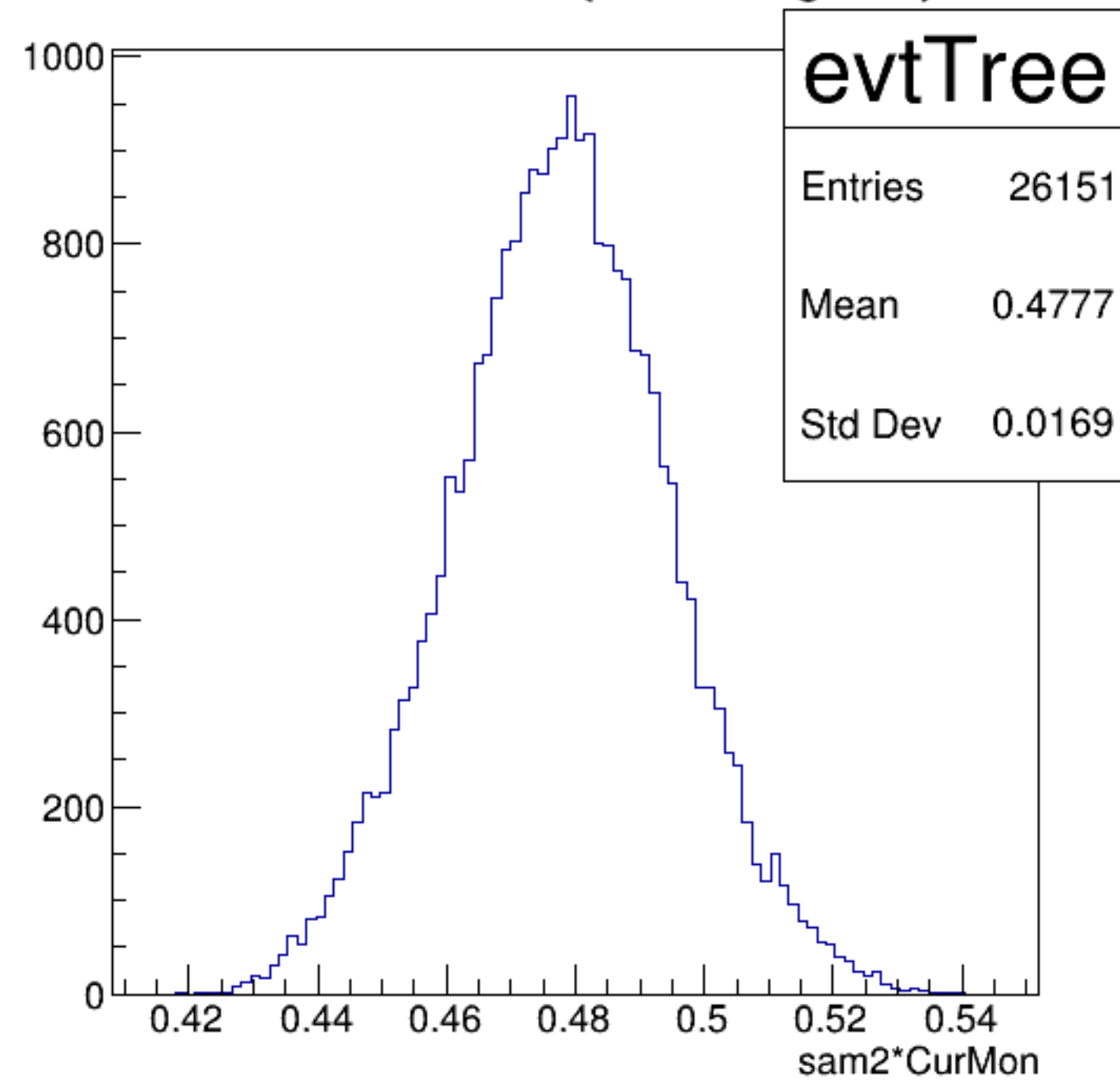
sam2*CurMon {ErrorFlag==0}
