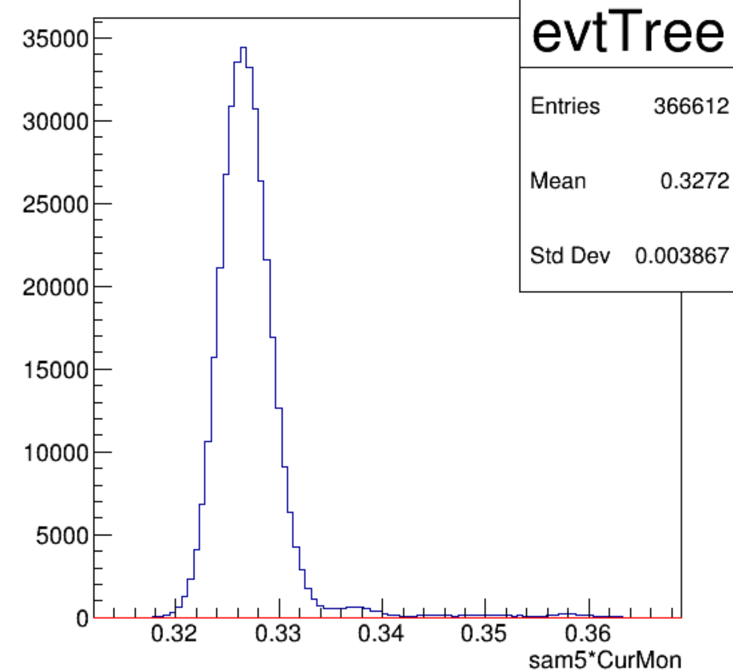
sam5*CurMon {ErrorFlag==0}
