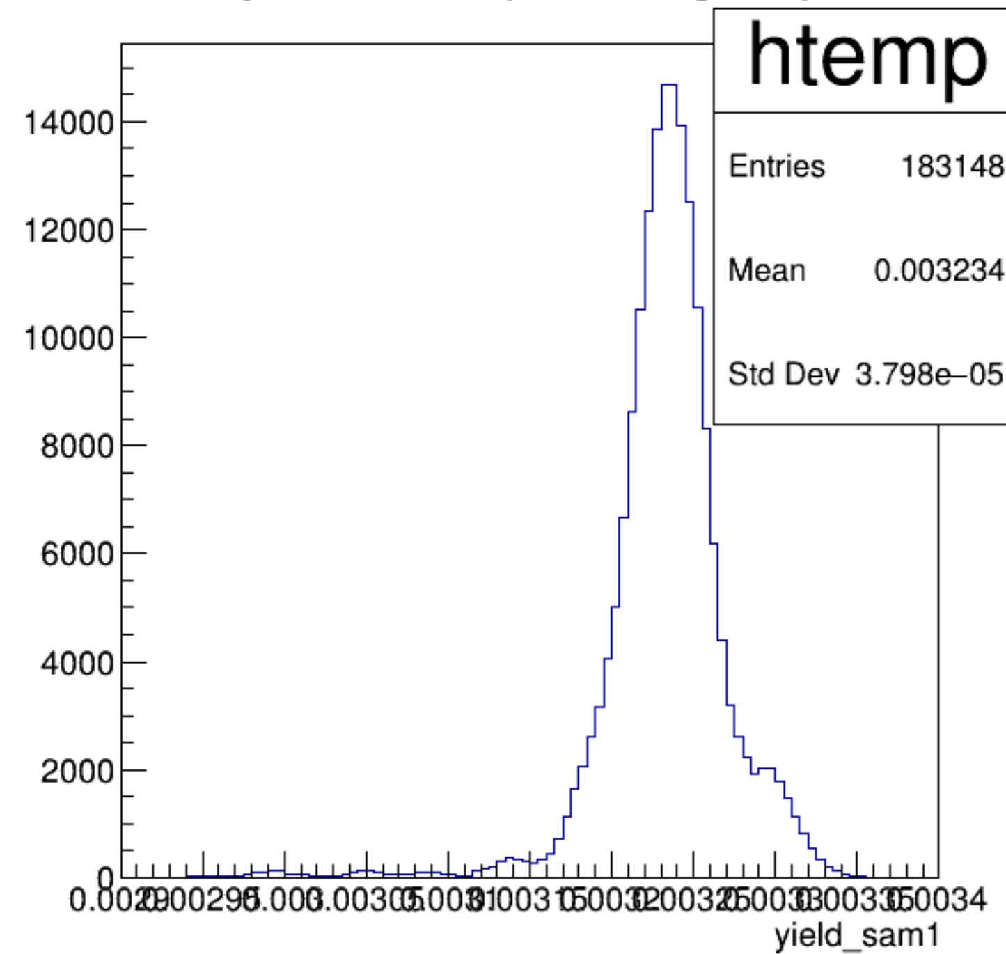
yield_sam1 {ErrorFlag==0}
