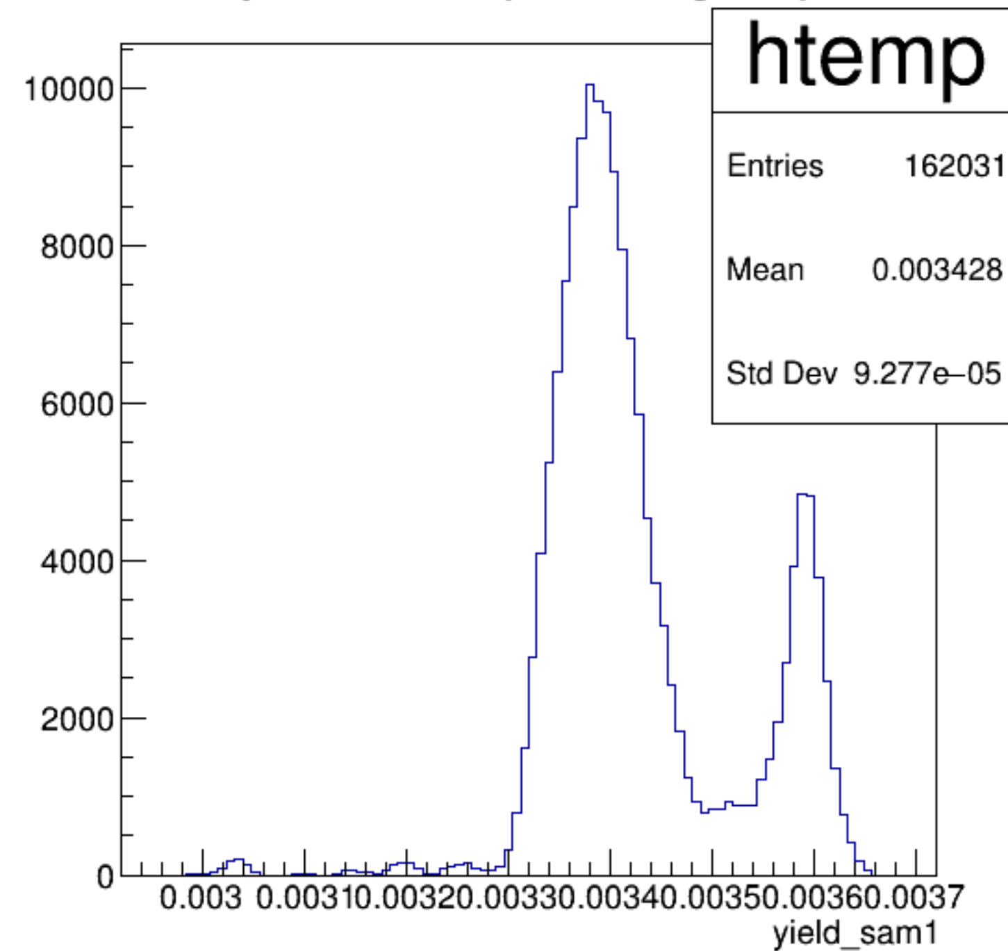
yield_sam1 {ErrorFlag==0}
