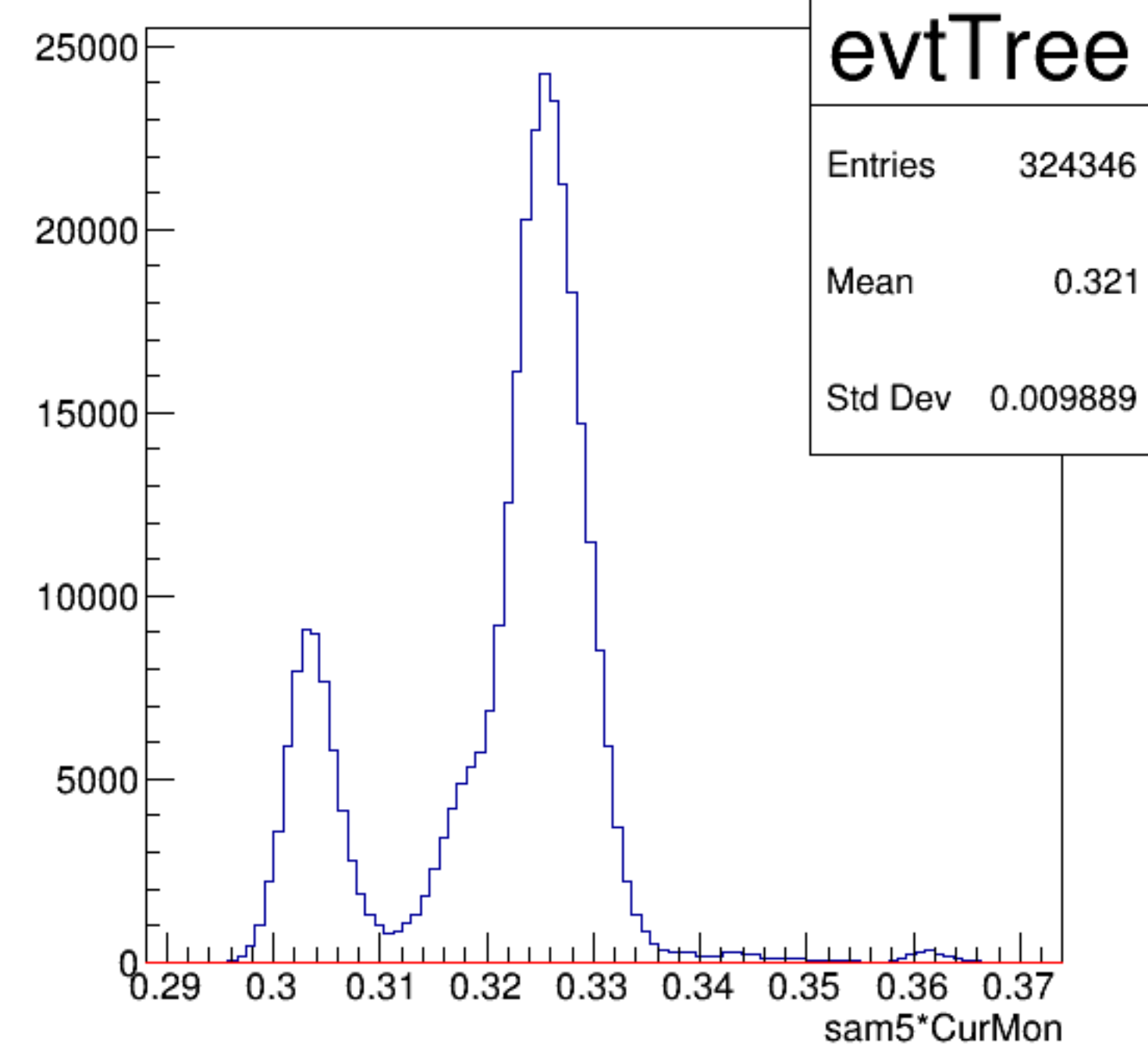
sam5*CurMon {ErrorFlag==0}
