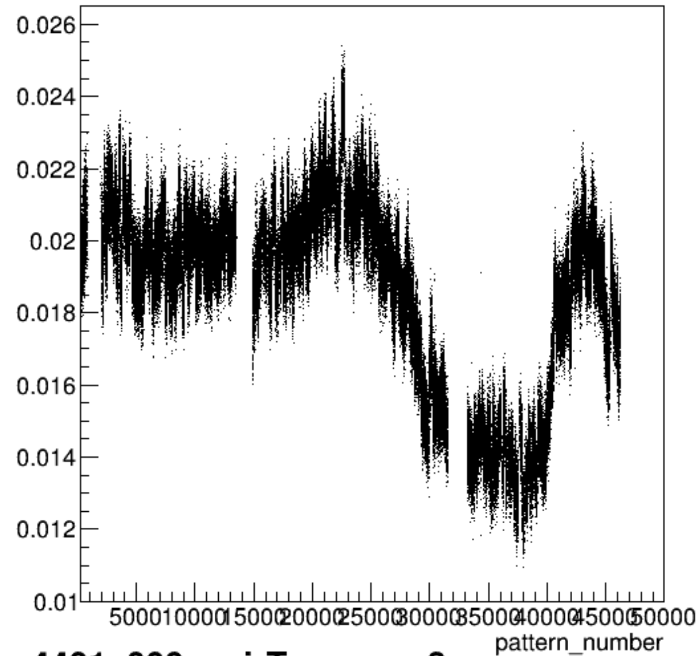
yield_sam3:pattern_number {ErrorFlag==0}
