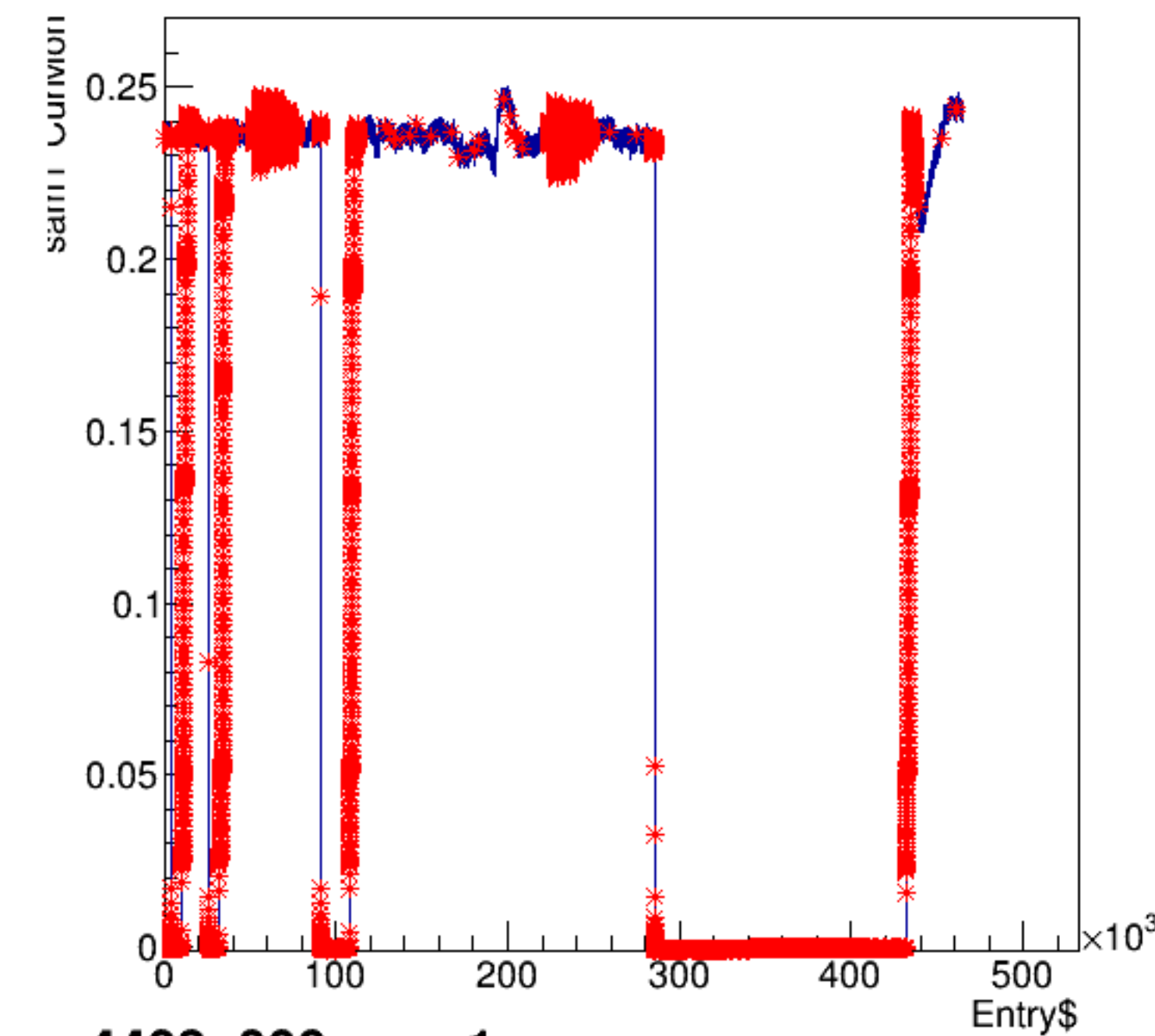
sam1*CurMon:Entry$
