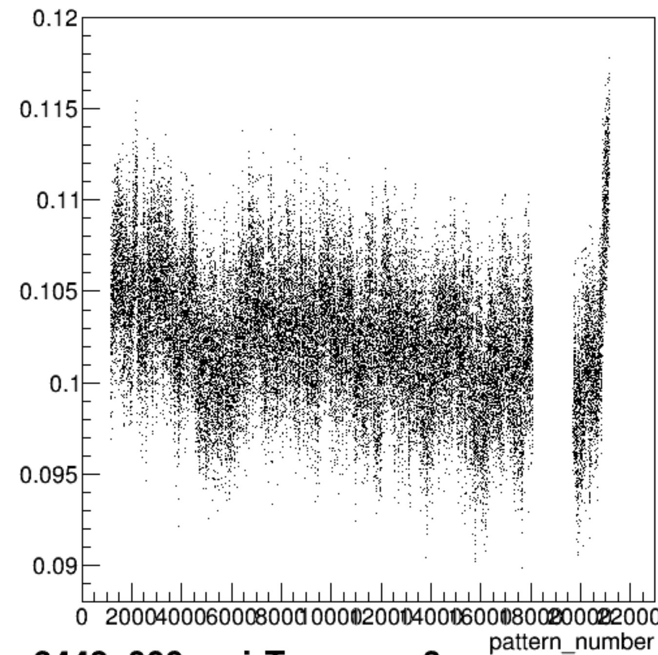
yield_sam3:pattern_number {ErrorFlag==0}
