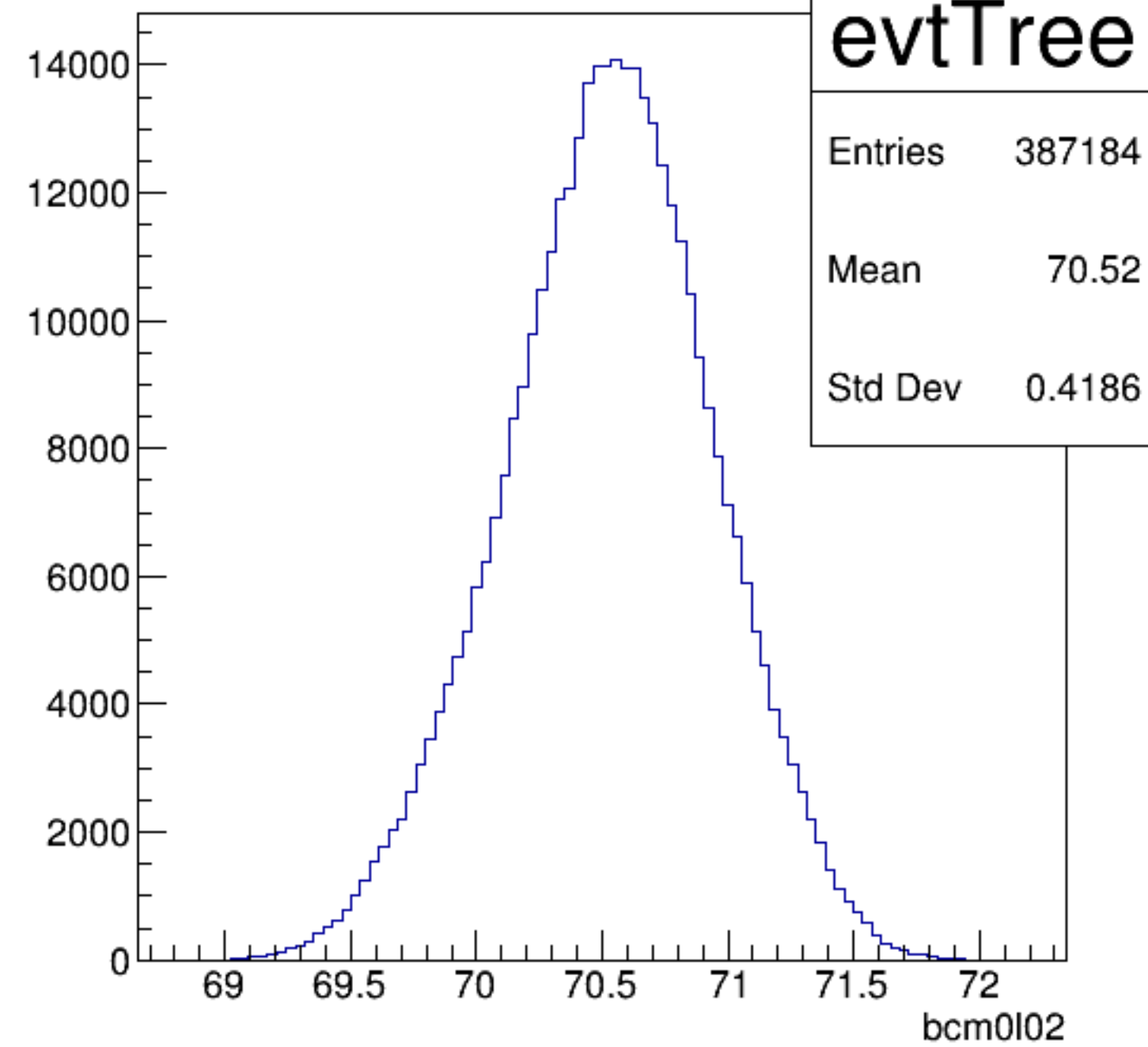
bcm0l02 {ErrorFlag==0}
