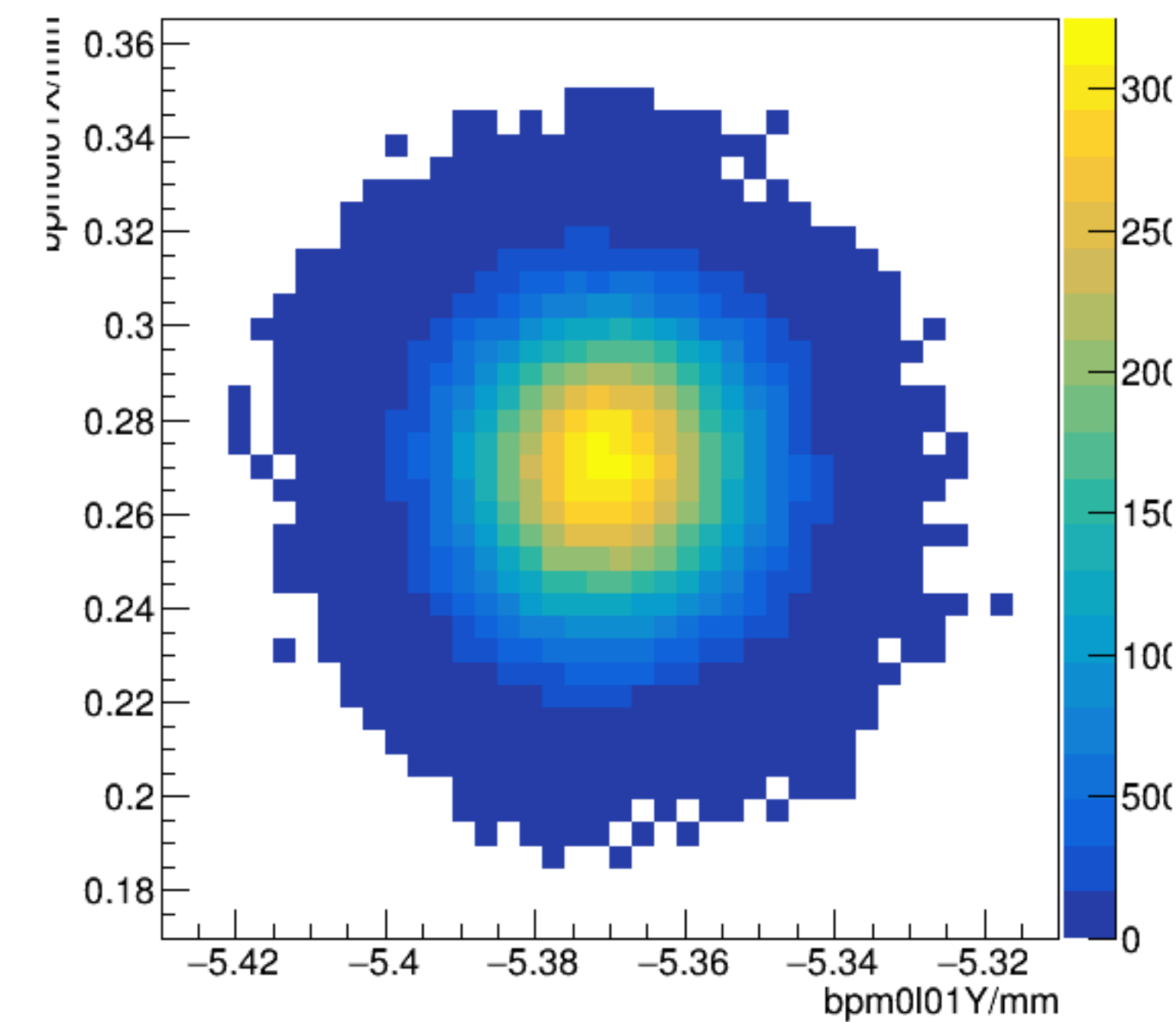
bpm0l01X/mm:bpm0l01Y/mm {ErrorFlag==0}
