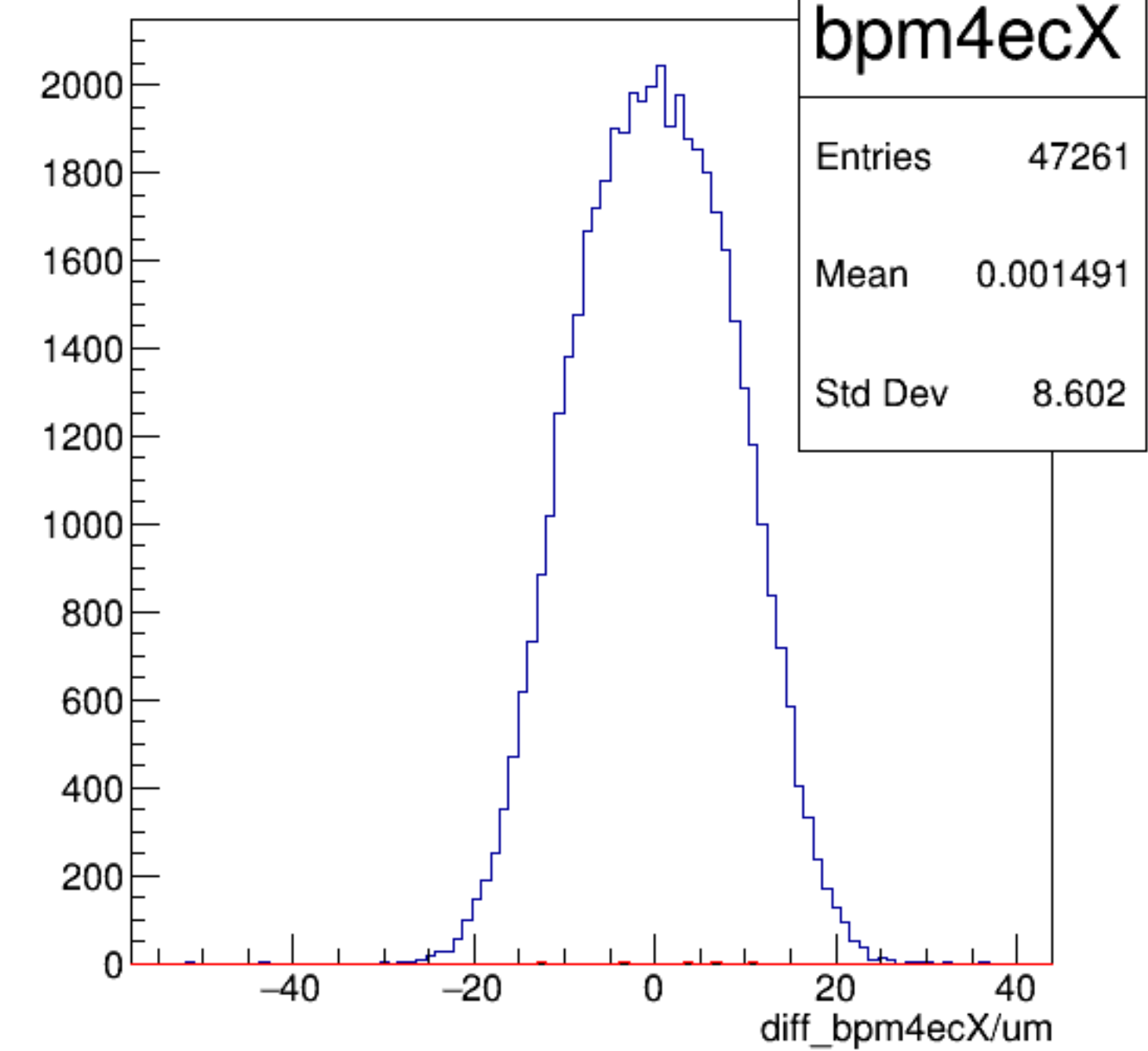
diff_bpm4ecX/um {ErrorFlag==0}
