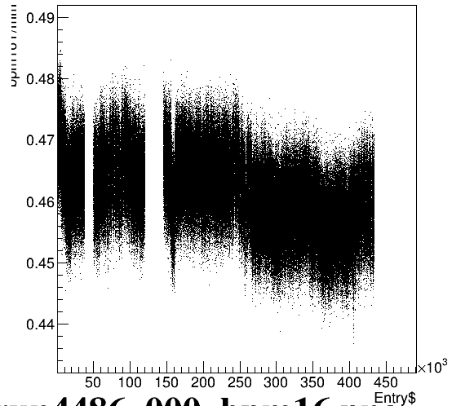
bpm16Y/mm:Entry$ {ErrorFlag==0}
