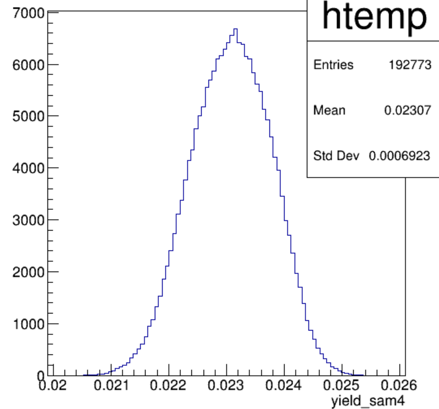
yield_sam4 {ErrorFlag==0}
