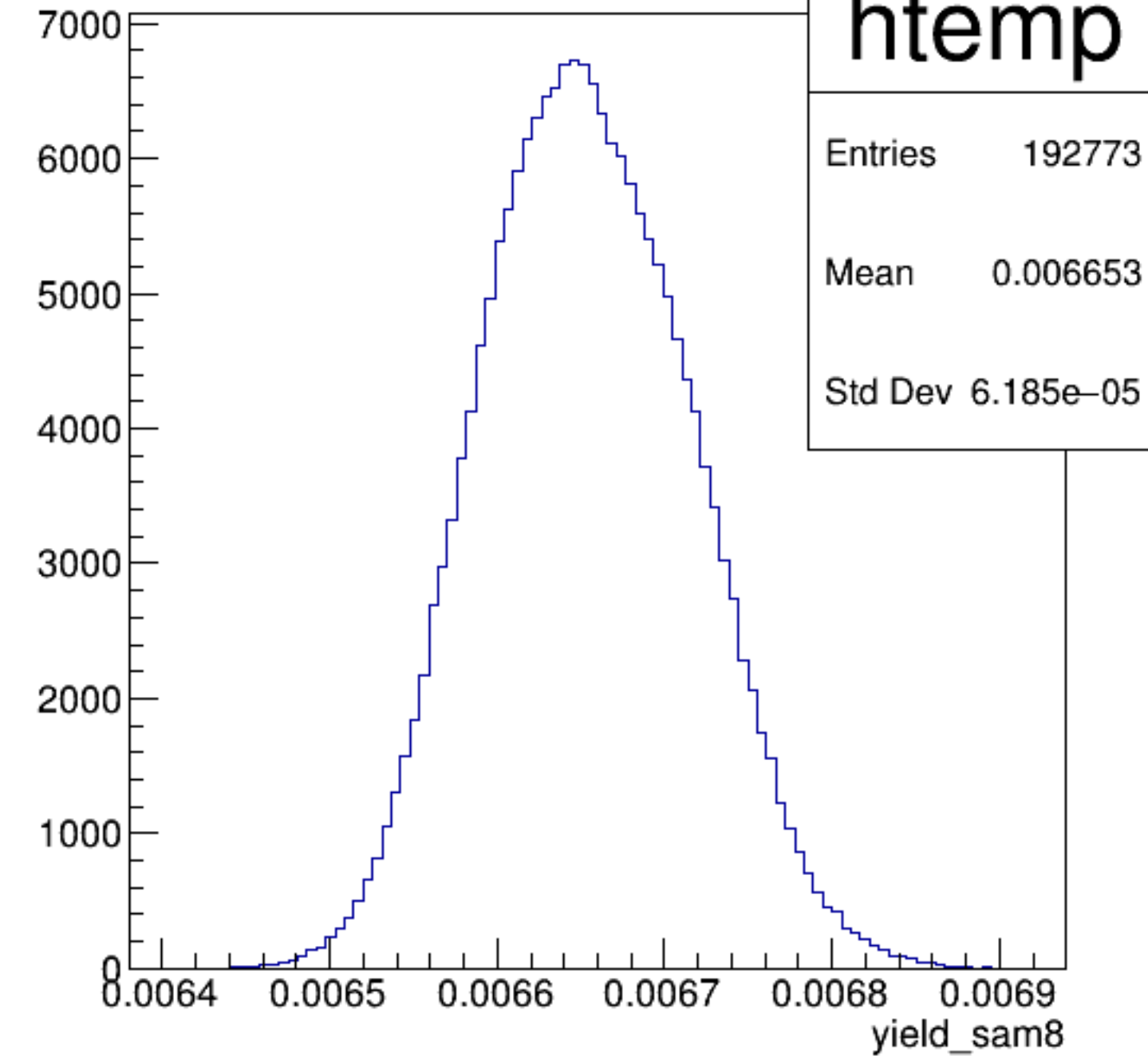
yield_sam8 {ErrorFlag==0}
