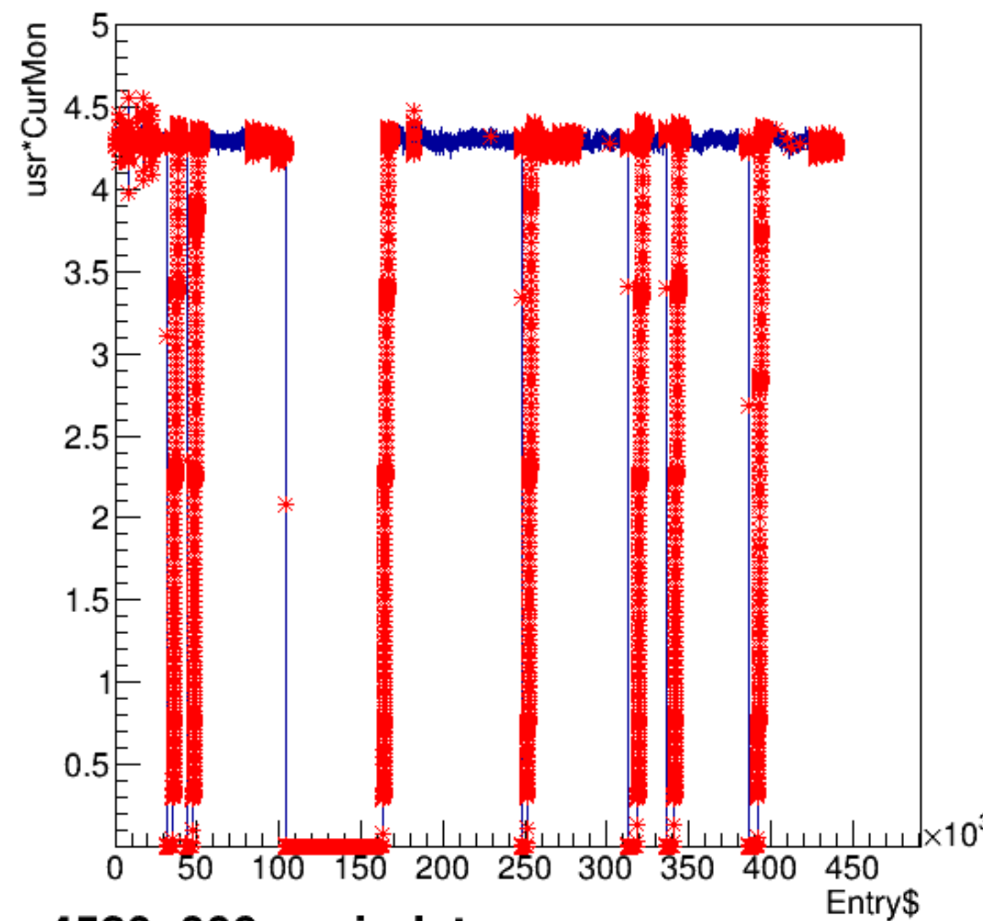
usr*CurMon:Entry$
