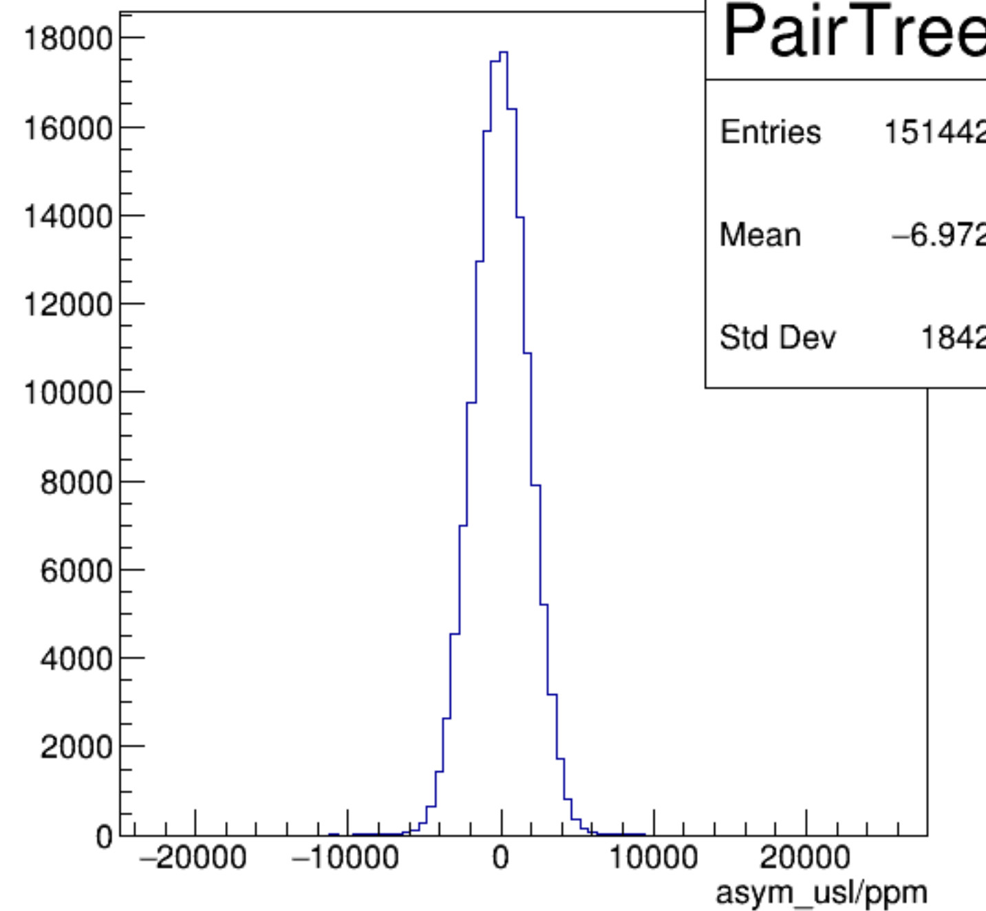
asym_usl/ppm {ErrorFlag==0}
