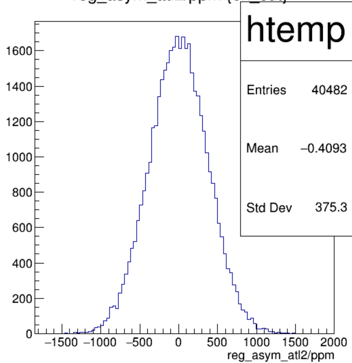
reg_asym_atl2/ppm {ok_cut}
