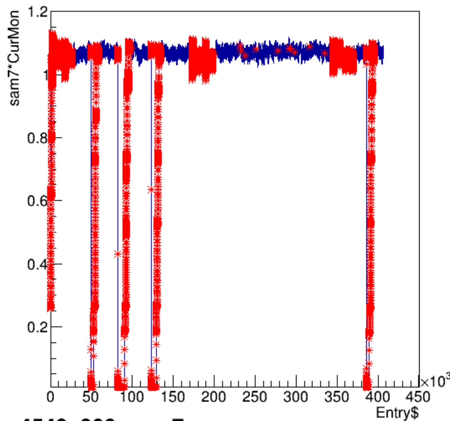
sam7*CurMon:Entry$
