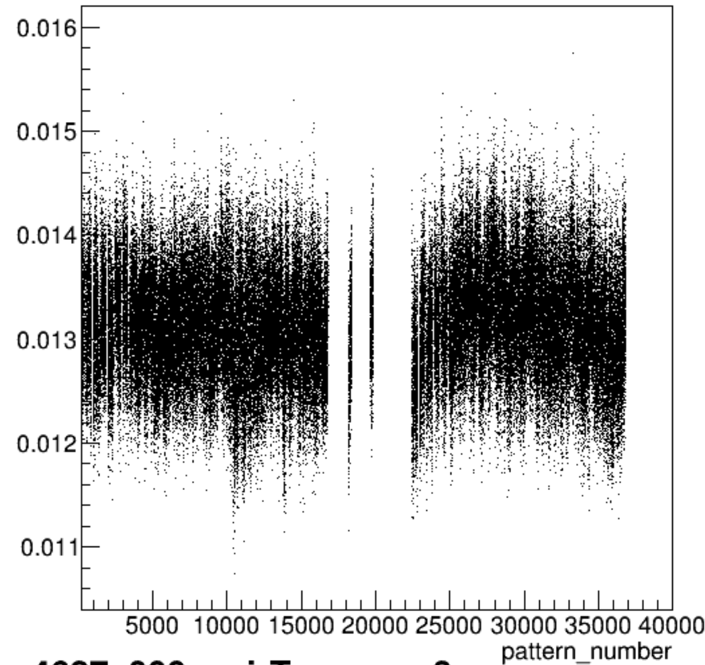
yield_sam3:pattern_number {ErrorFlag==0}
