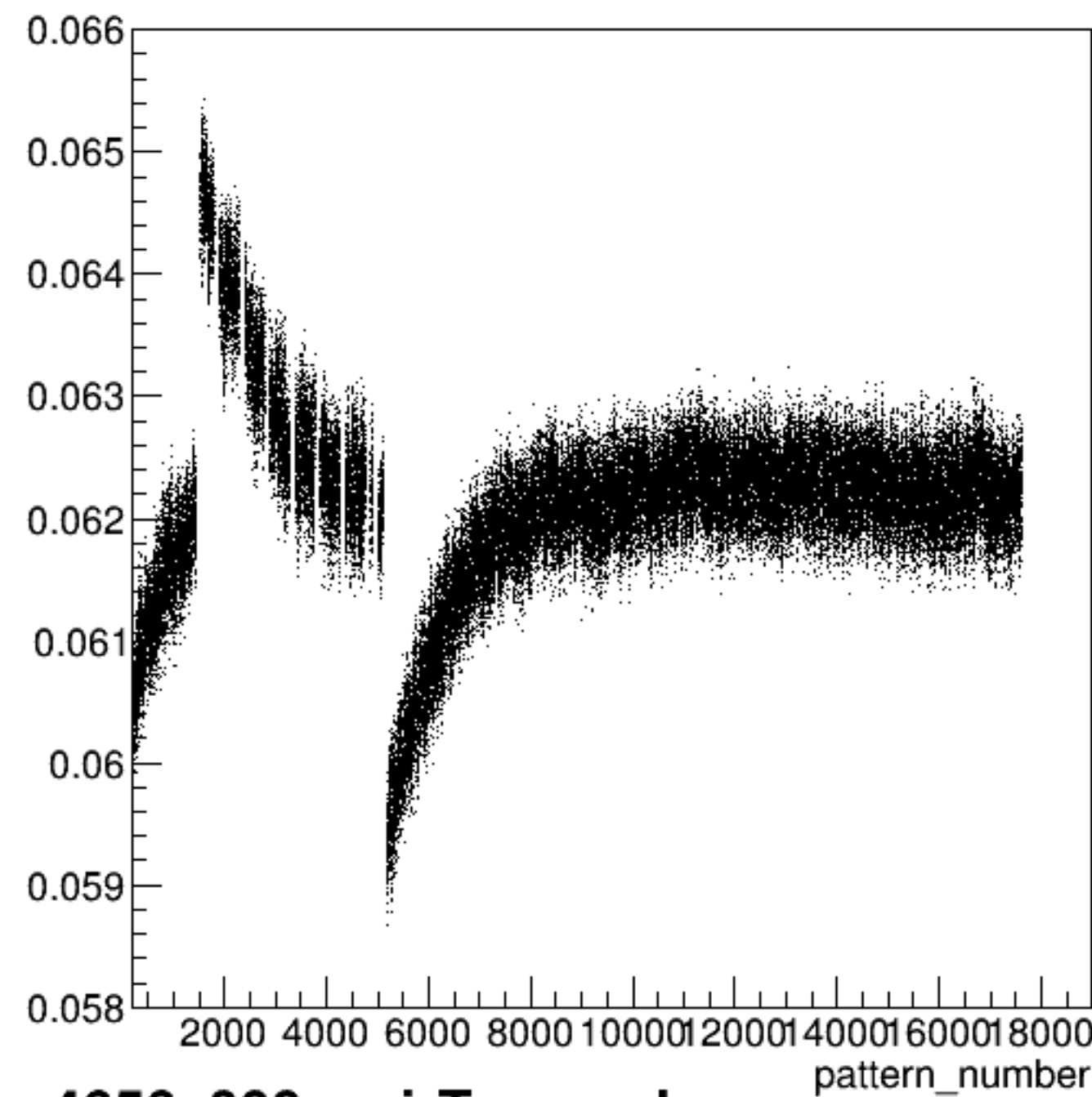
yield_usl:pattern_number {ErrorFlag==0}
