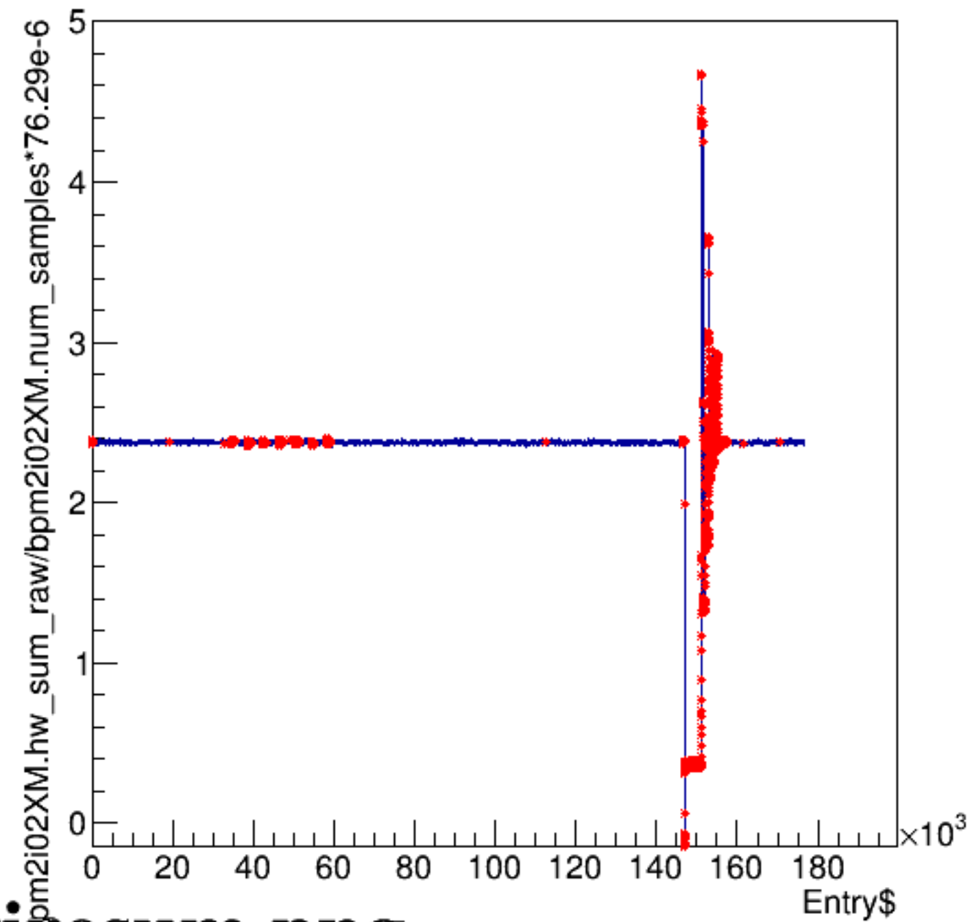
bpm2i02XM.hw_sum_raw/bpm2i02XM.num_samples*76.29e-6:Entry$
