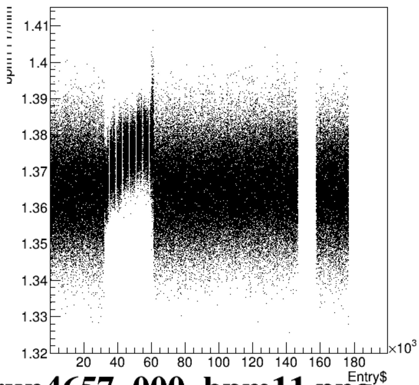
bpm11Y/mm:Entry$ {ErrorFlag==0}
