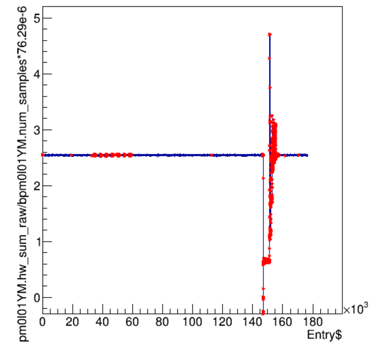
bpm0l01YM.hw_sum_raw/bpm0l01YM.num_samples*76.29e-6:Entry$
