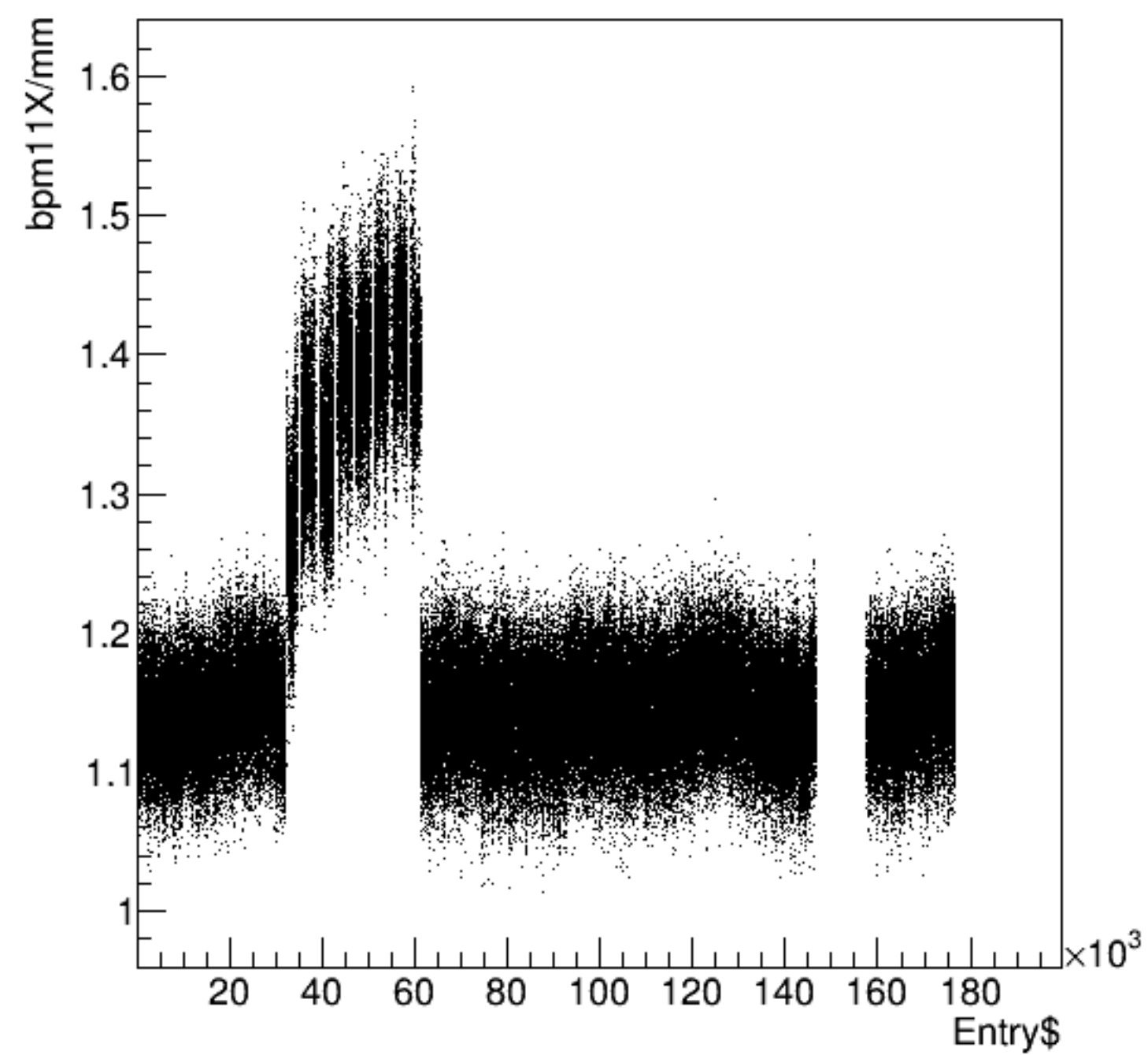
bpm11X/mm:Entry$ {ErrorFlag==0}
