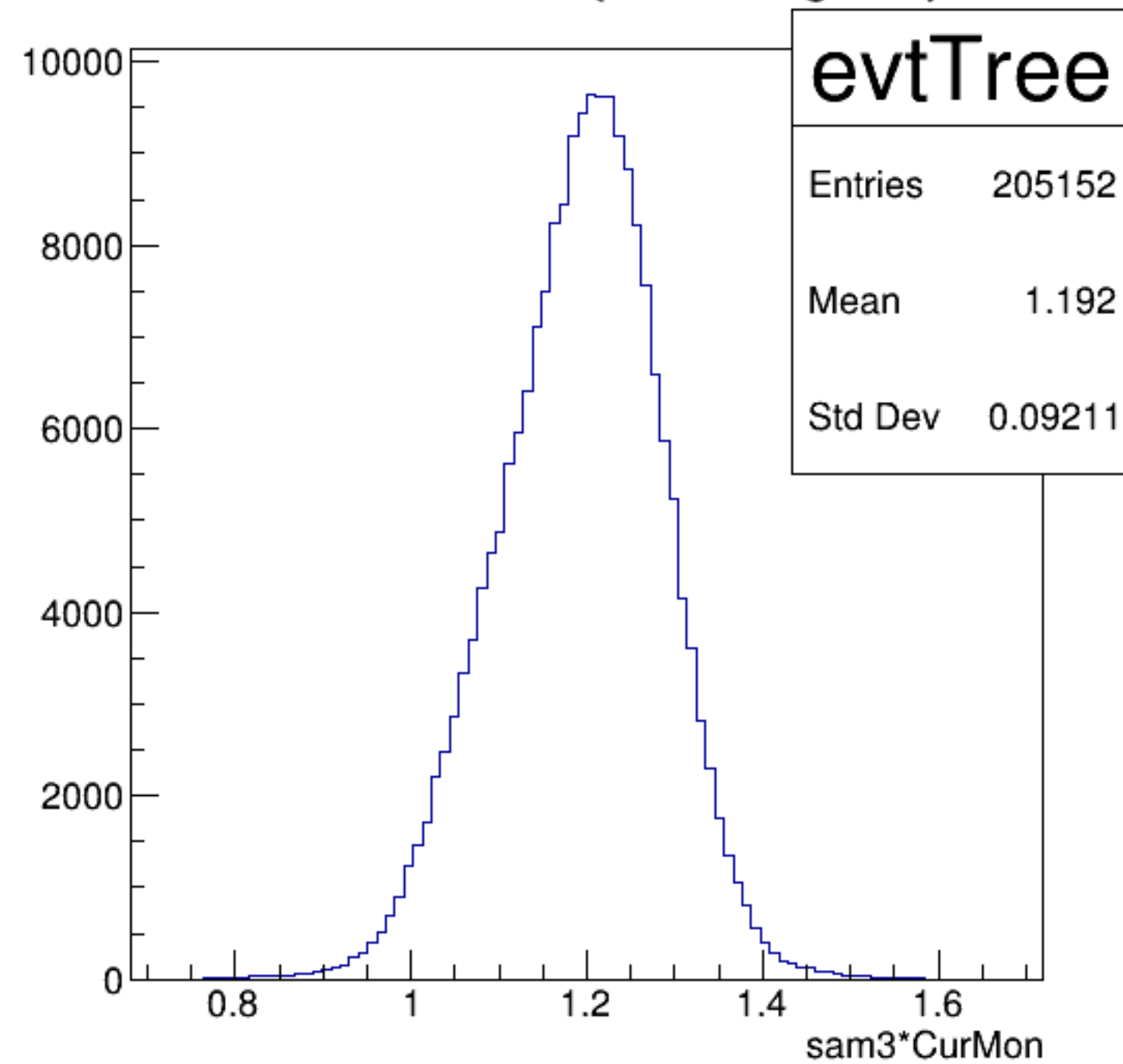
sam3*CurMon {ErrorFlag==0}
