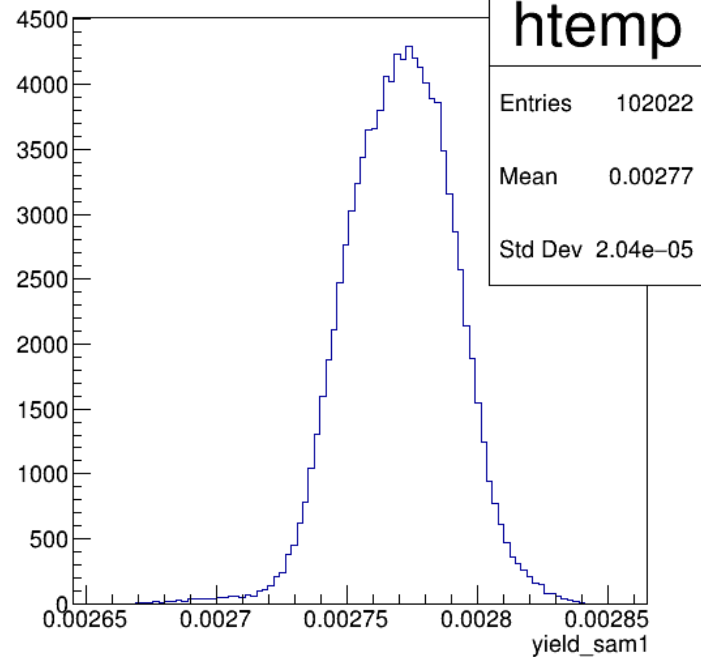
yield_sam1 {ErrorFlag==0}
