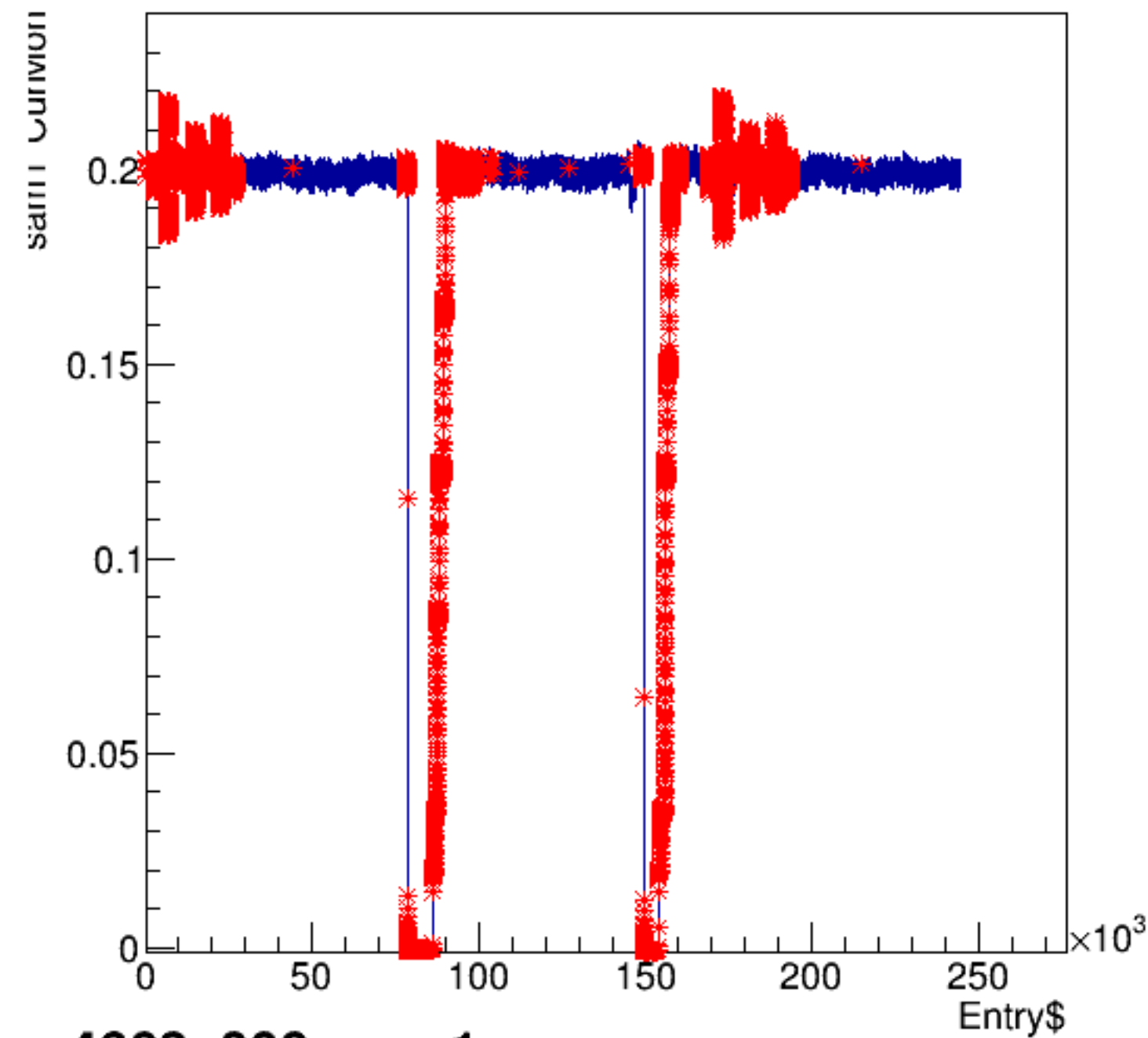
sam1*CurMon:Entry$
