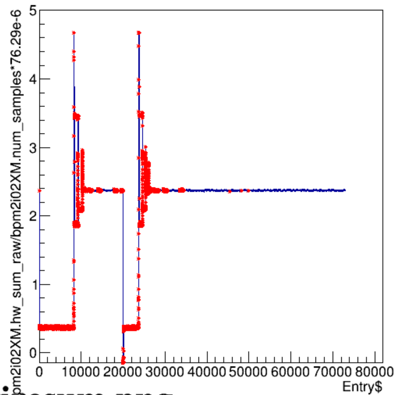
bpm2i02XM.hw_sum_raw/bpm2i02XM.num_samples*76.29e-6:Entry$
