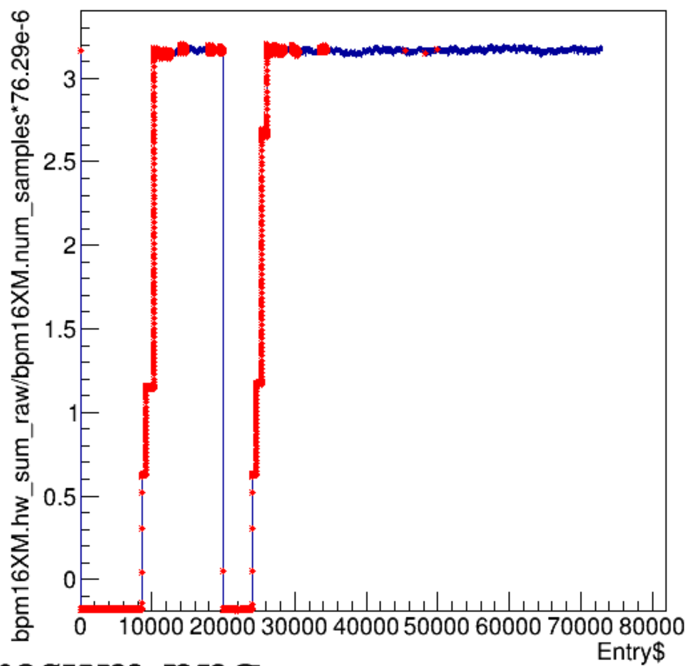
bpm16XM.hw_sum_raw/bpm16XM.num_samples*76.29e-6:Entry$
