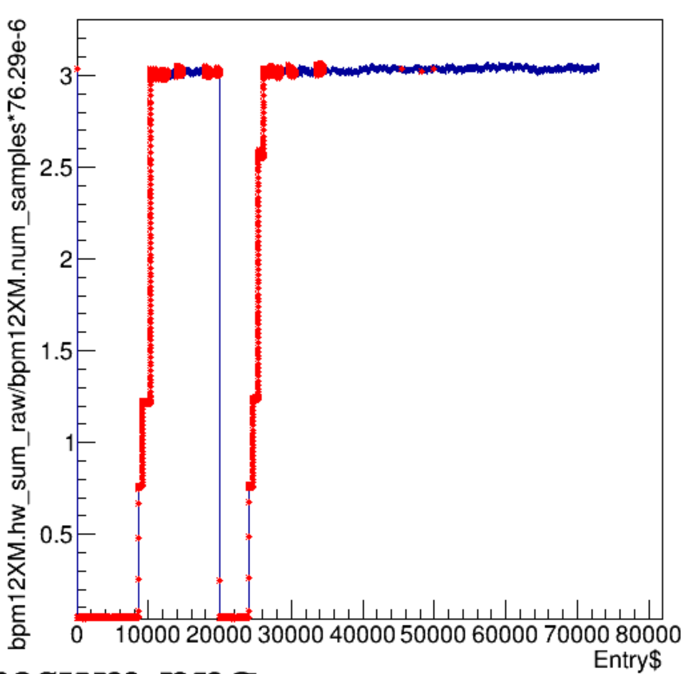
bpm12XM.hw_sum_raw/bpm12XM.num_samples*76.29e-6:Entry$
