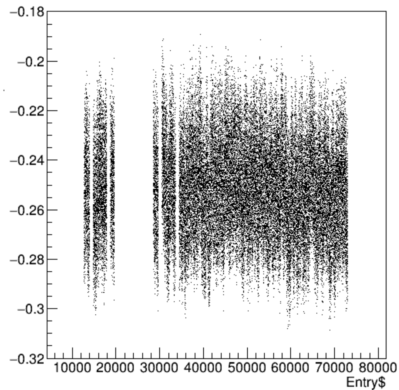
bpm0i02X/mm:Entry$ {ErrorFlag==0}
