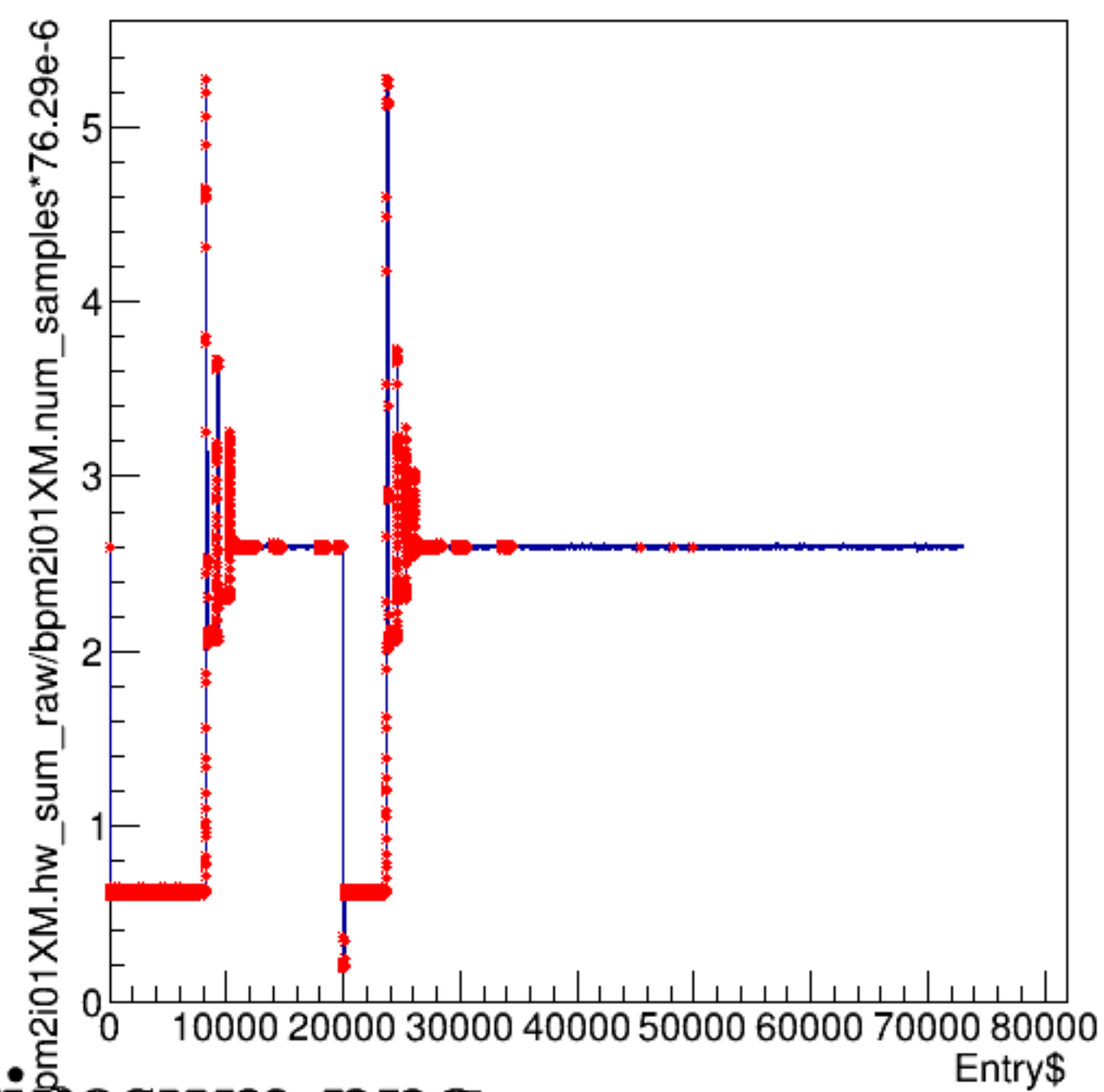
bpm2i01XM.hw_sum_raw/bpm2i01XM.num_samples*76.29e-6:Entry$
