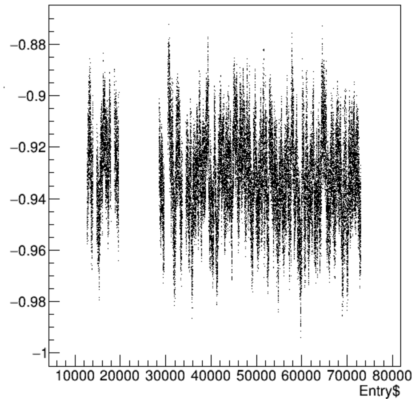
bpm1i02X/mm:Entry$ {ErrorFlag==0}
