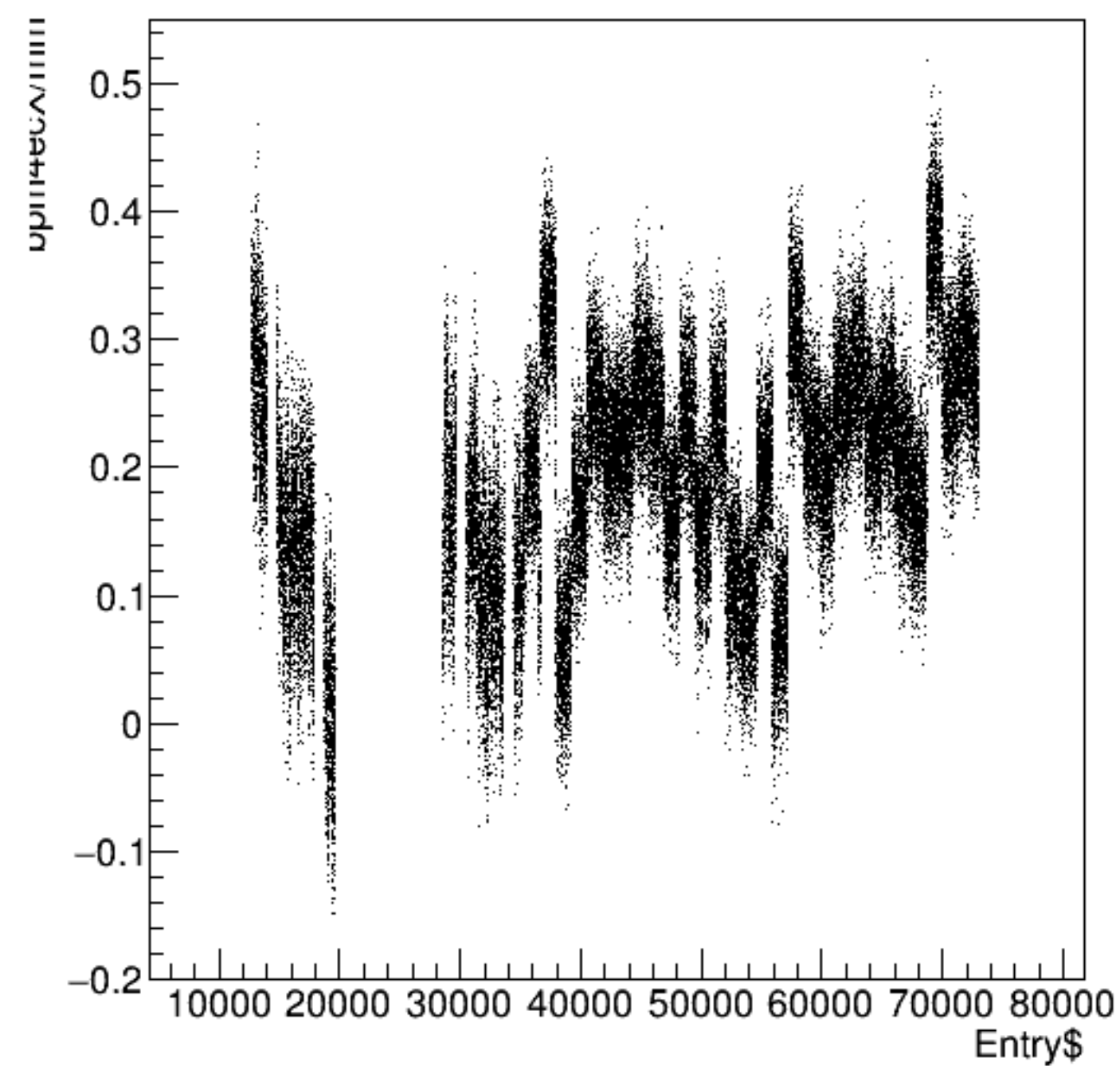
bpm4ecX/mm:Entry$ {ErrorFlag==0}
