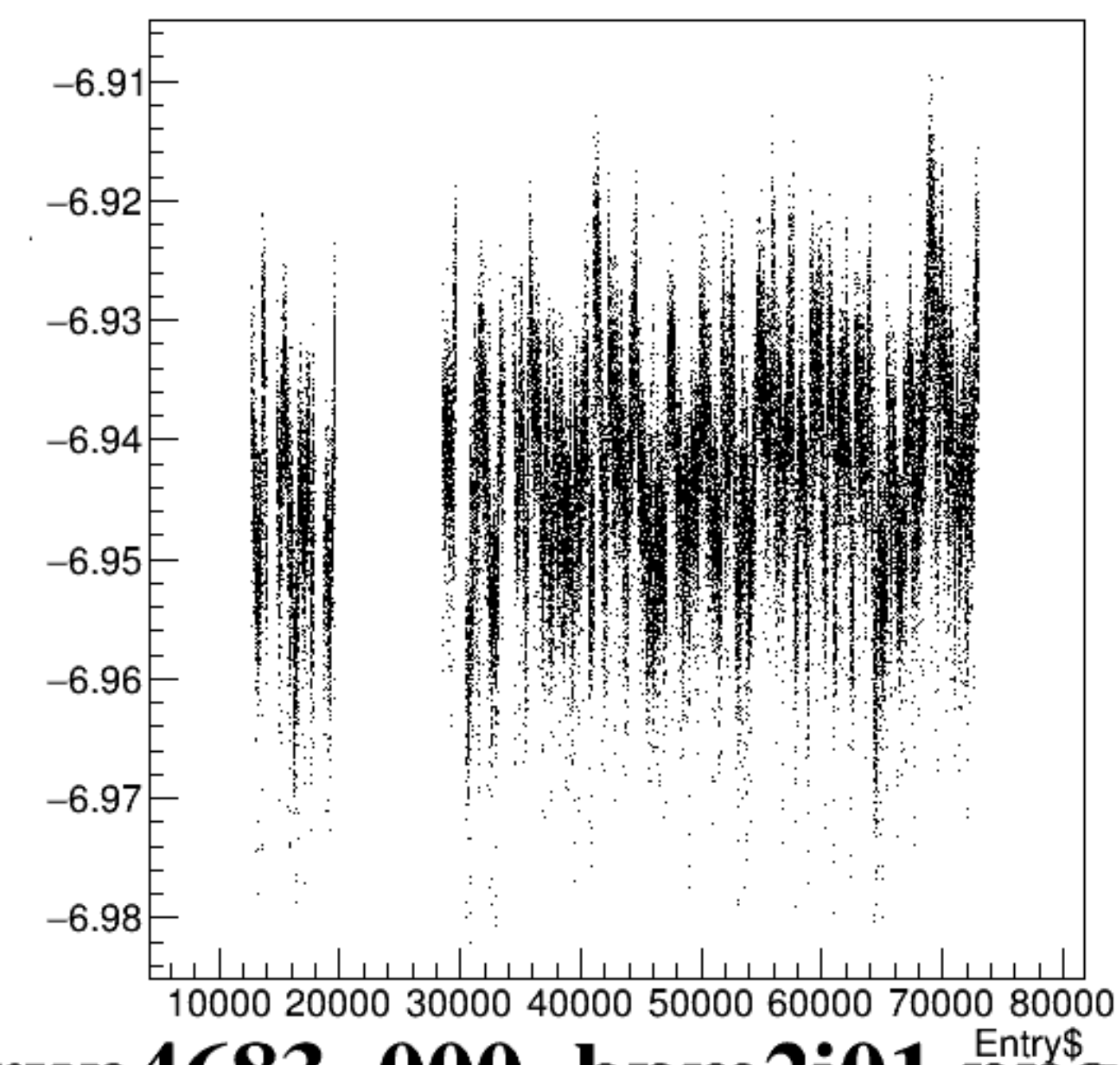
bpm2i01Y/mm:Entry$ {ErrorFlag==0}
