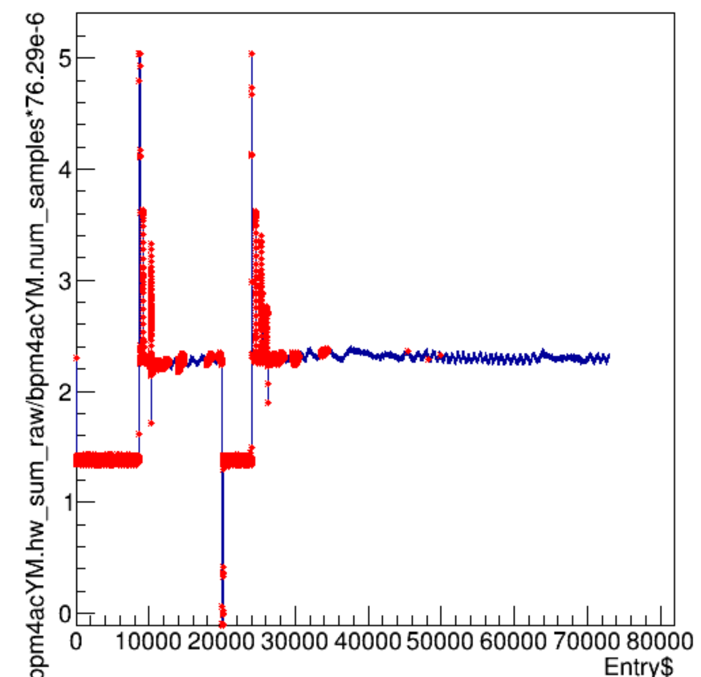
bpm4acYM.hw_sum_raw/bpm4acYM.num_samples*76.29e-6:Entry$
