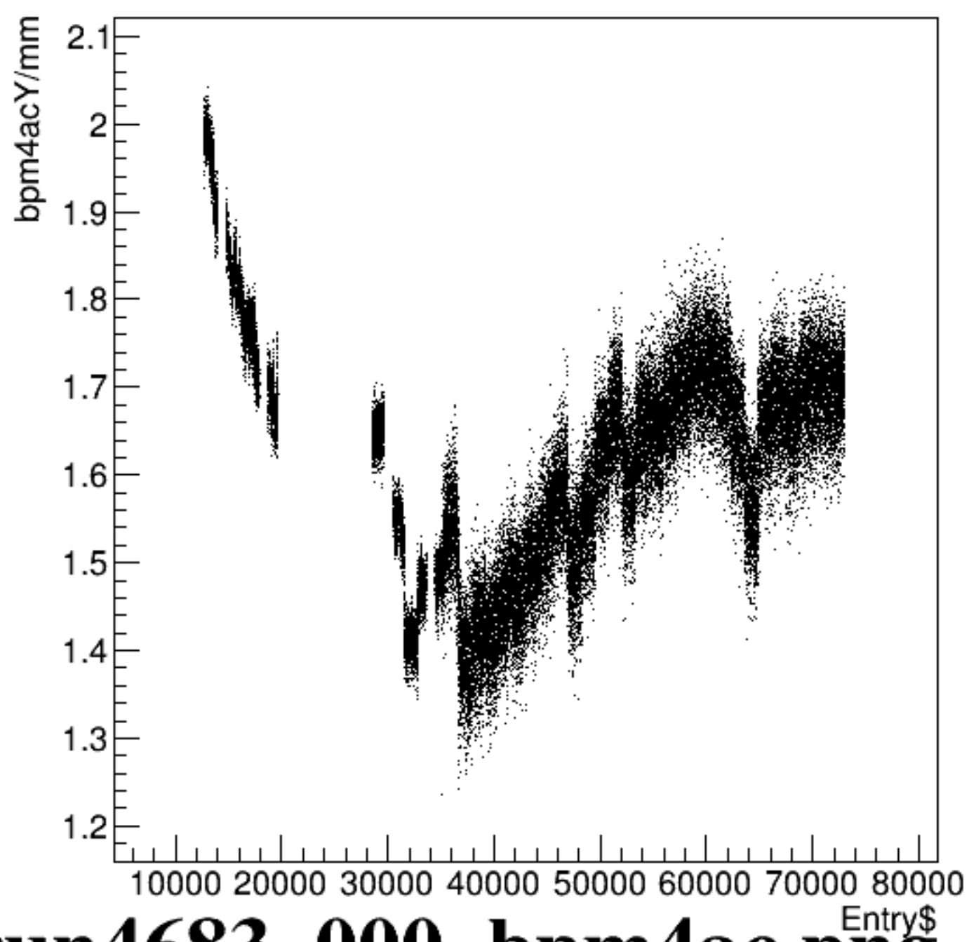
bpm4acY/mm:Entry$ {ErrorFlag==0}
