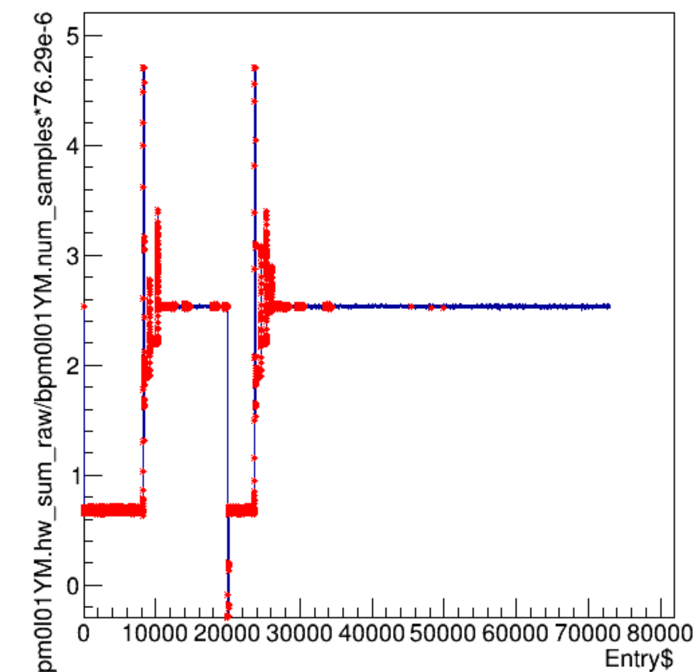
bpm0l01YM.hw_sum_raw/bpm0l01YM.num_samples*76.29e-6:Entry$
