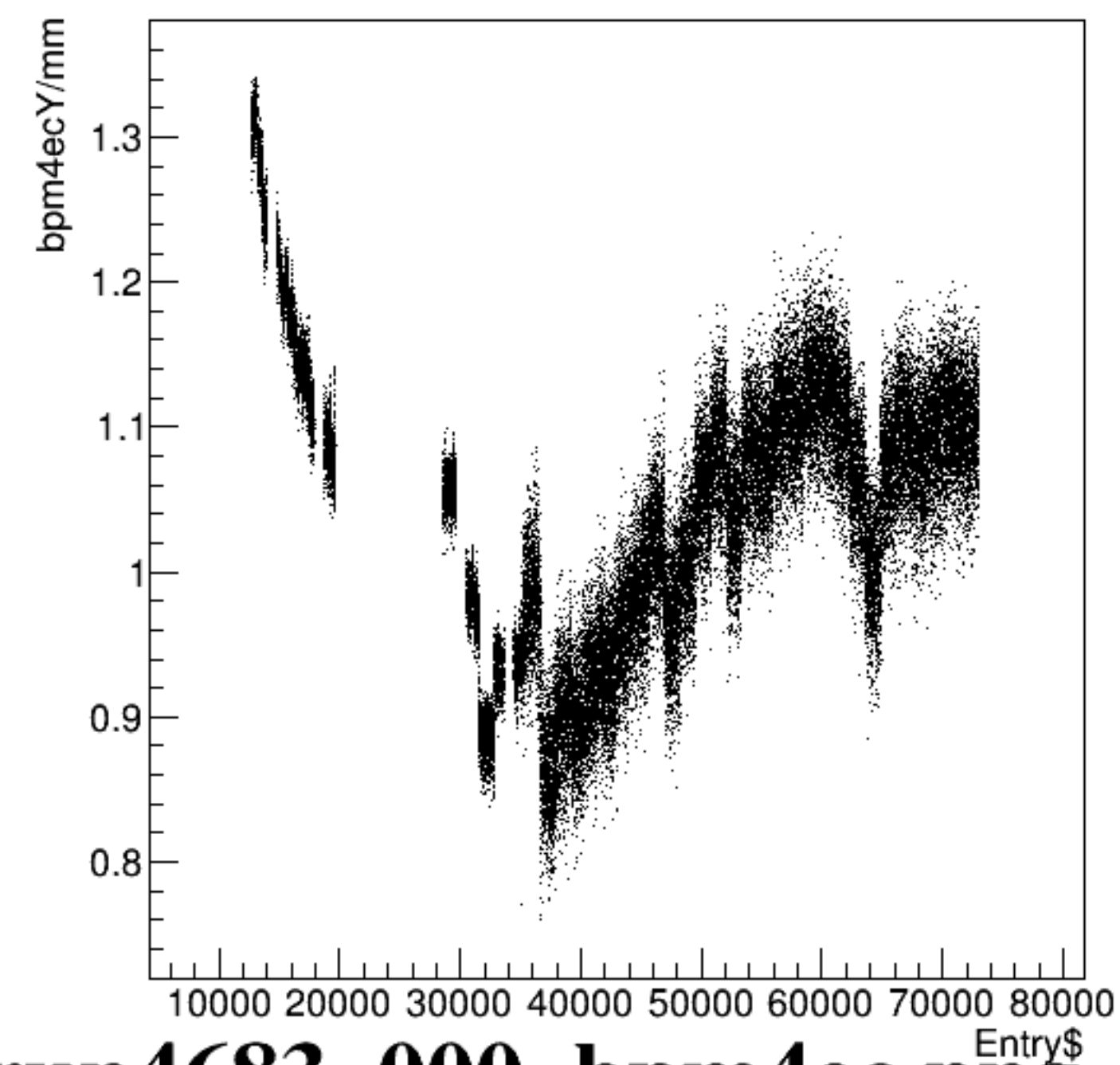
bpm4ecY/mm:Entry$ {ErrorFlag==0}
