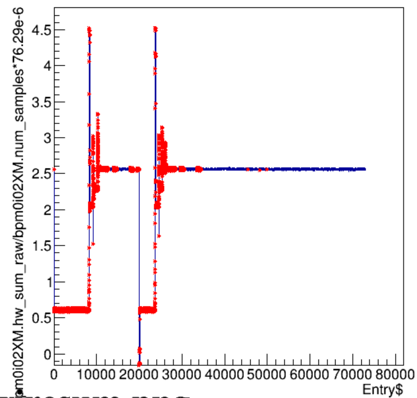
bpm0i02XM.hw_sum_raw/bpm0i02XM.num_samples*76.29e-6:Entry$
