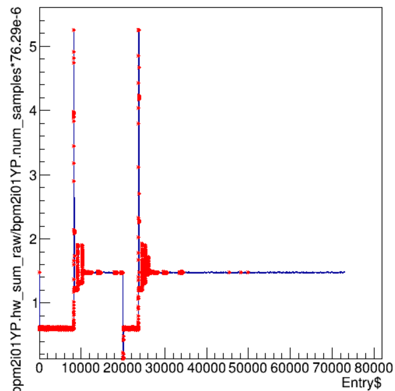
bpm2i01YP.hw_sum_raw/bpm2i01YP.num_samples*76.29e-6:Entry$
