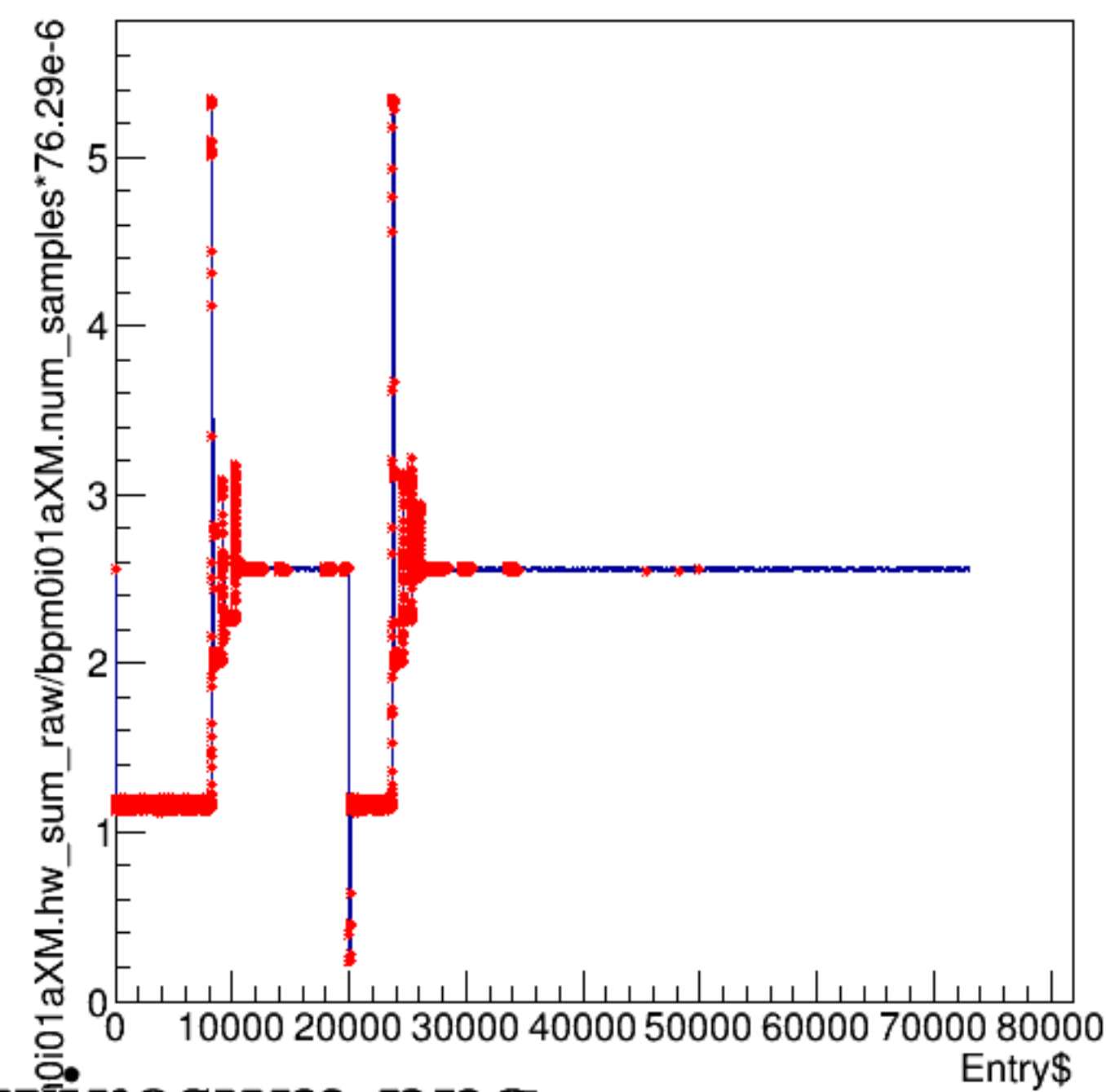
bpm0i01aXM.hw_sum_raw/bpm0i01aXM.num_samples*76.29e-6:Entry$
