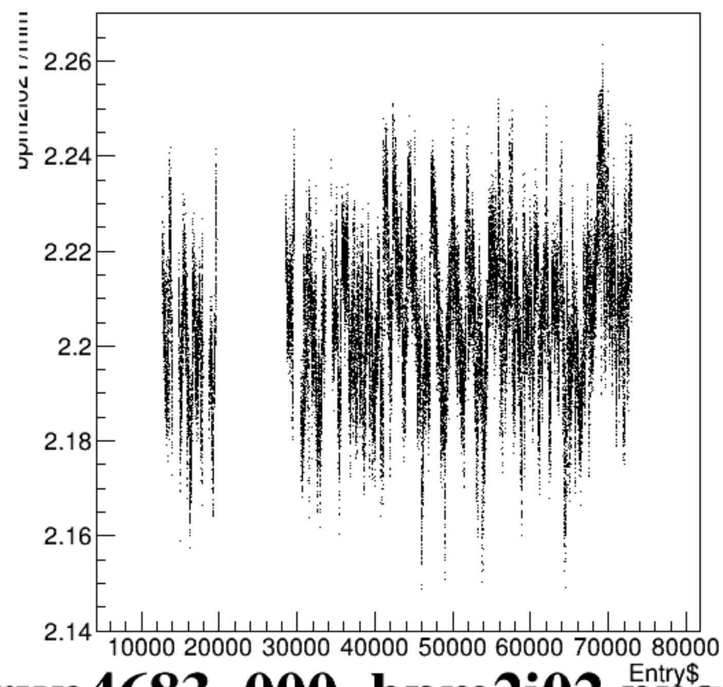
bpm2i02Y/mm:Entry$ {ErrorFlag==0}
