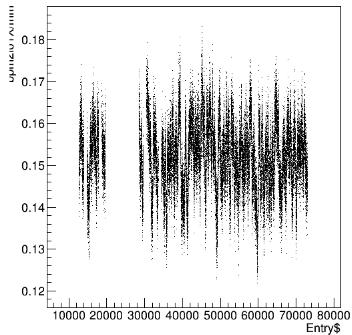
bpm2i01X/mm:Entry$ {ErrorFlag==0}
