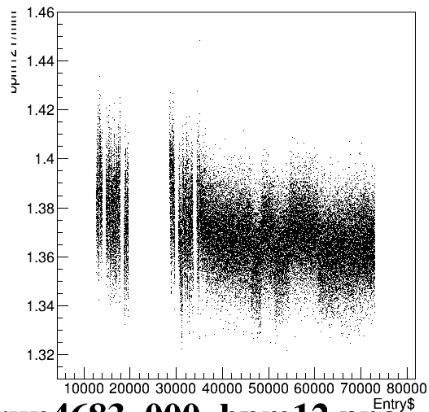
bpm12Y/mm:Entry$ {ErrorFlag==0}
