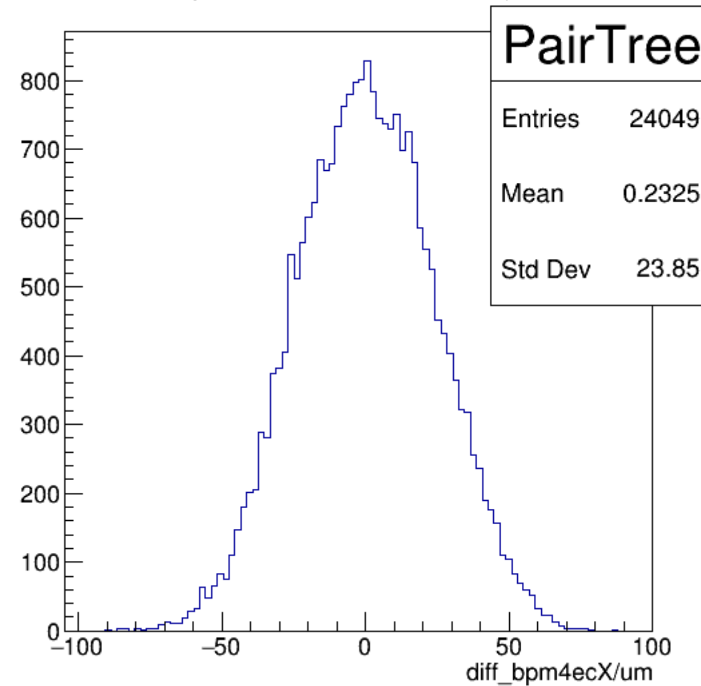
diff_bpm4ecX/um {ErrorFlag==0}
