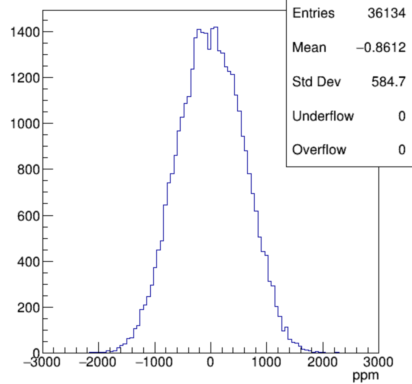
asym_usl
