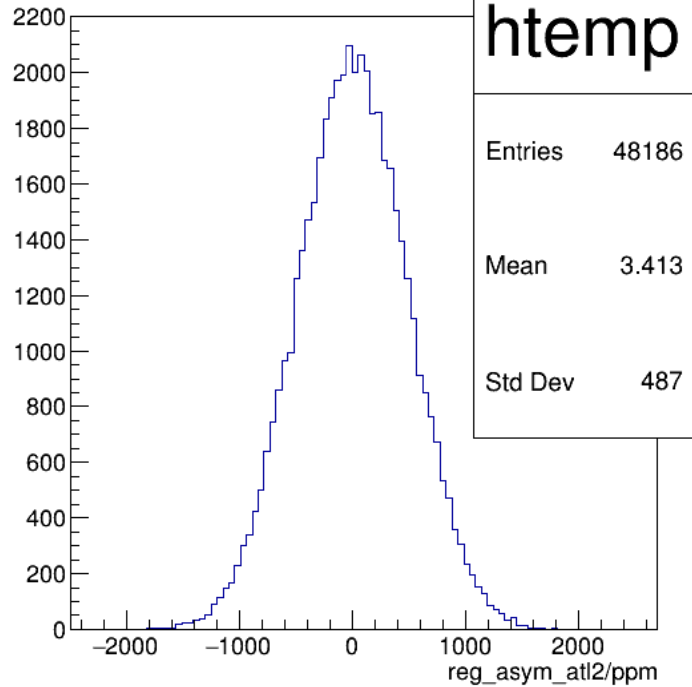
reg_asym_atl2/ppm {ok_cut}
