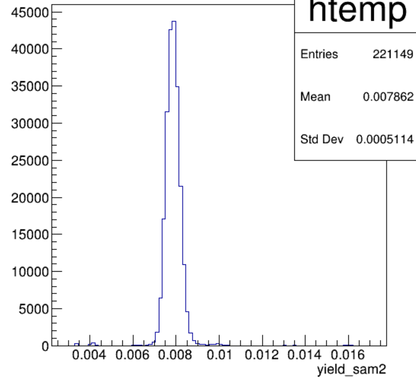
yield_sam2 {ErrorFlag==0}
