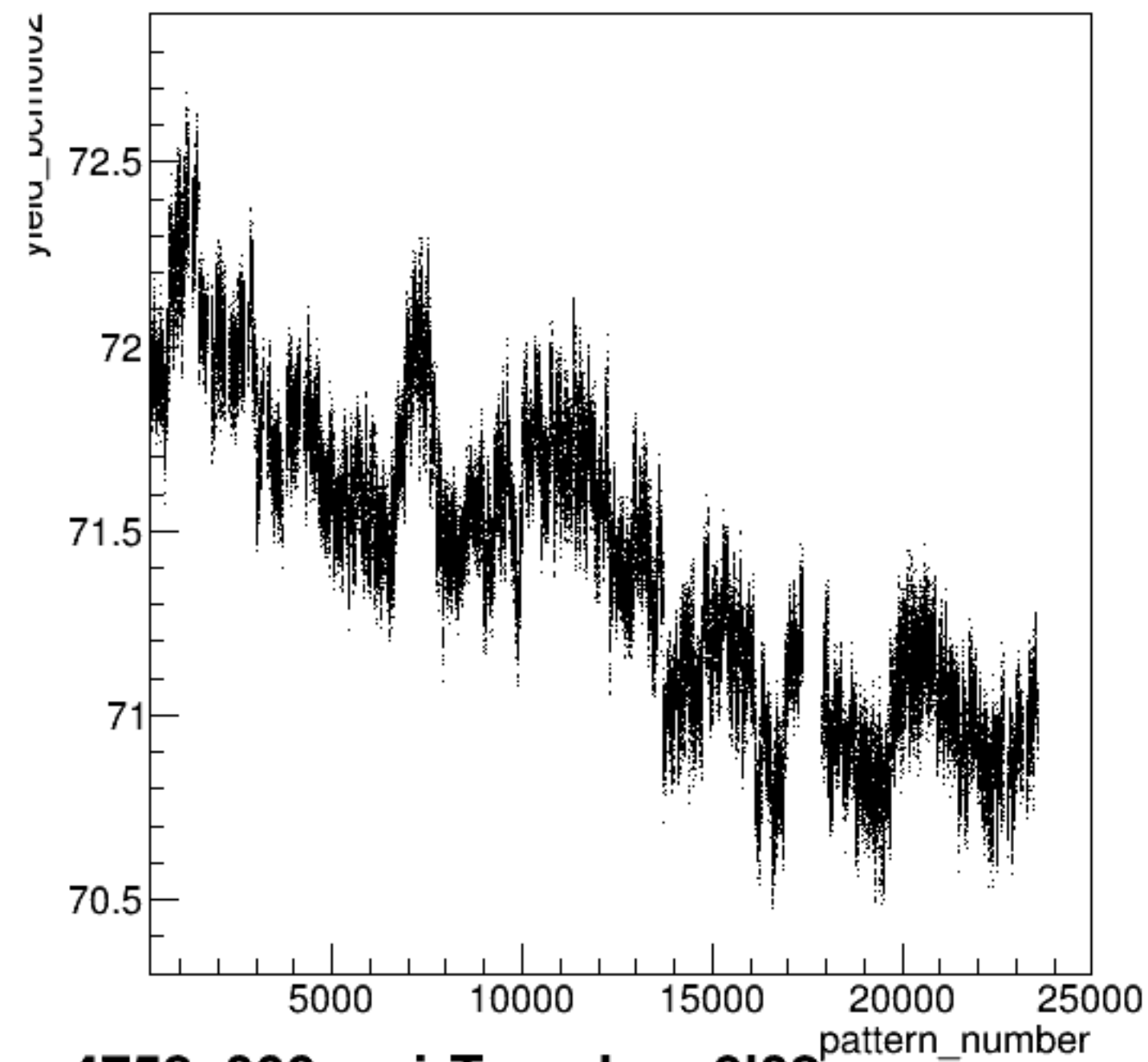
run4752_000_pairTree_bcm0l02.png
