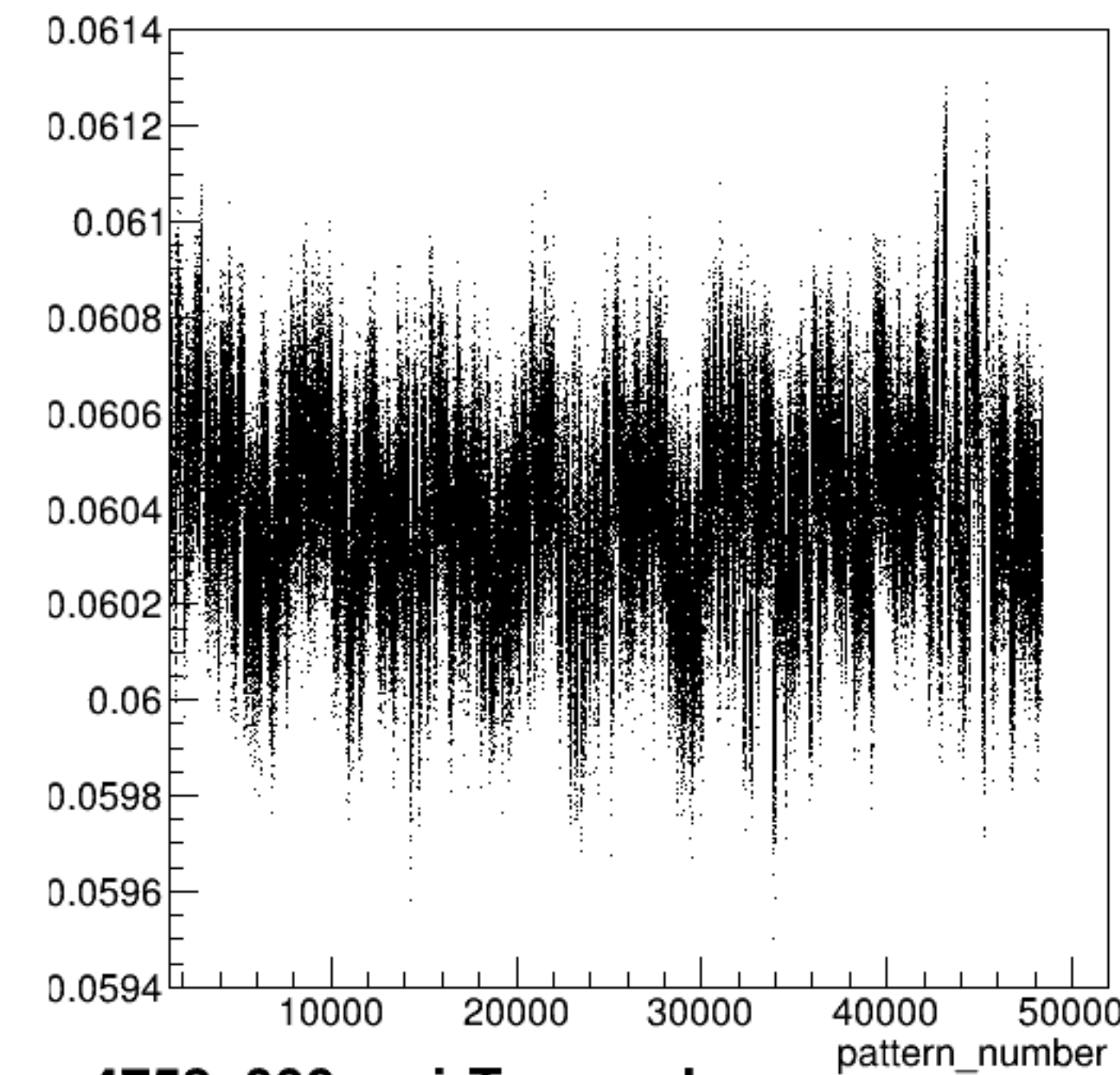
yield_usl:pattern_number {ErrorFlag==0}
