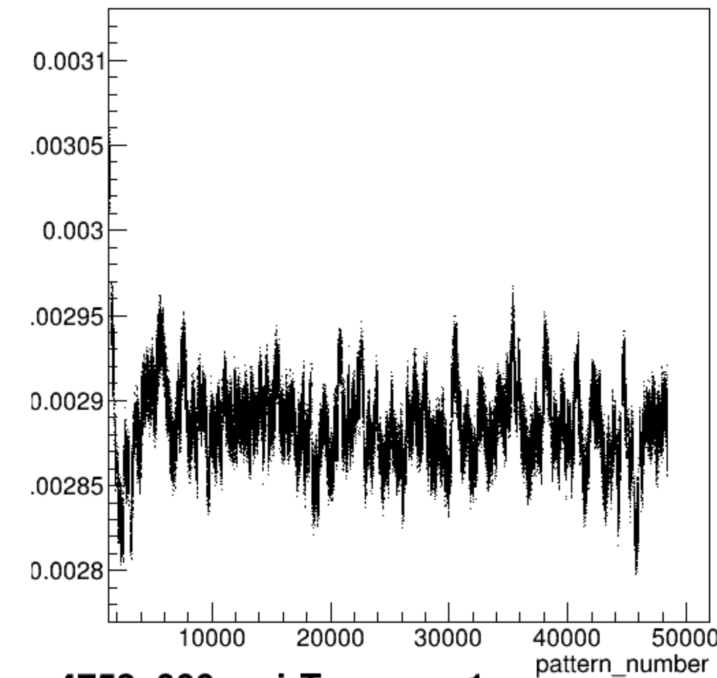
yield_sam1:pattern_number {ErrorFlag==0}
