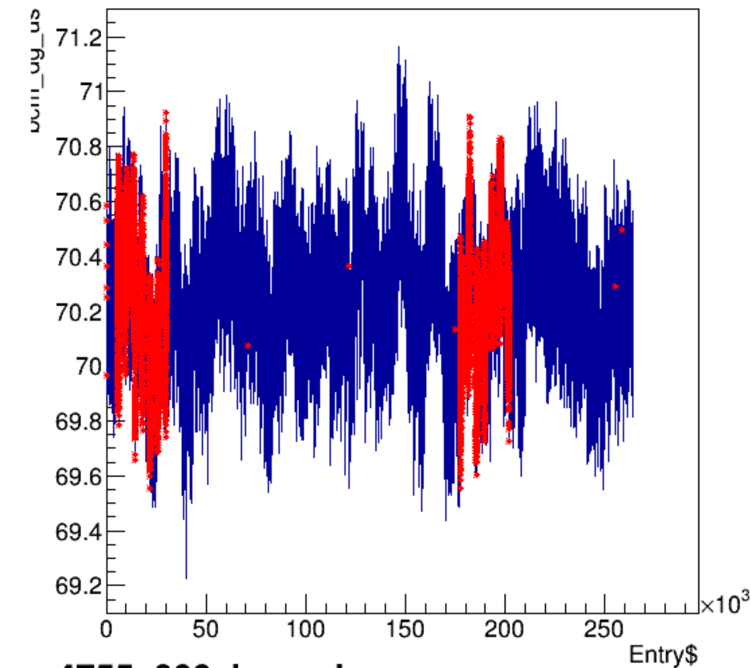
bcm_dg_us:Entry$
