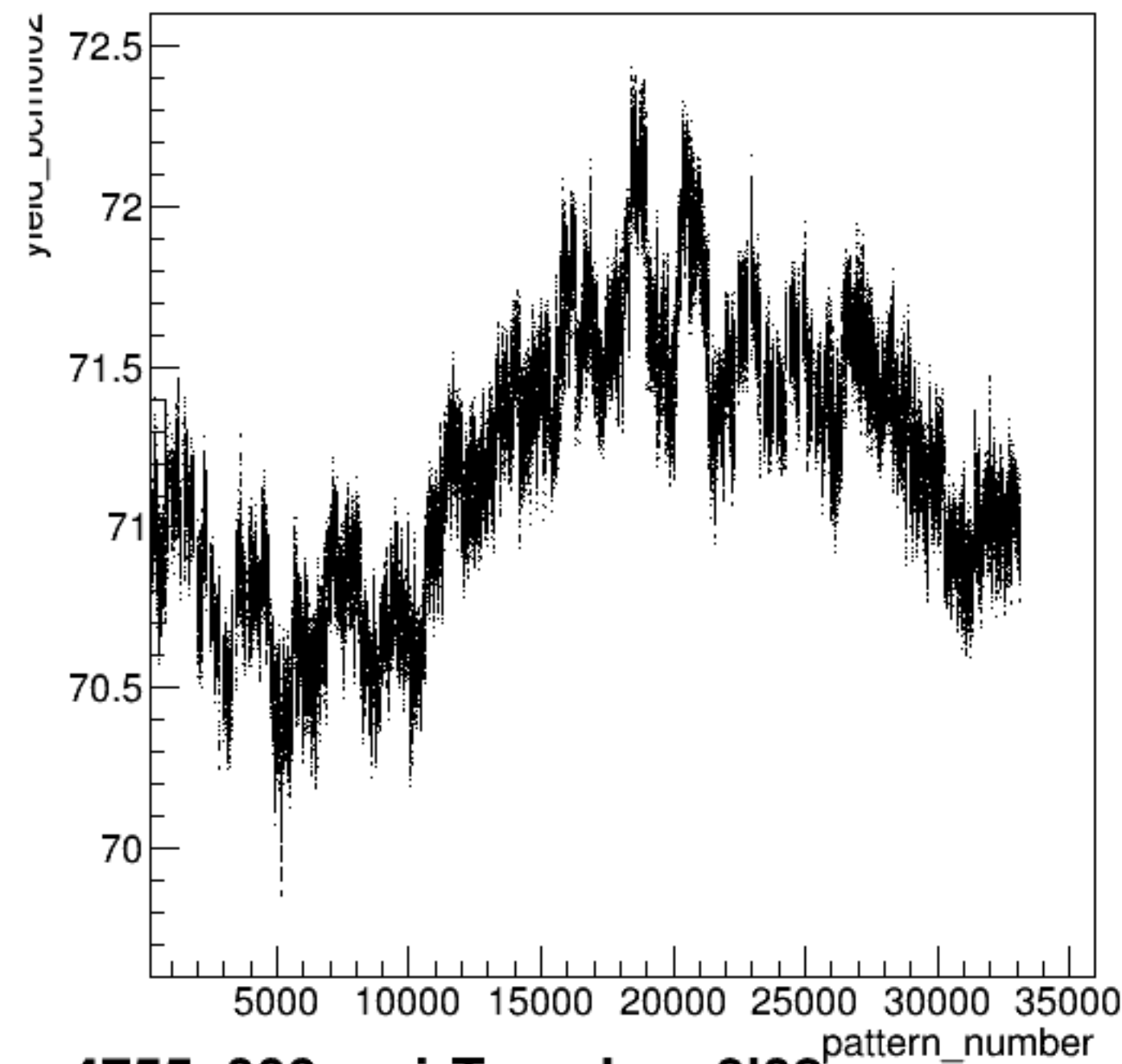
run4755_000_pairTree_bcm0l02.png
