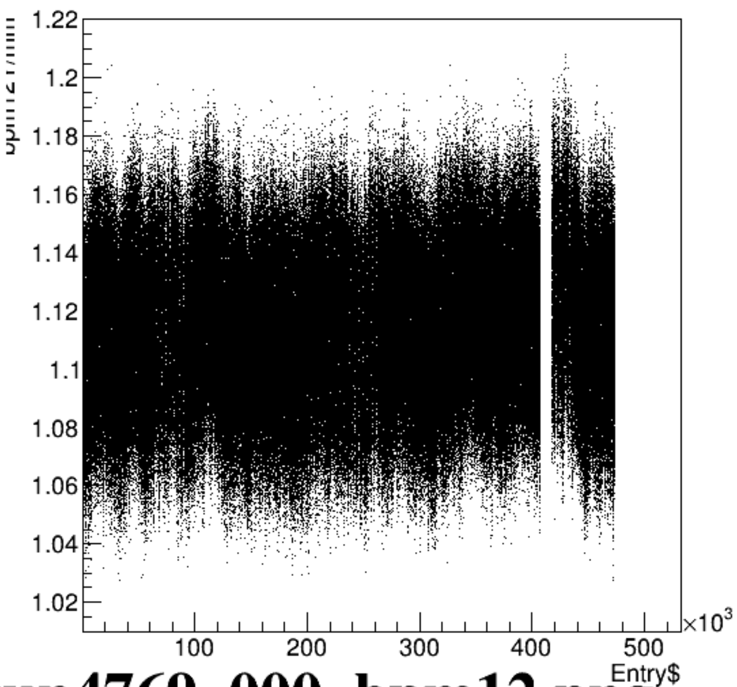
bpm12Y/mm:Entry$ {ErrorFlag==0}
