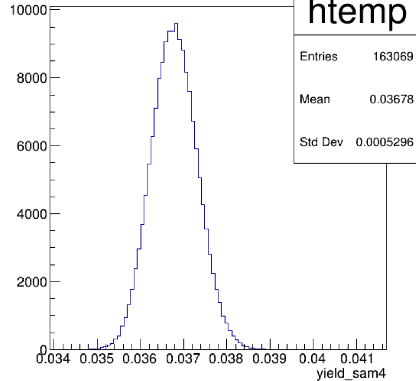
yield_sam4 {ErrorFlag==0}
