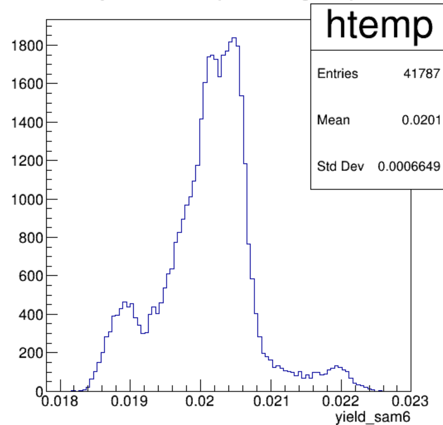
yield_sam6 {ErrorFlag==0}
