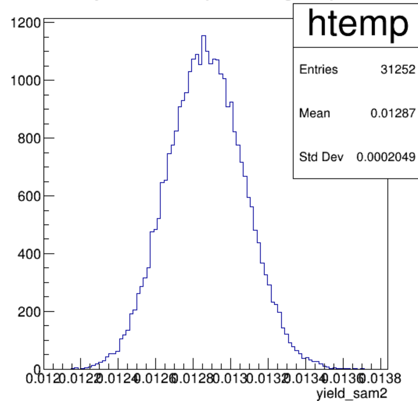
yield_sam2 {ErrorFlag==0}
