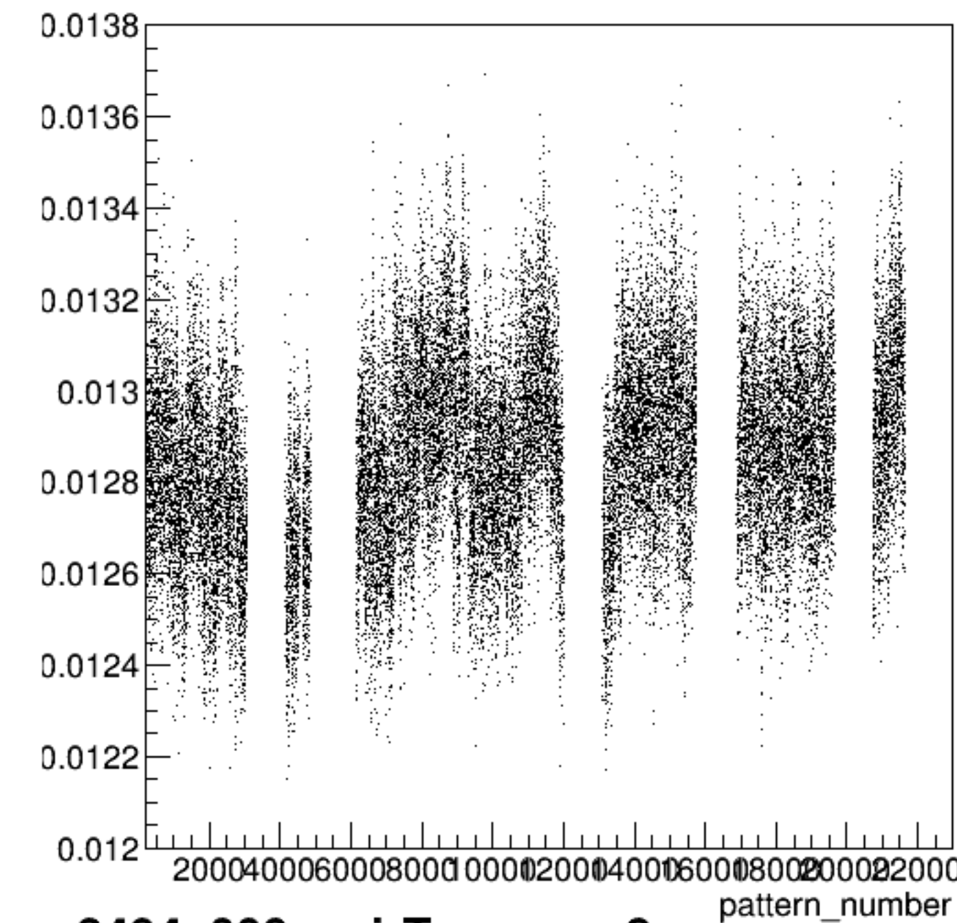
yield_sam2:pattern_number {ErrorFlag==0}
