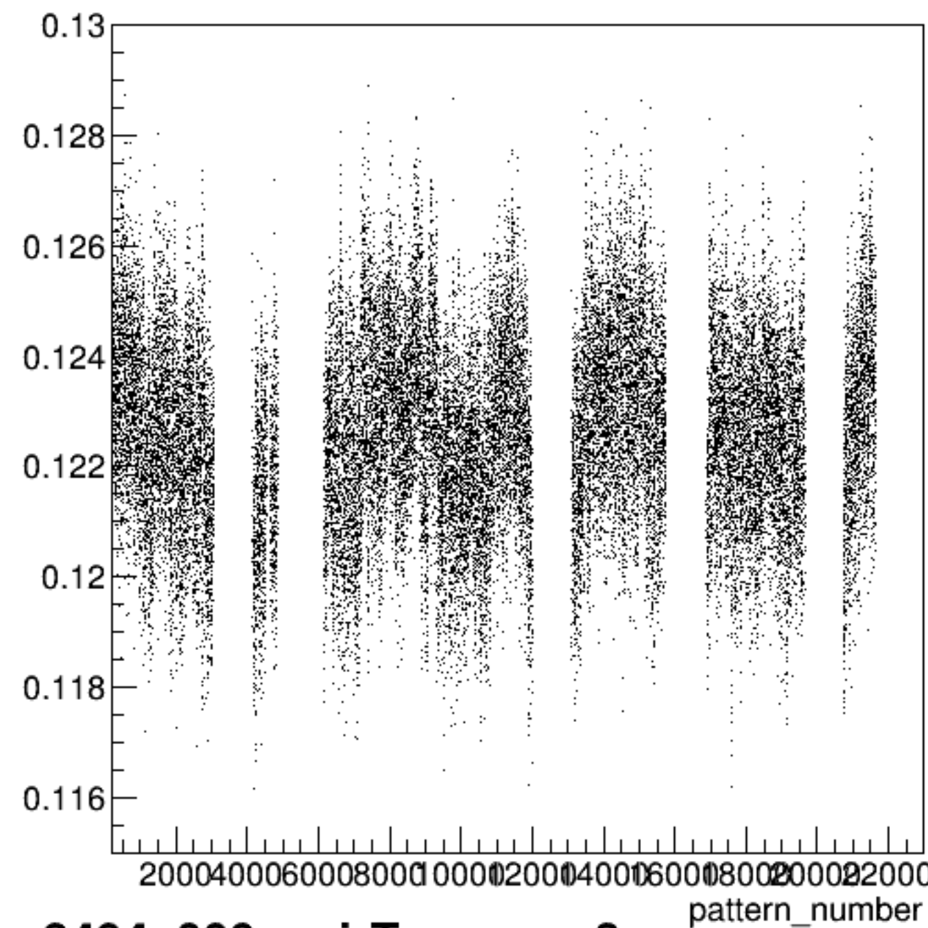
yield_sam3:pattern_number {ErrorFlag==0}
