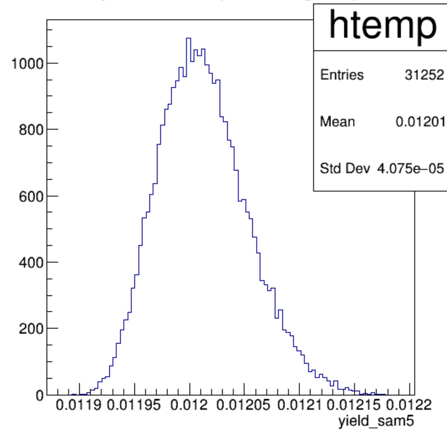
yield_sam5 {ErrorFlag==0}
