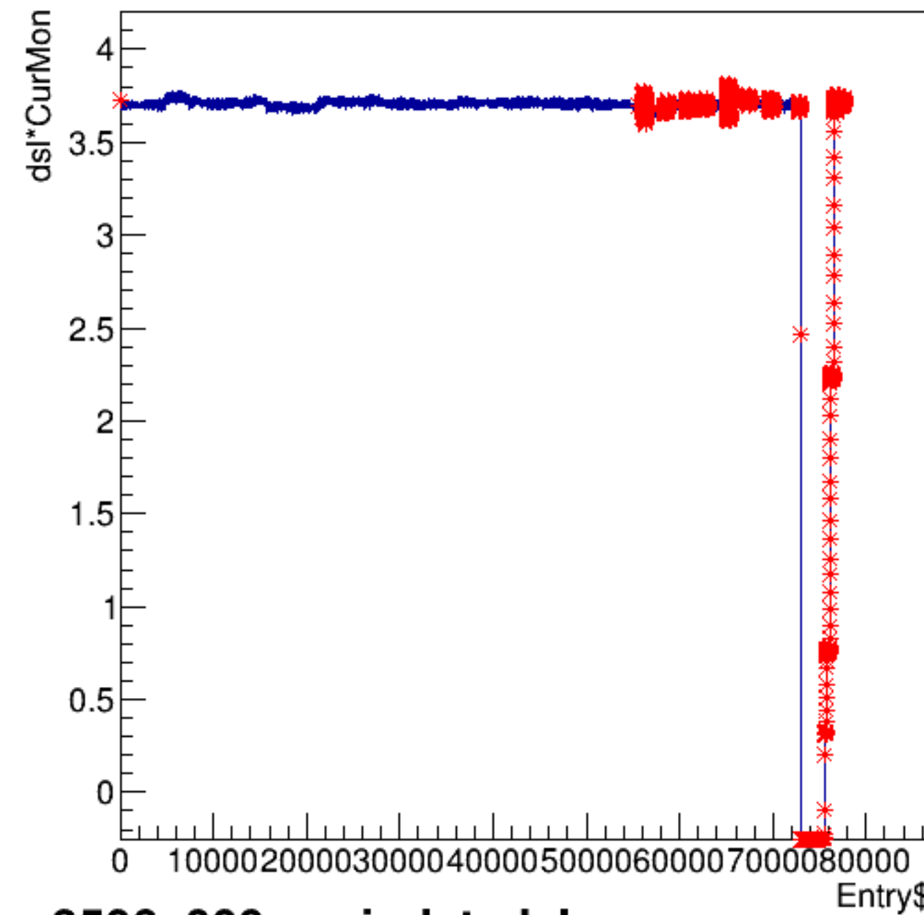
dsl*CurMon:Entry$
