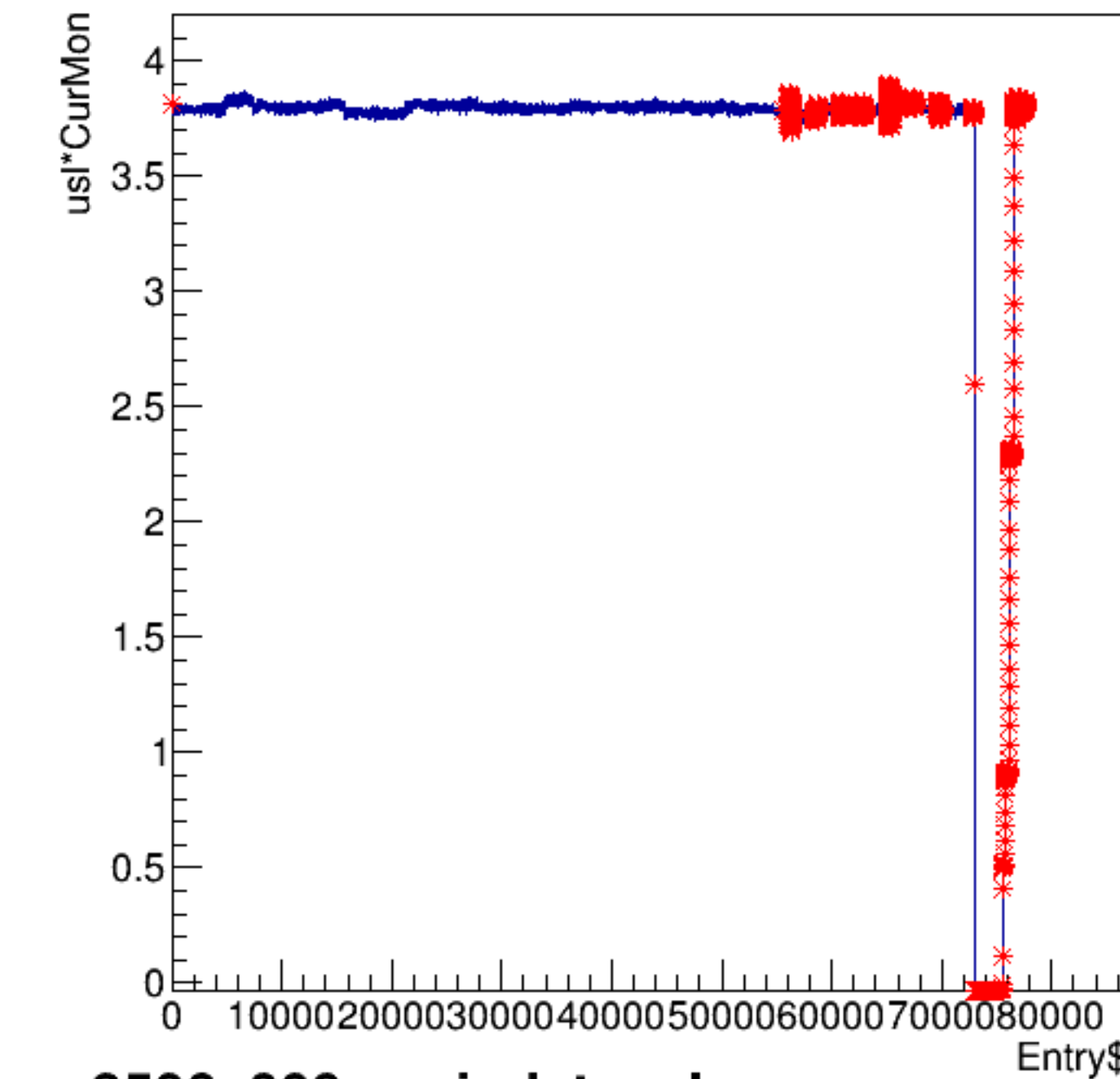
usl*CurMon:Entry$
