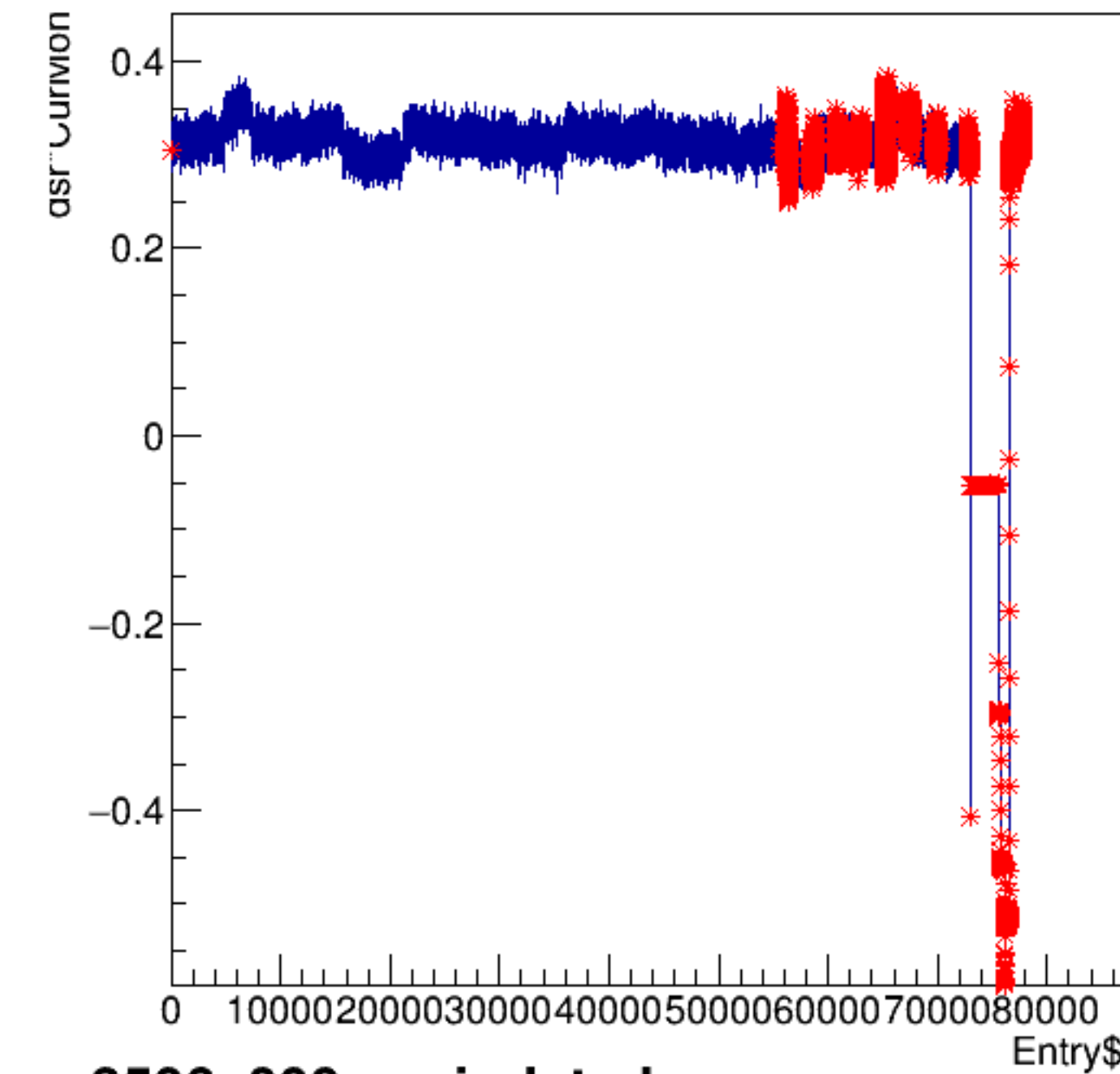
dsr*CurMon:Entry$
