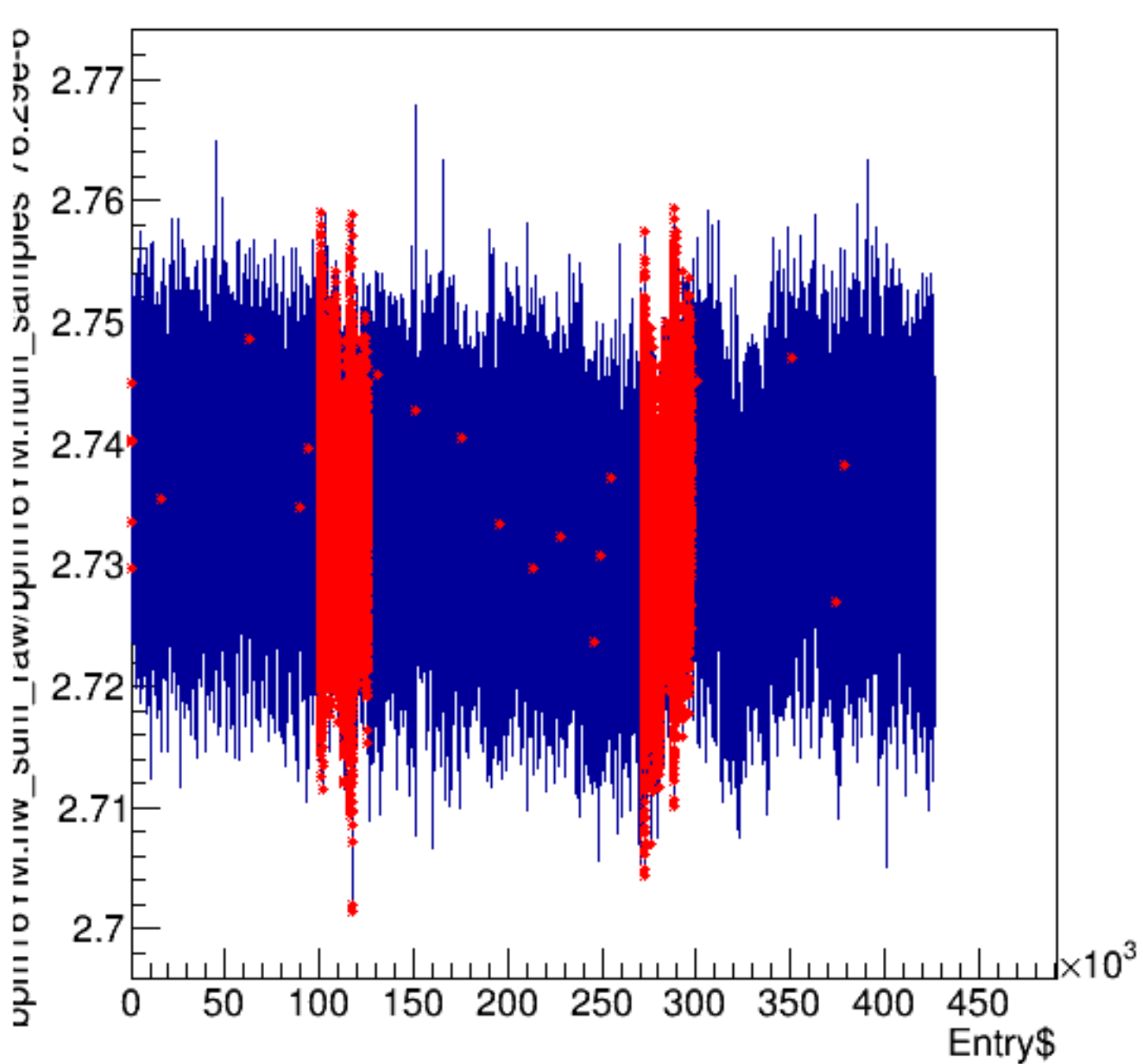
bpm16YM.hw_sum_raw/bpm16YM.num_samples*76.29e-6:Entry$
