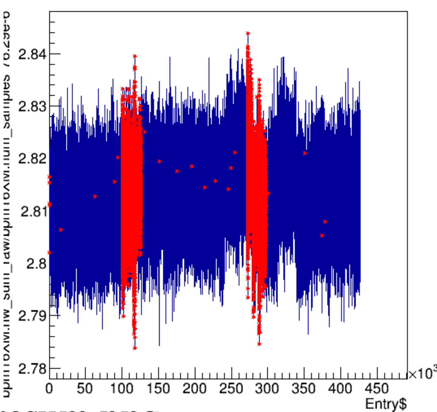
bpm16XM.hw_sum_raw/bpm16XM.num_samples*76.29e-6:Entry$
