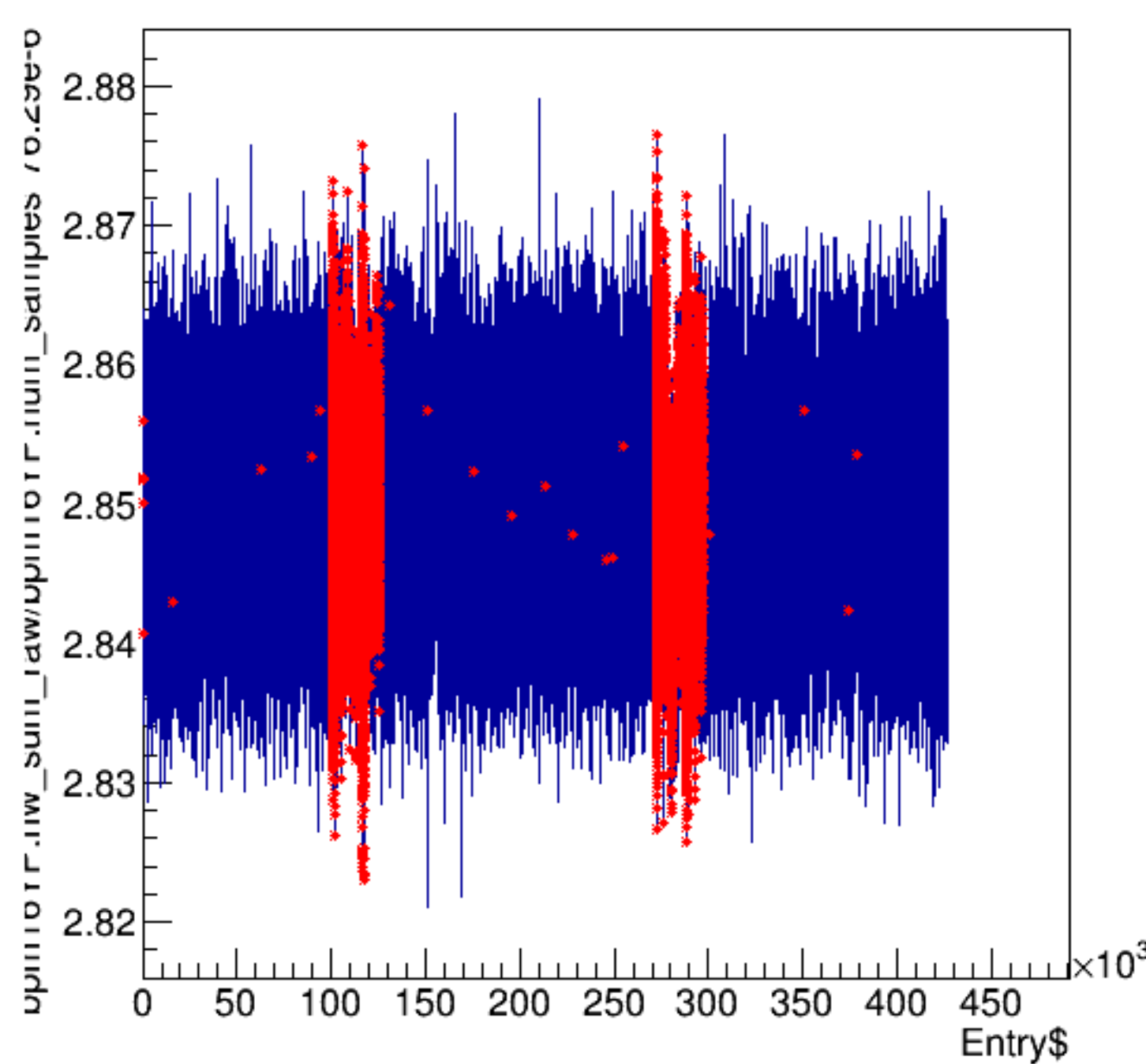
bpm16YP.hw_sum_raw/bpm16YP.num_samples*76.29e-6:Entry$
